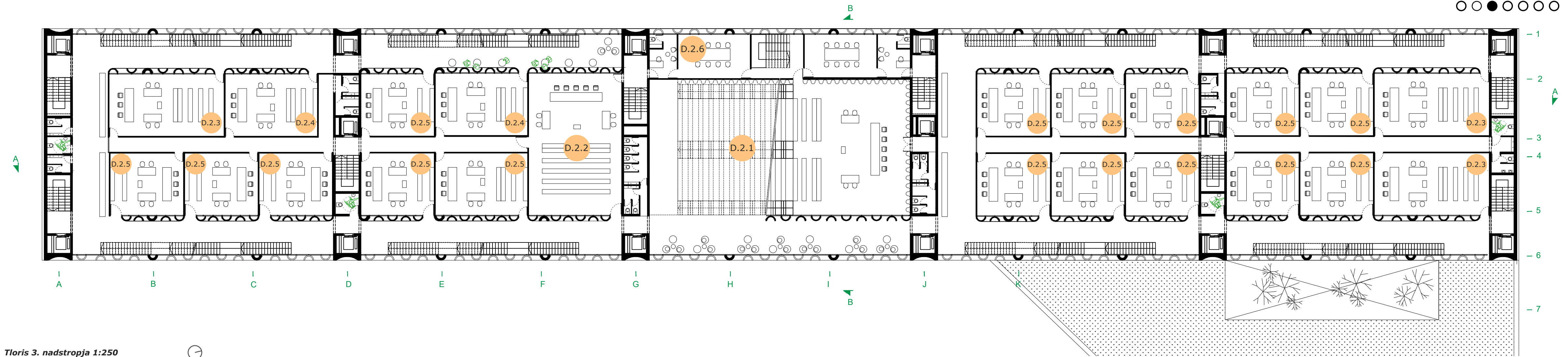
Tloris 3. nadstropja 1:250
