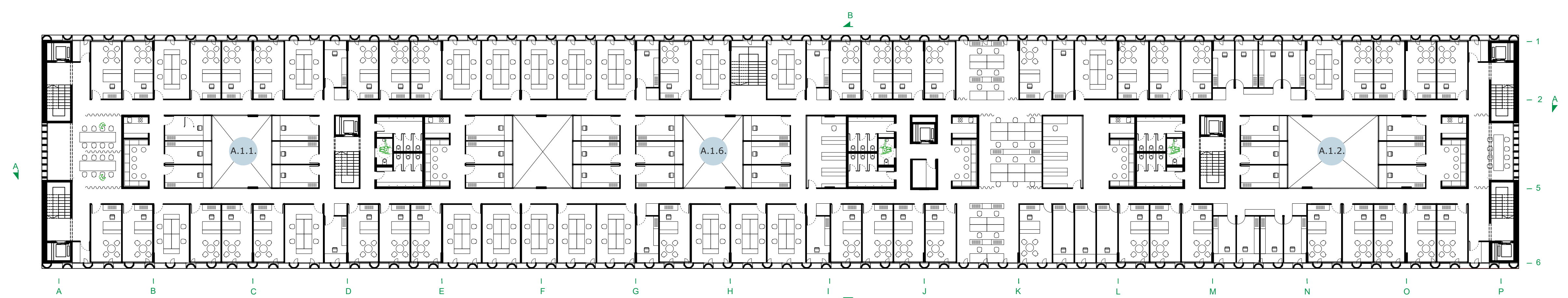
Tloris 7. nadstropja 1:250
