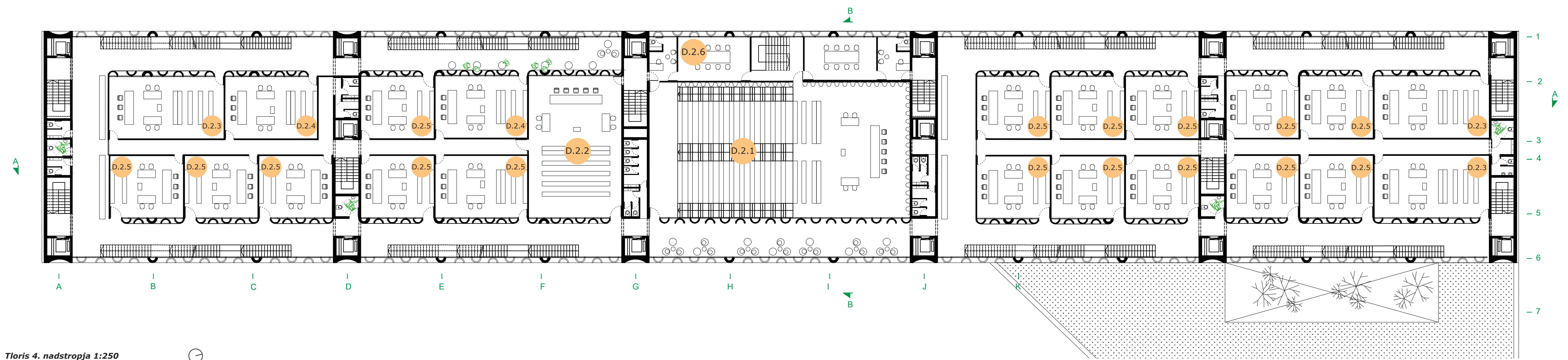
Tloris 4. nadstropja 1:250
