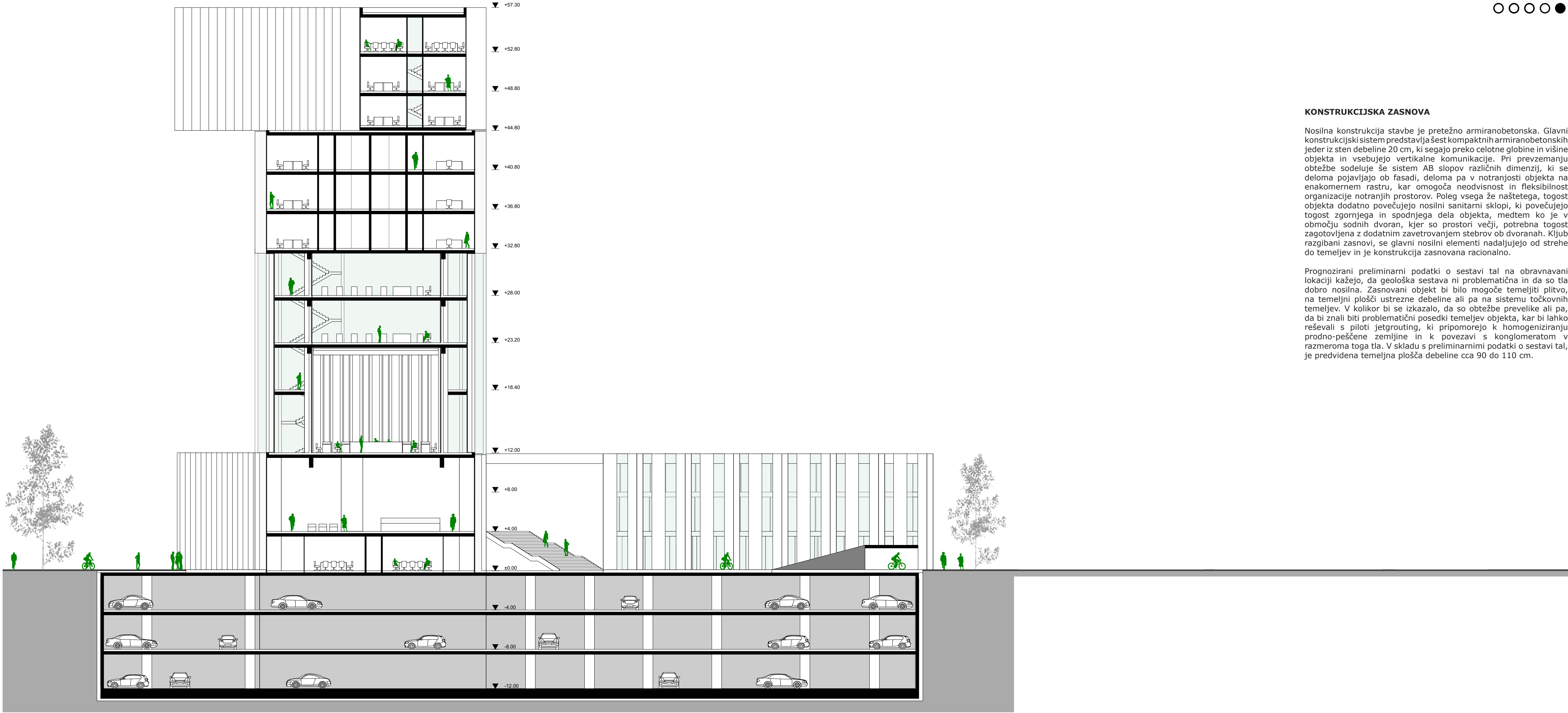
Prerez B-B 1:250
