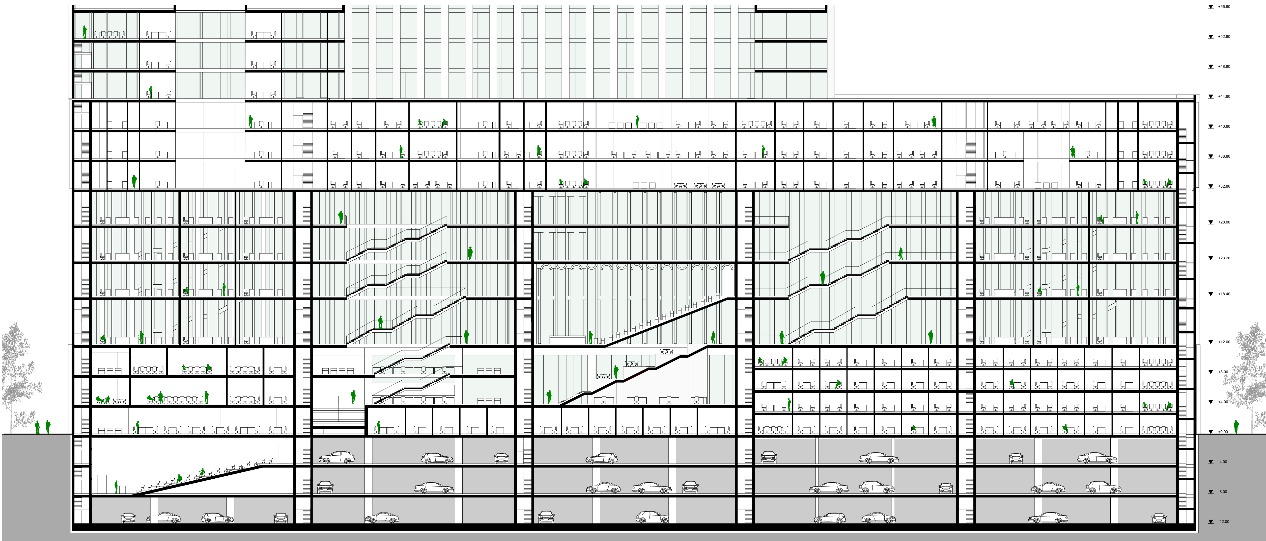
Prerez A-A 1:250
