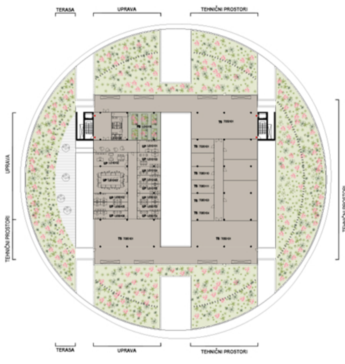
TLORIS TERASNE ETAŽE
