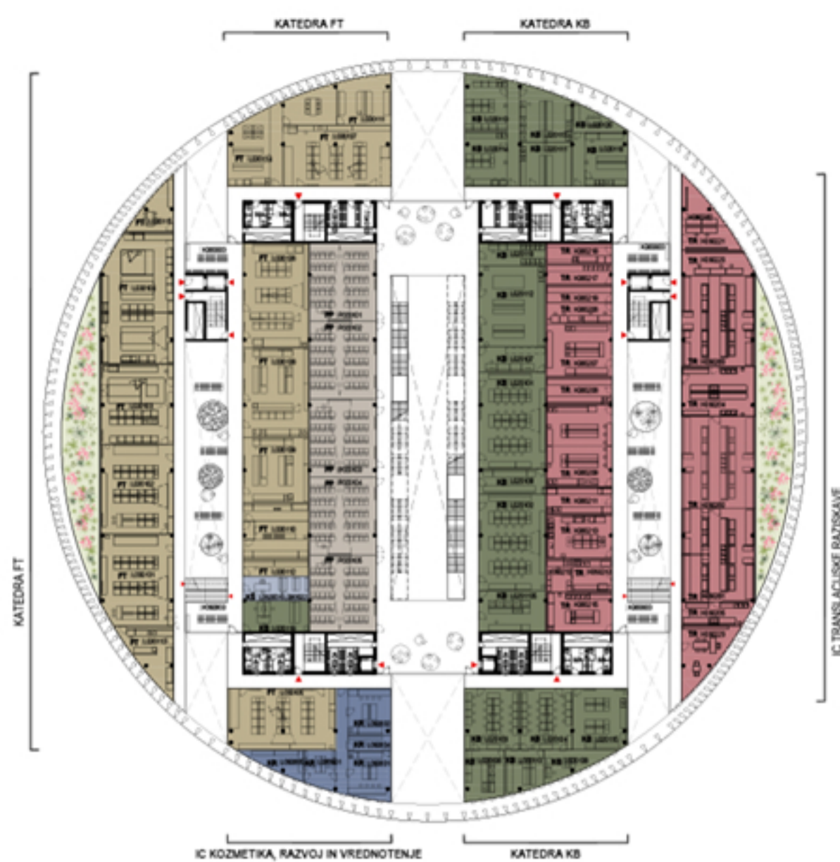
TLORIS 1. NADSTROPJA
