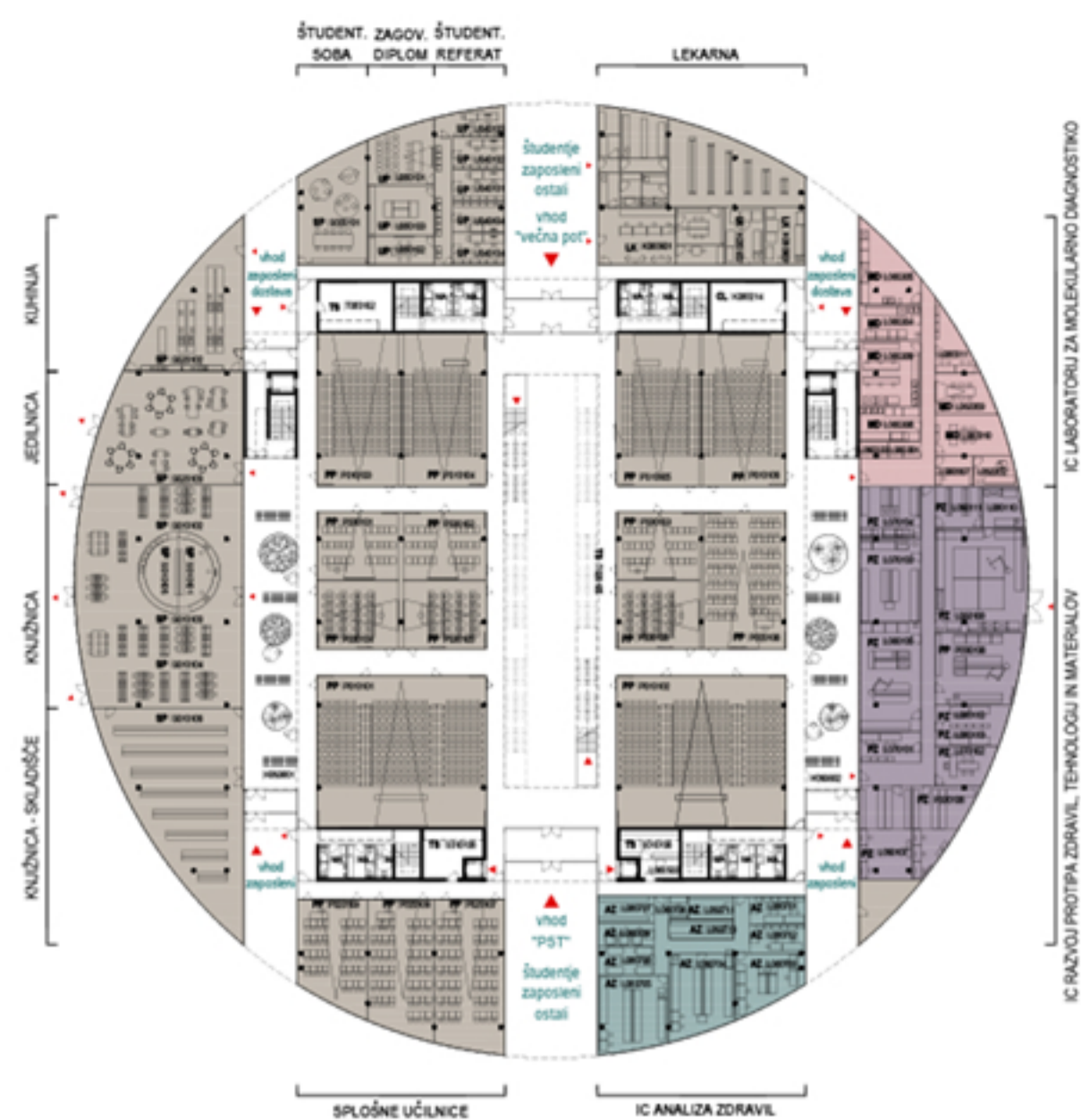
TLORIS PRITLIČJA
