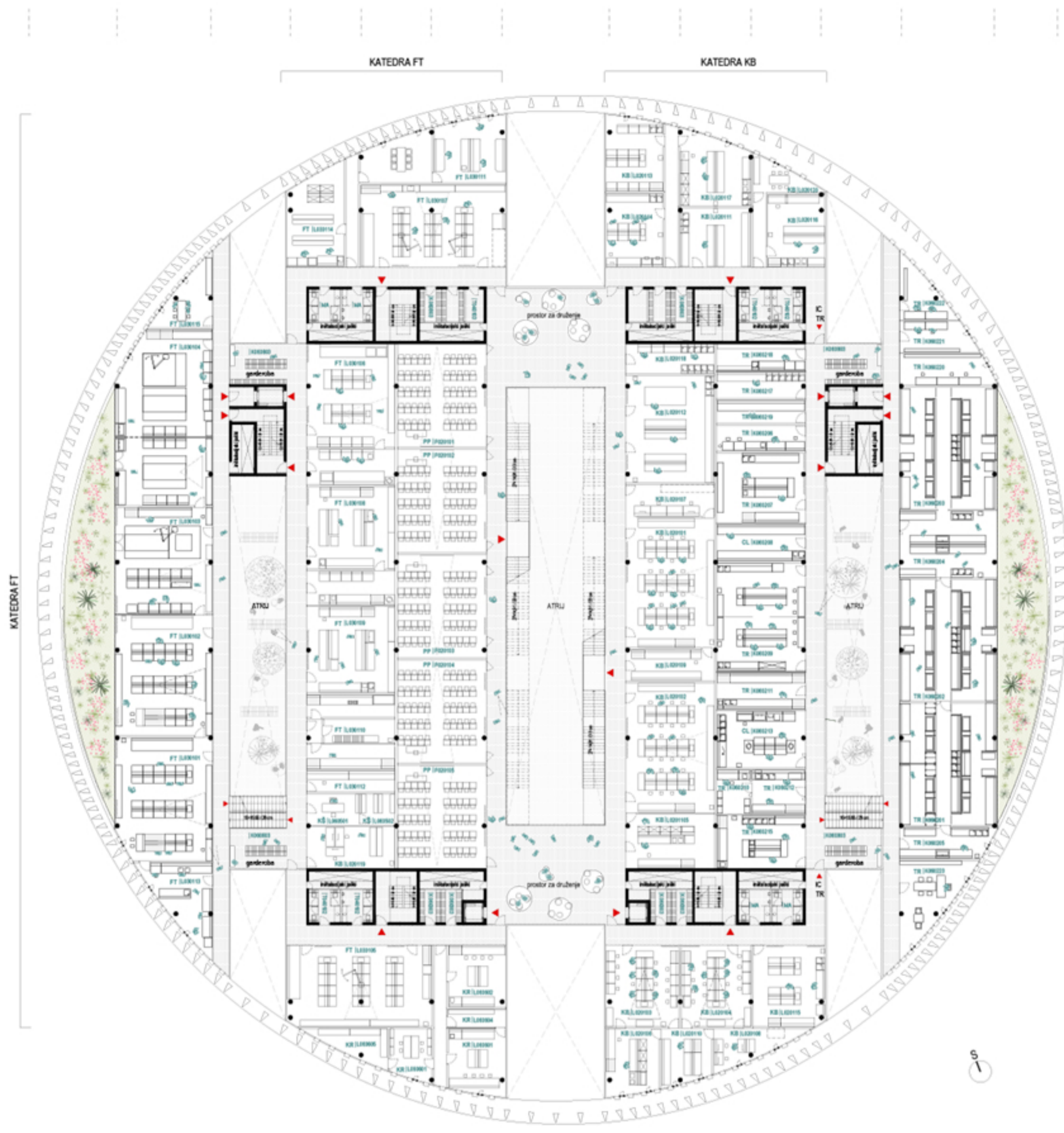
TLORIS 1. NADSTROPJA
