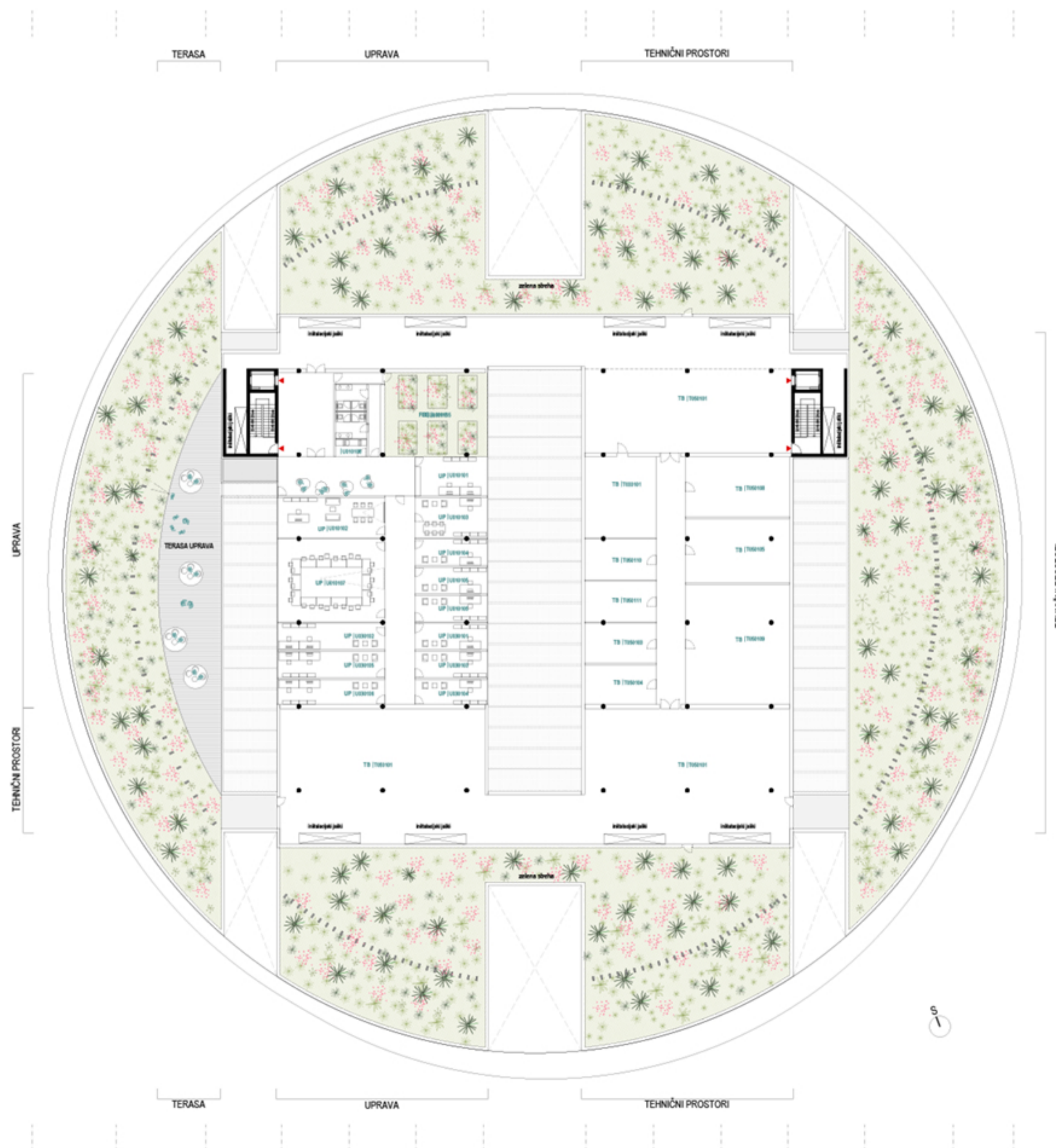
TLORIS TERASNE ETAŽE
