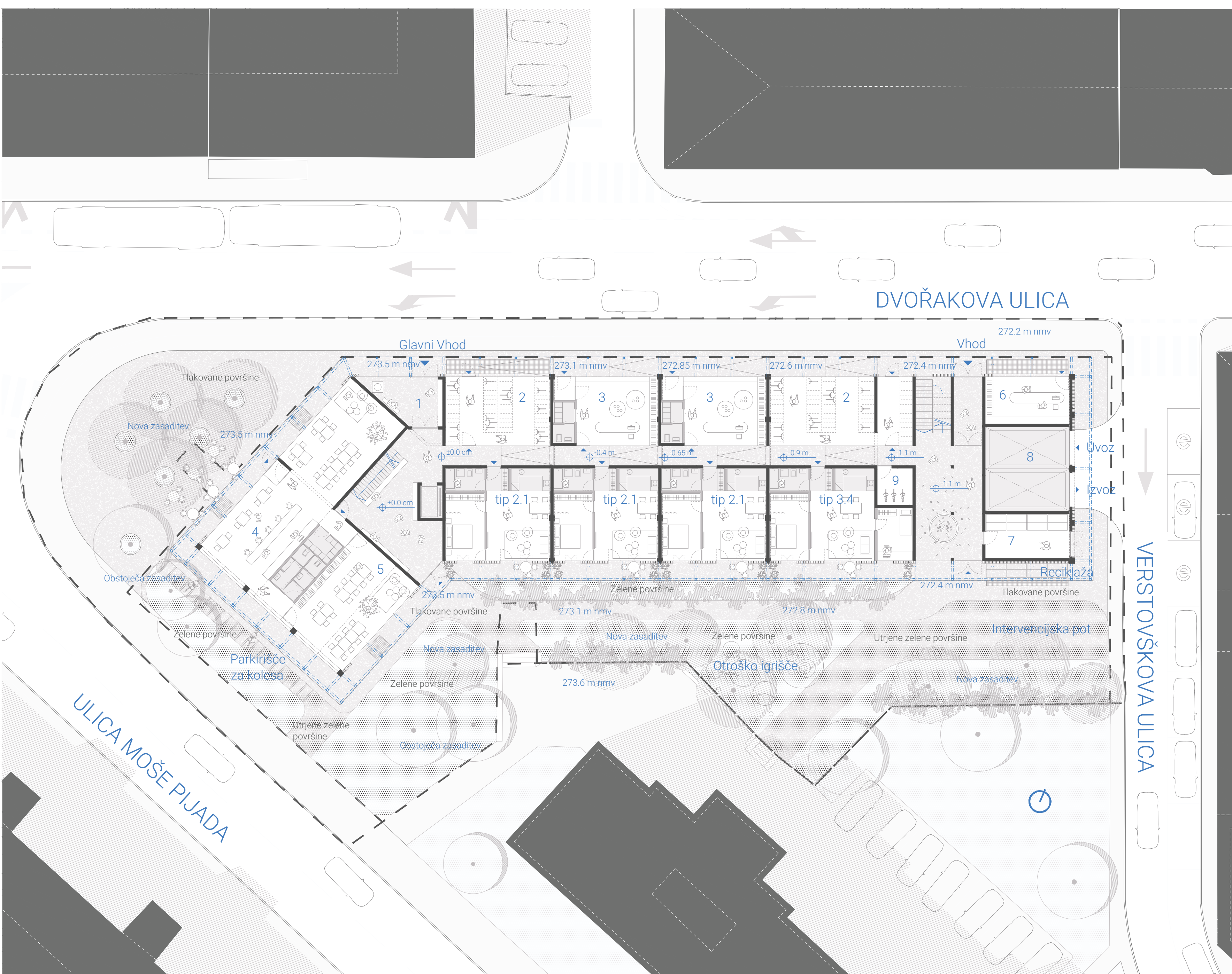
TLORIS PRITLIČJA Z ZUNANJO UREDITVIJO M 1:200
