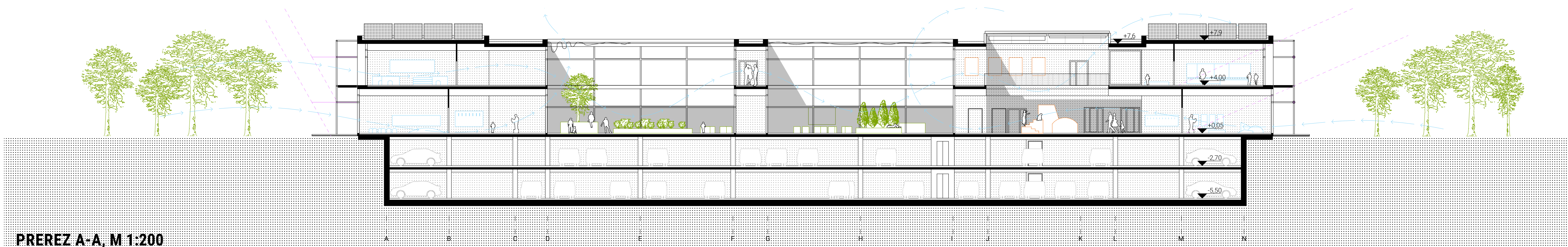
PREREZ A-A, M 1:200
