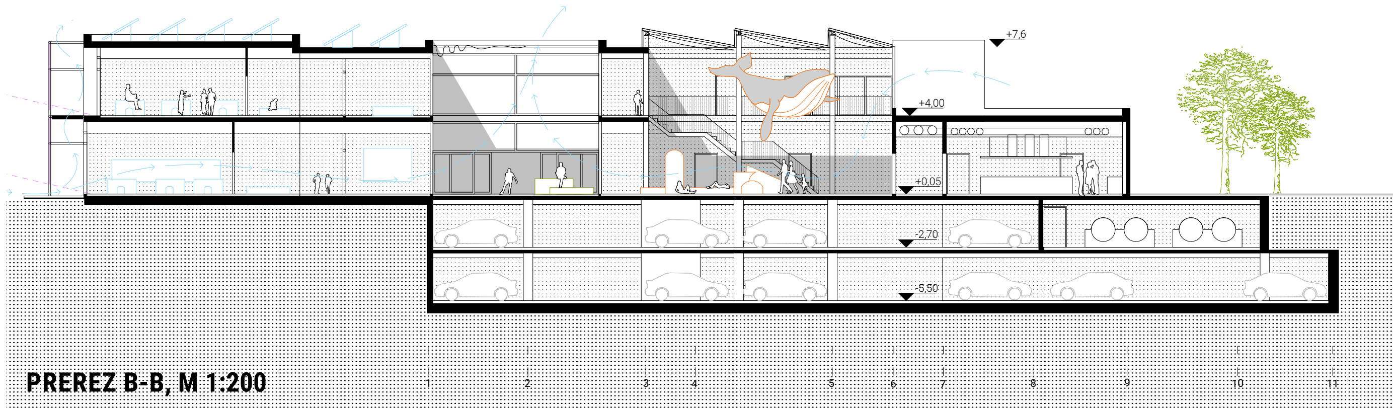
JUGOVZHODNA FASADA, M 1:200
