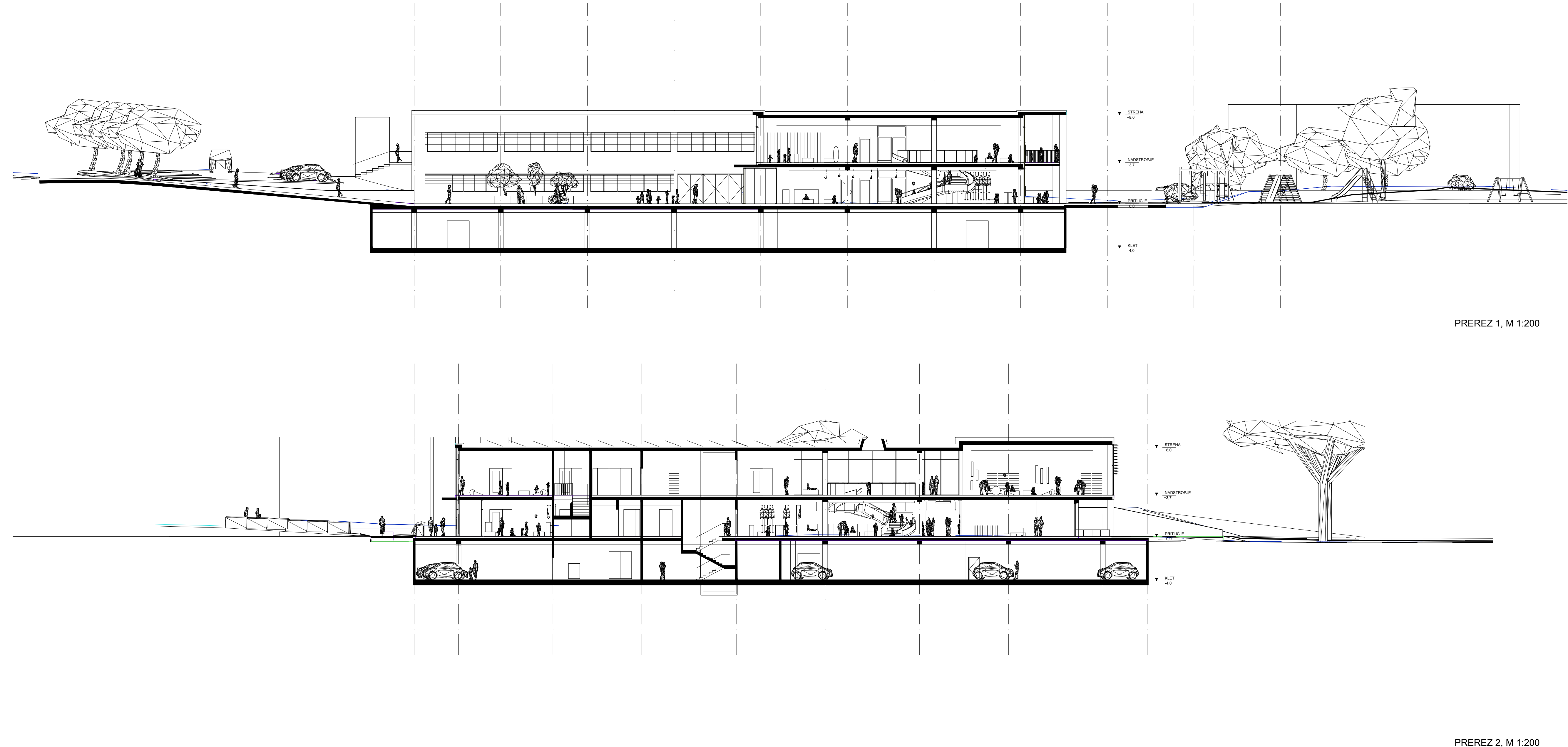
PREREZ 2, M 1:200
