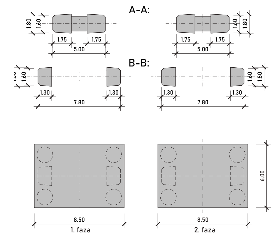
PREČNI PREREZI PODPOR IN OBEŠENE BRVI
