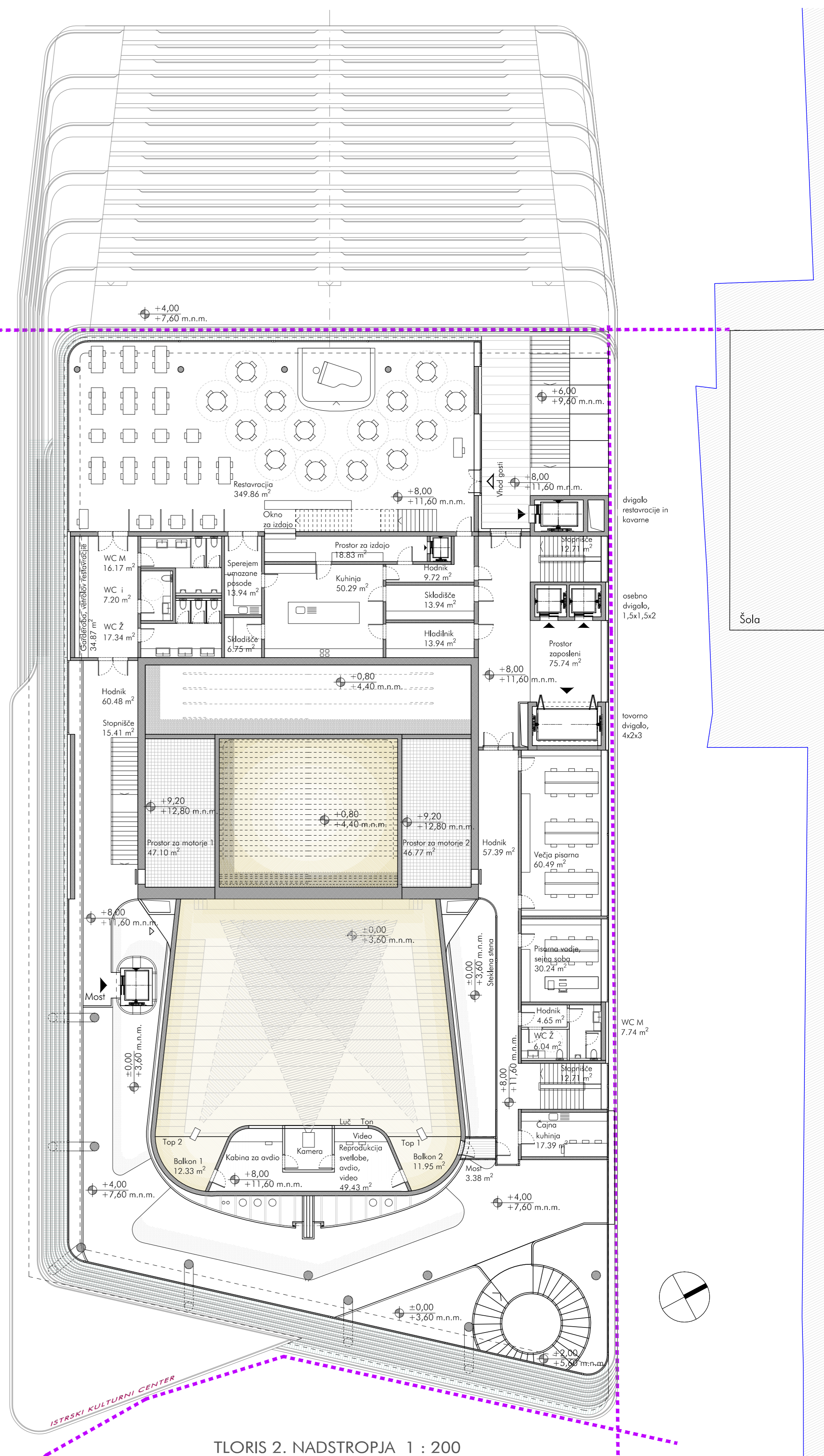
TLORIS 2. NADSTROPJA 1 : 200
