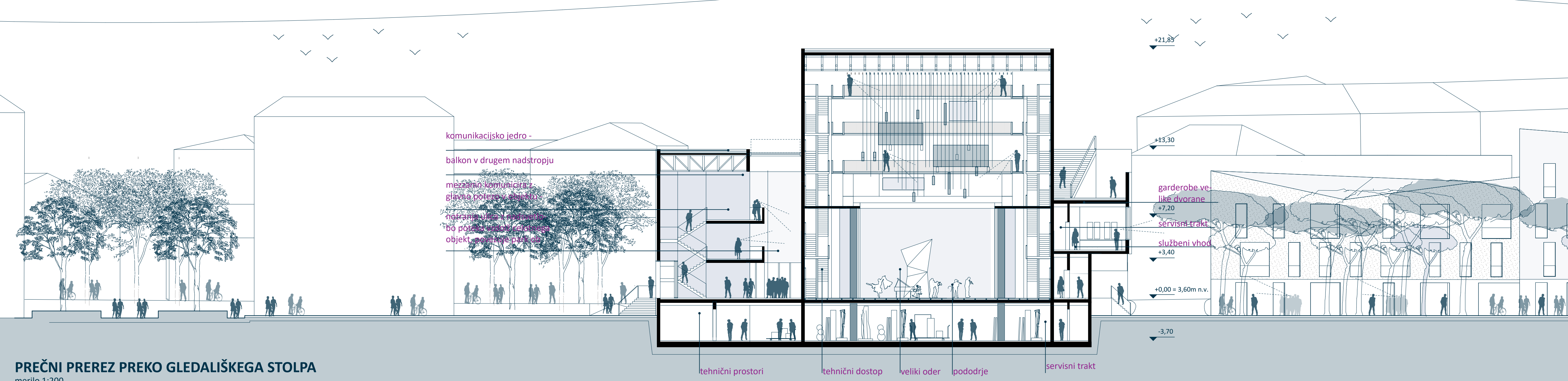
VZDOLŽNI PREREZ PREKO DVORANE merilo 1:200
