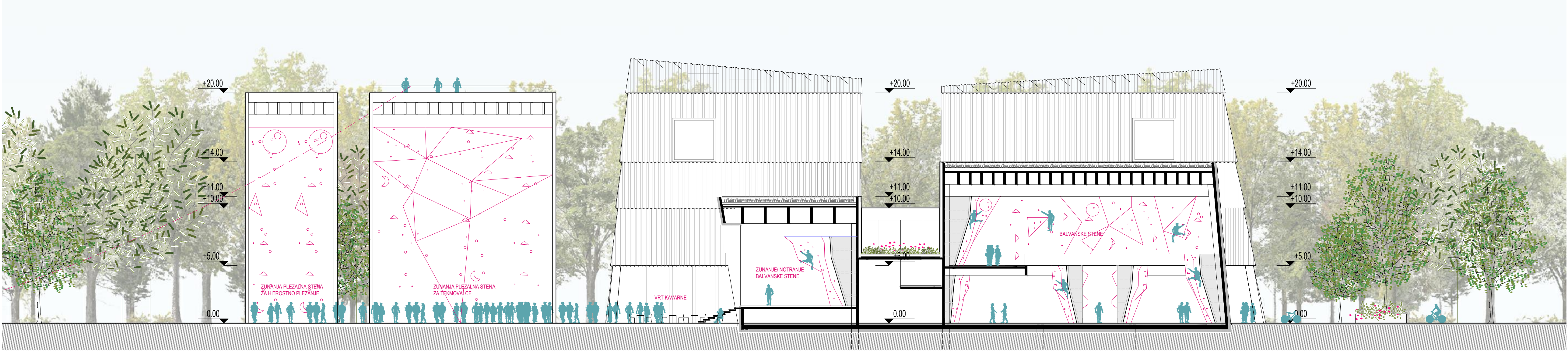
PREČNI PREREZ B-B, M 1:200
