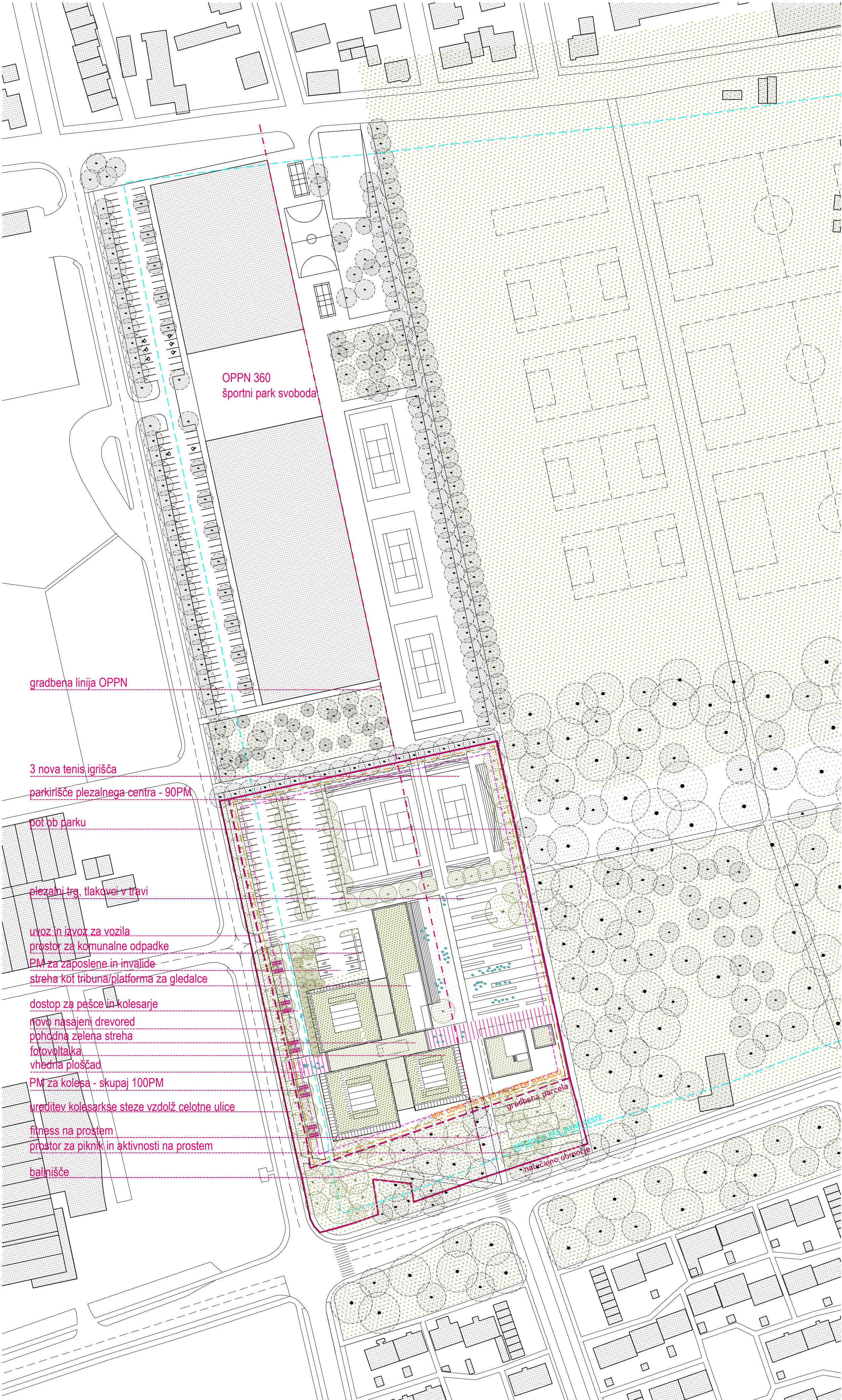
UREDITVENA SITUACIJA NATEČAJNEGA IN RAZŠIRJENEGA OBMOČJA S PRIKAZOM TLORISA STREH, M 1:1000
