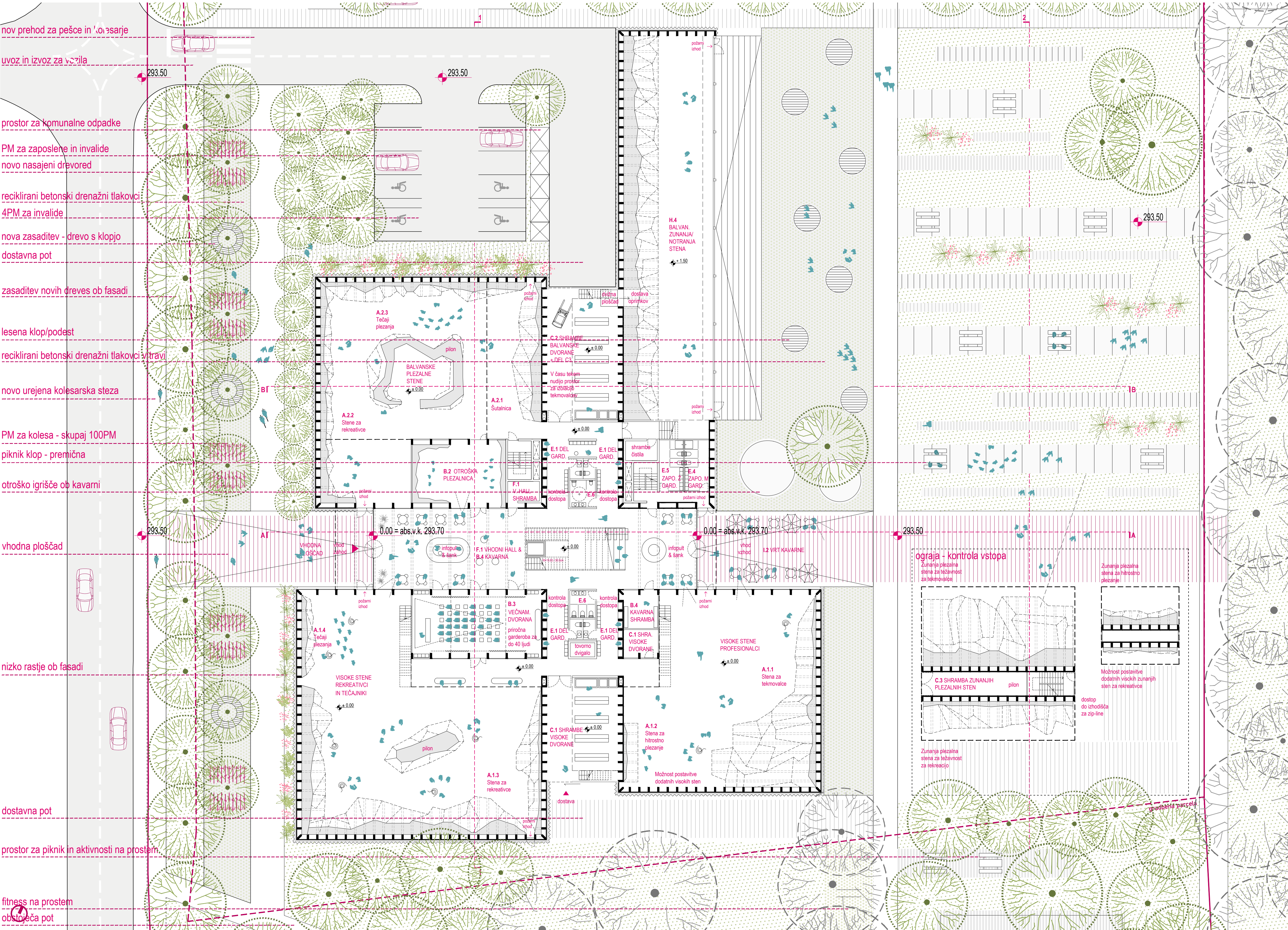
TLORIS PRITLIČJA OBJEKTA Z ZUNANJO UREDITVIJO, M 1:200
