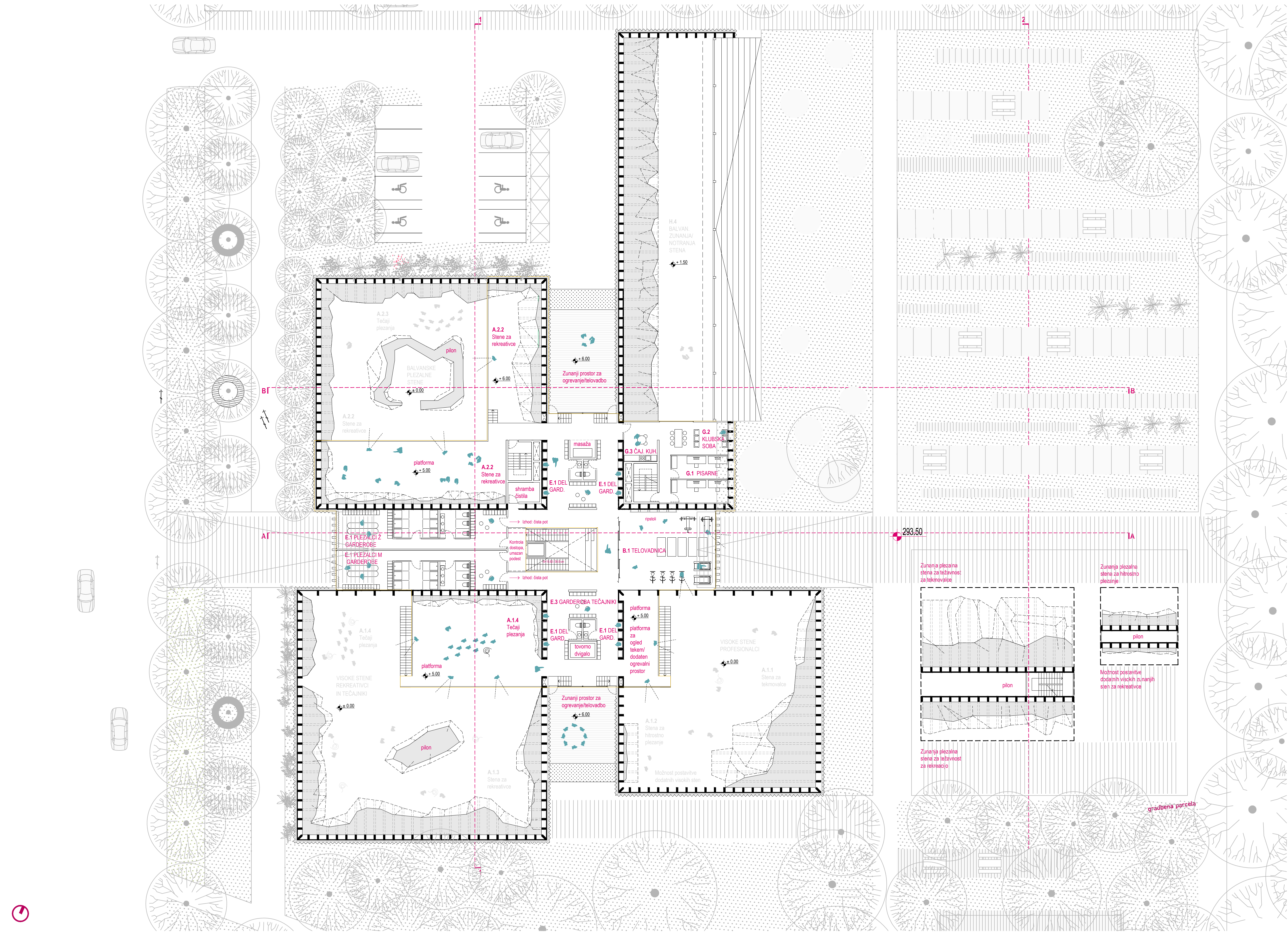
TLORIS NADSTROPJA, M 1:200
