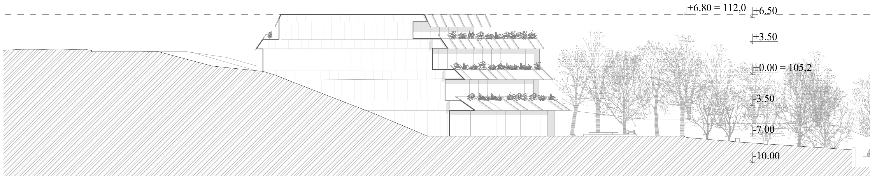
Vzhodna fasada merilo 1:250
