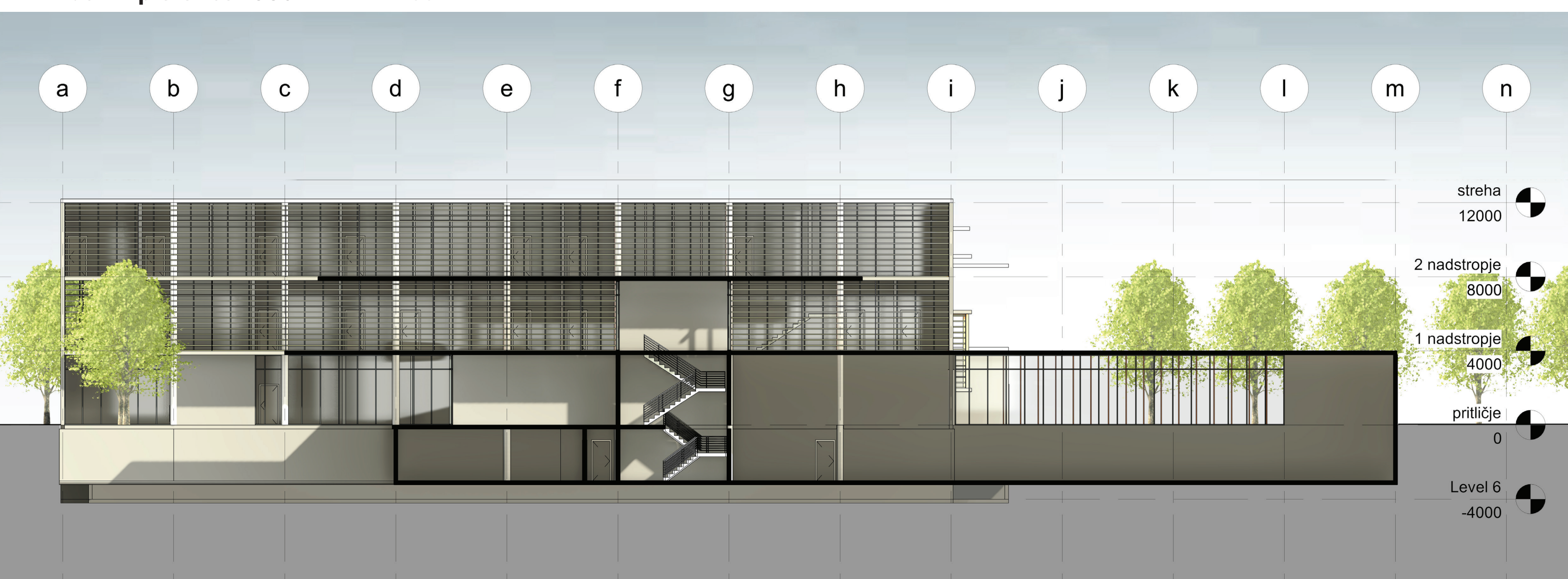
vzdolžni prerez čez CSGM | 1:200
