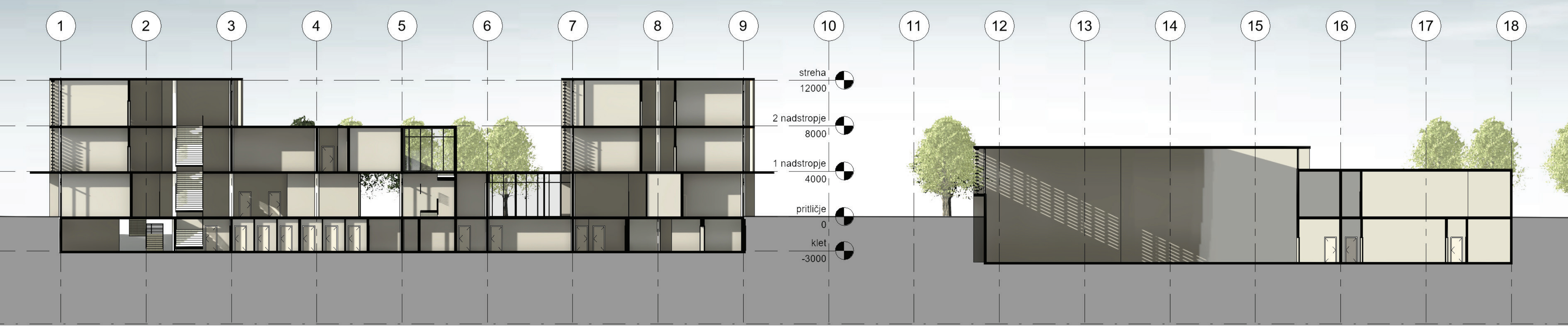
prečni prerez skozi CSGM in športno dvorano | 1:200
