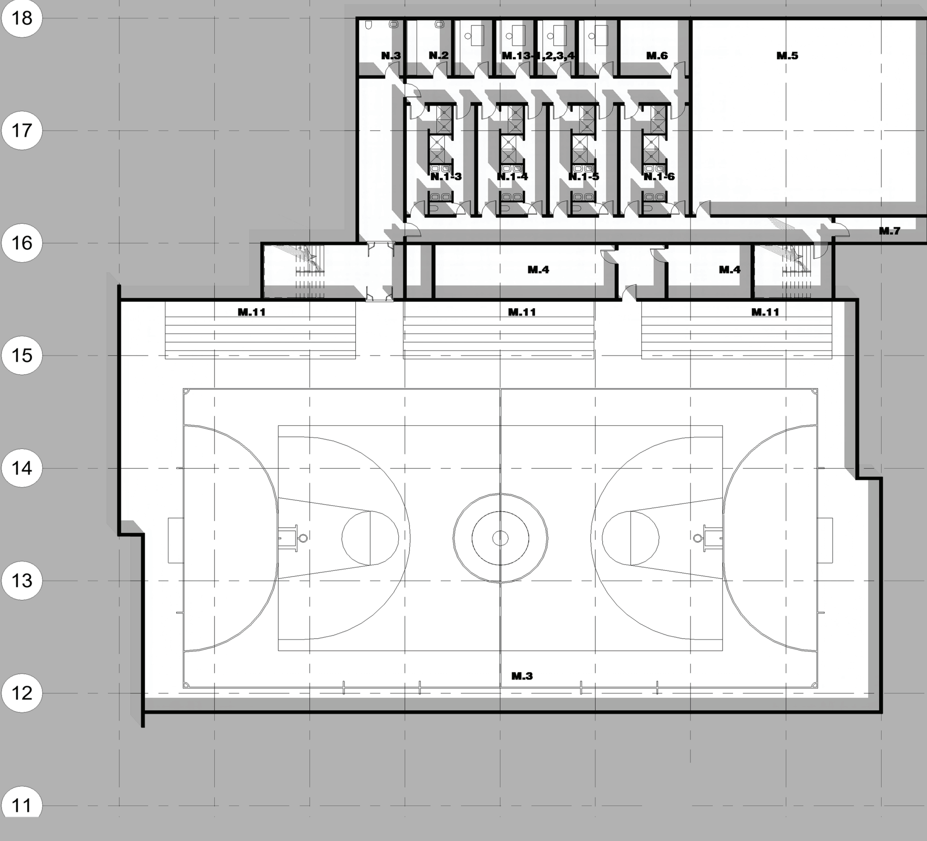
tloris kleti športne dvorane in pripadajočih prostorov | 1:200
