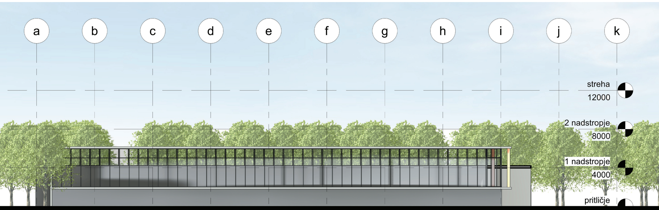
južna fasada dvorane | 1:200
