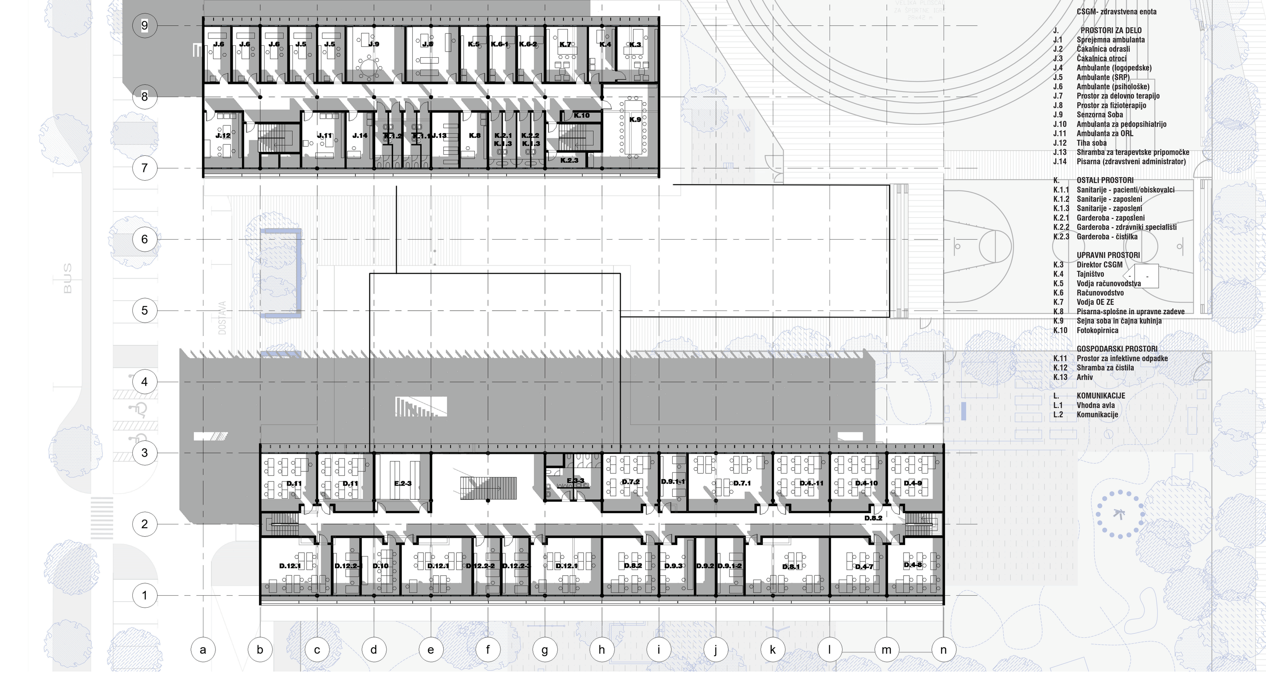
tloris 2. nadstropja | 1:200
