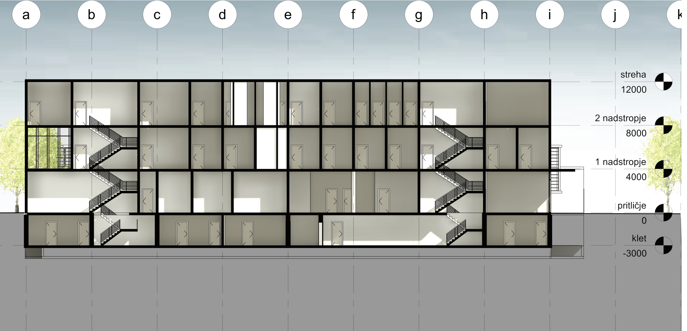
vzdolžni prerez čez CSGM | 1:200
