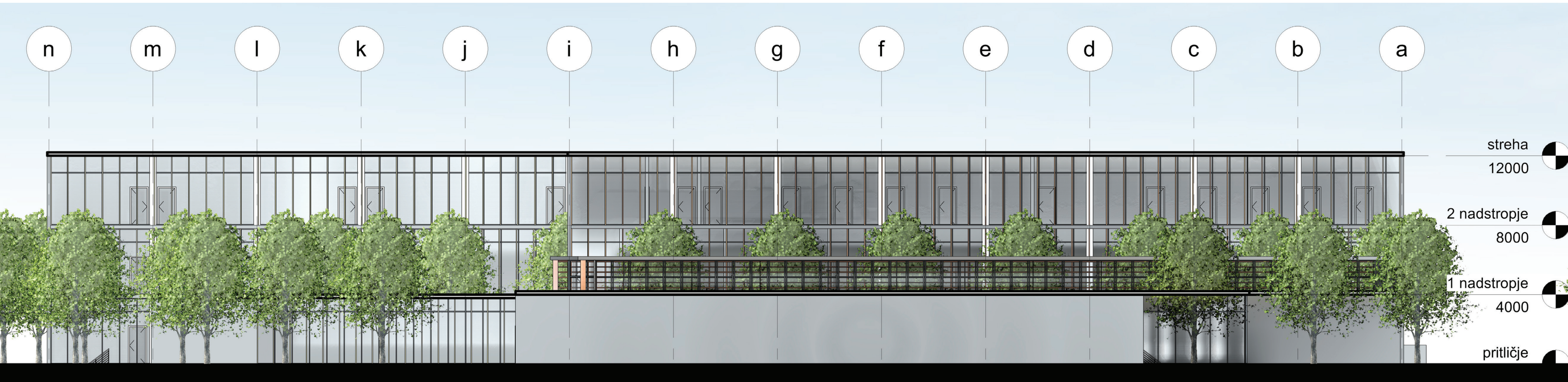
severna fasada dvorane | 1:200
