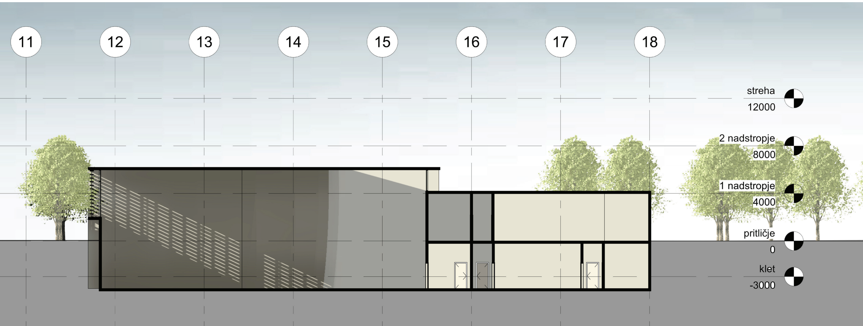
vzdolžni prerez čez športno dvorano | 1:200
