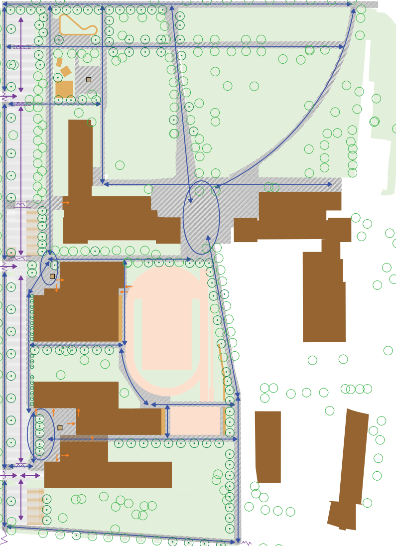
shema povezav z zelenitvijo
