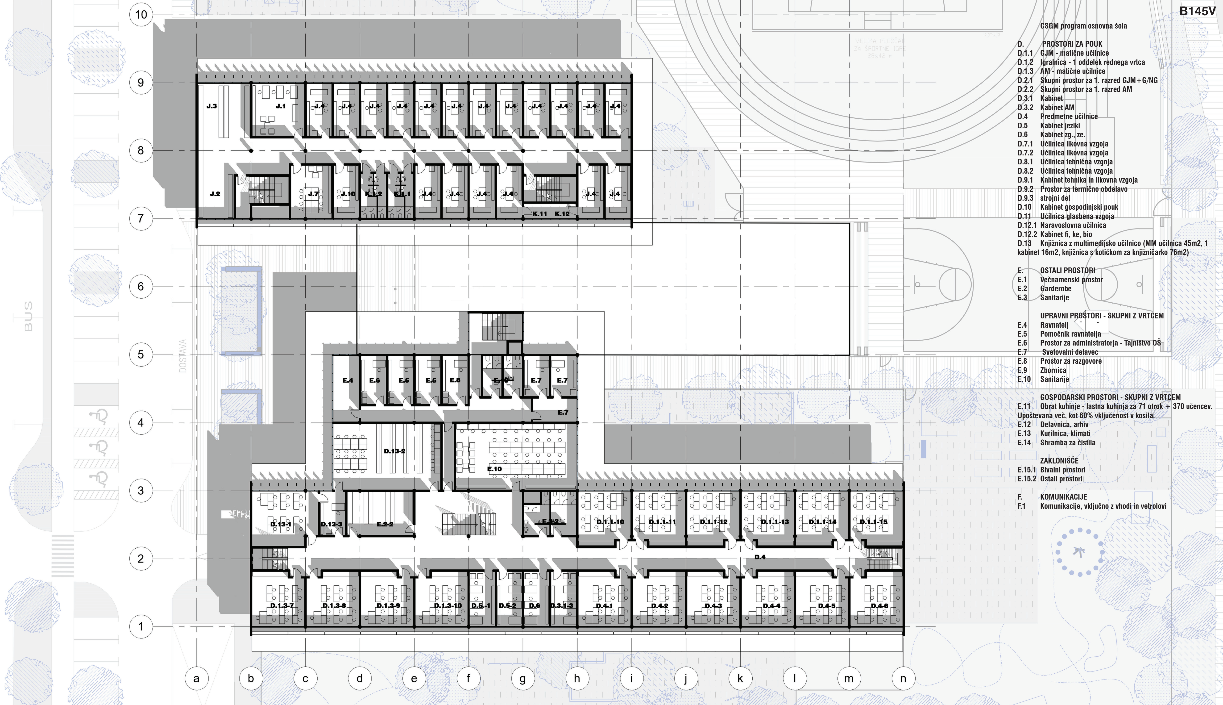
tloris 1. nadstropja | 1:200
