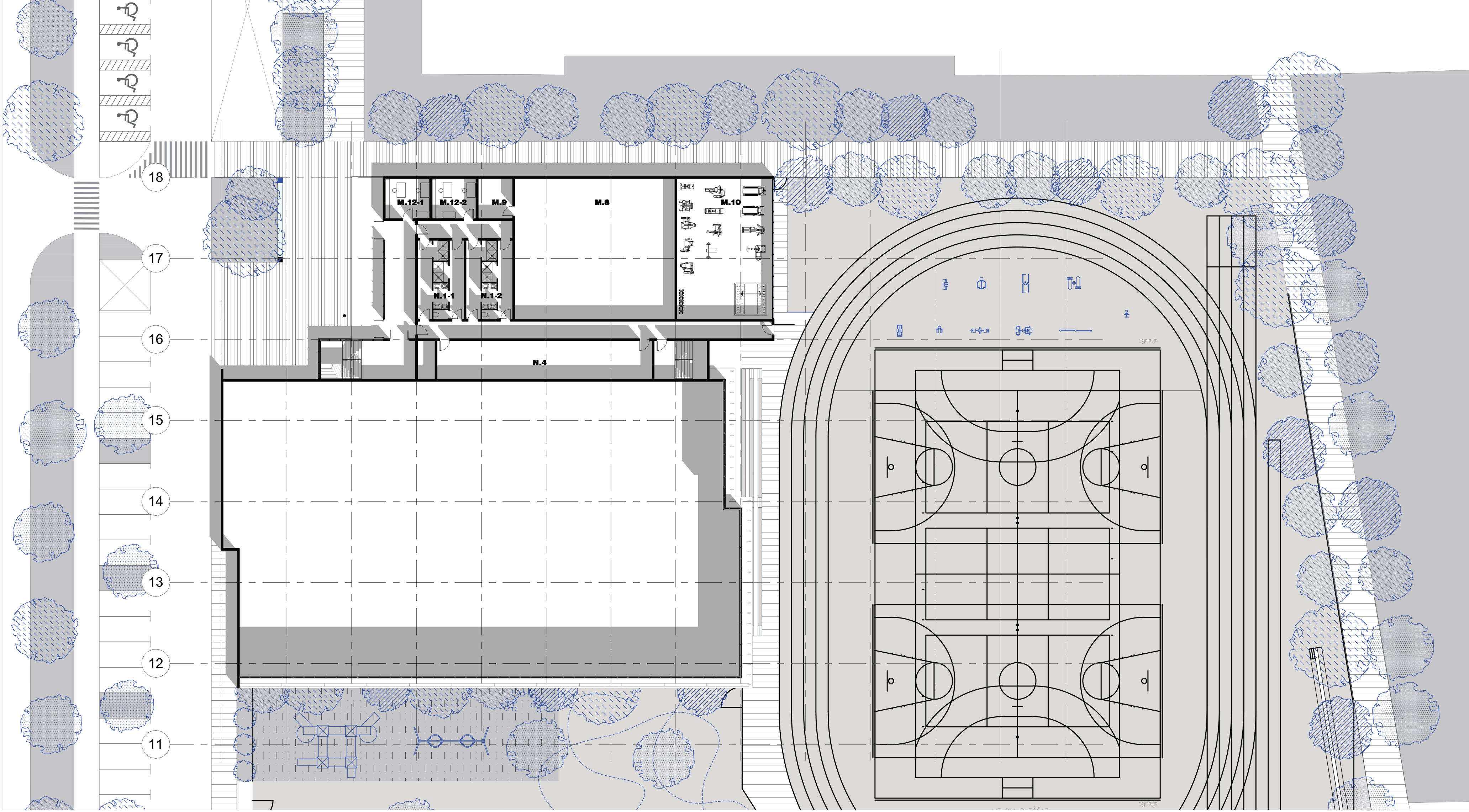
tloris pritličja športne dvorane in pripadajočih prostorov | 1:200
