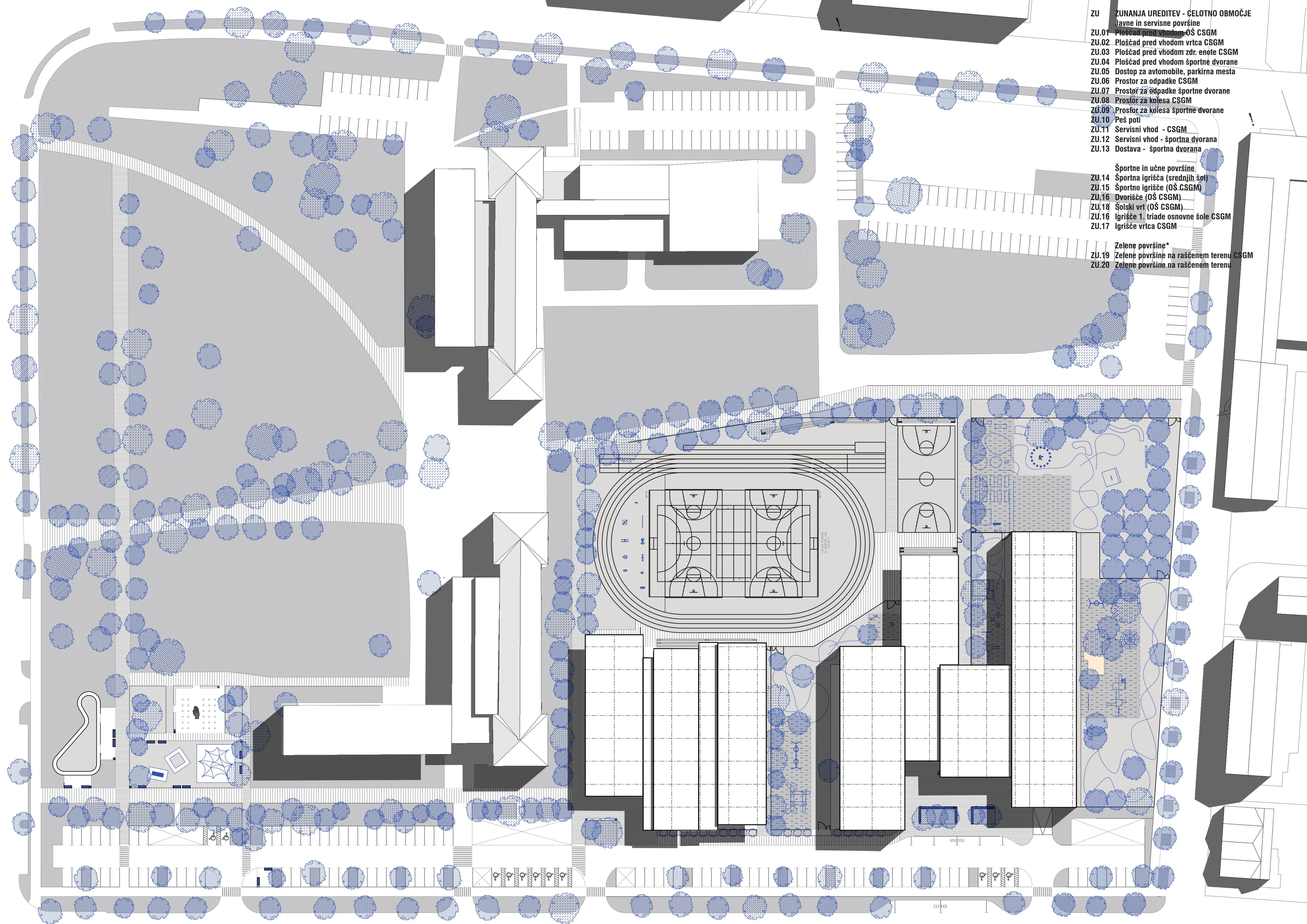
UREDITVENA SITUACIJA Z ZUNANJO IN PROMETNO UREDITVIJO / M 1:500
