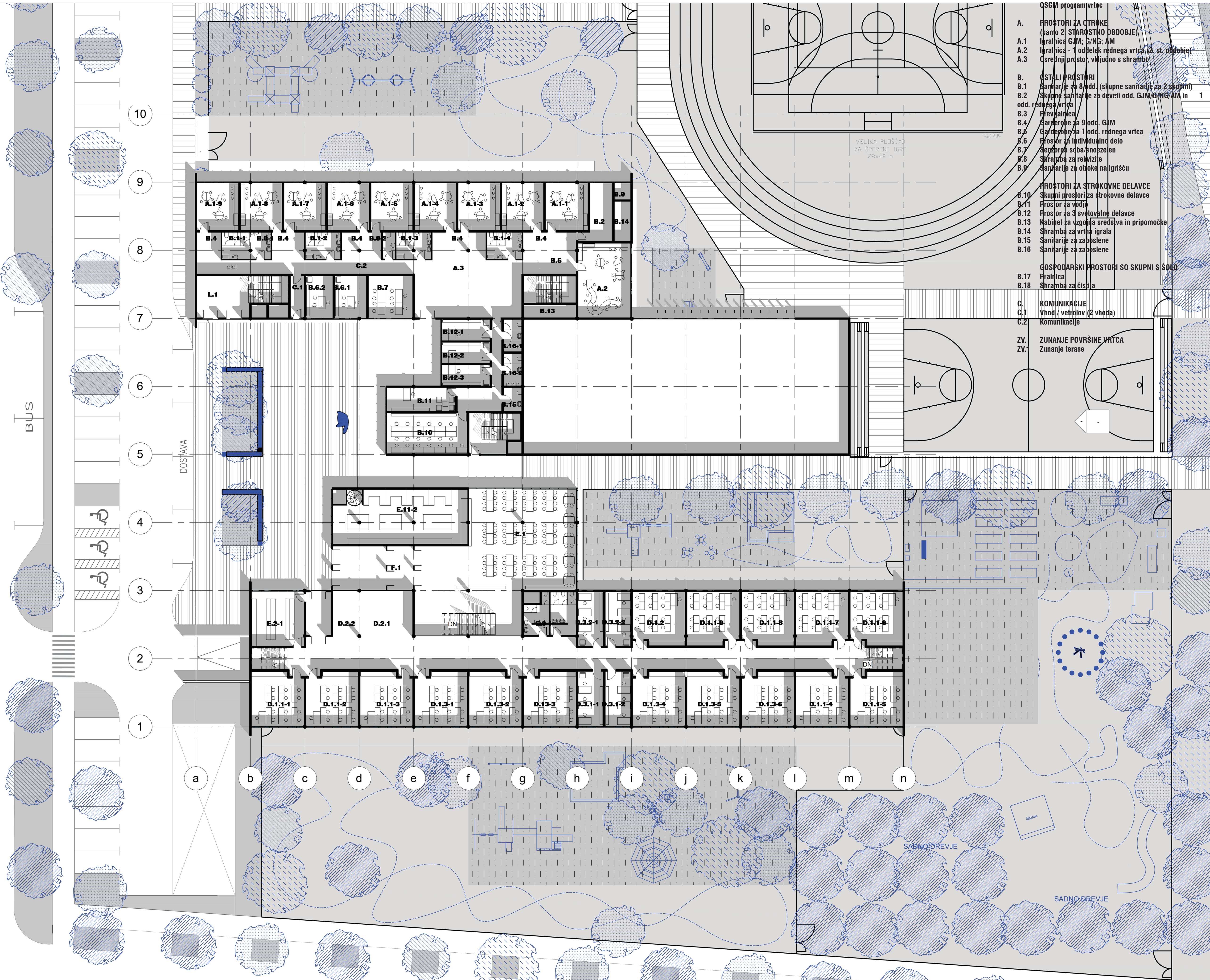
tloris prtiličja | 1:200
