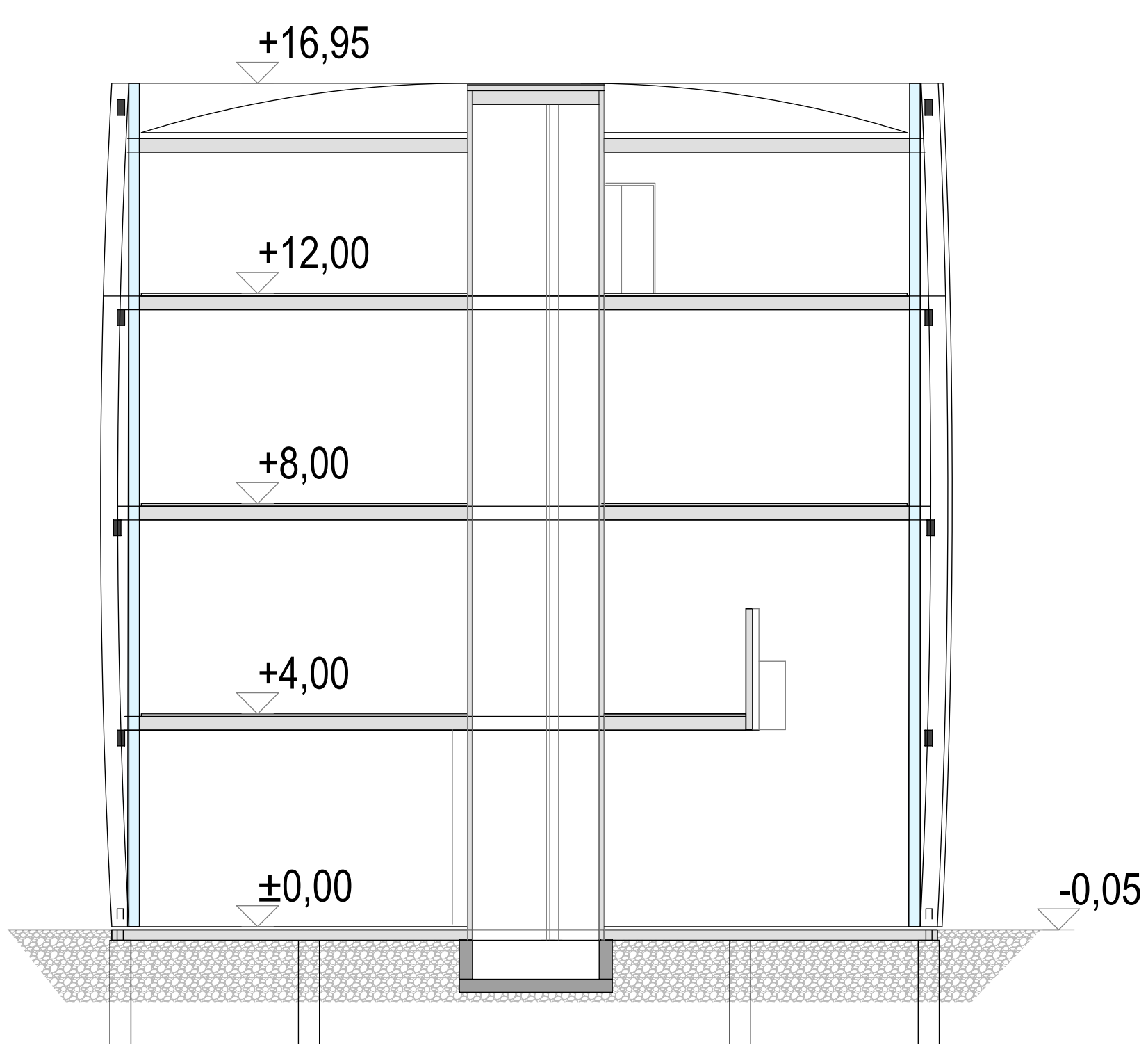
prerez 2 - 2
