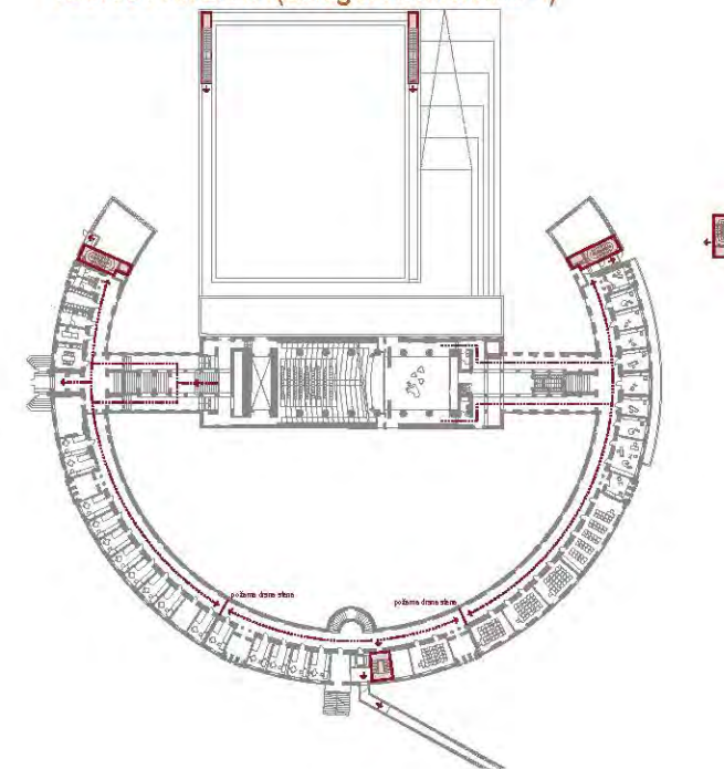
Shema požarne varnosti: TLORIS PRITLIČJA (Baragovo semenišče -1)
