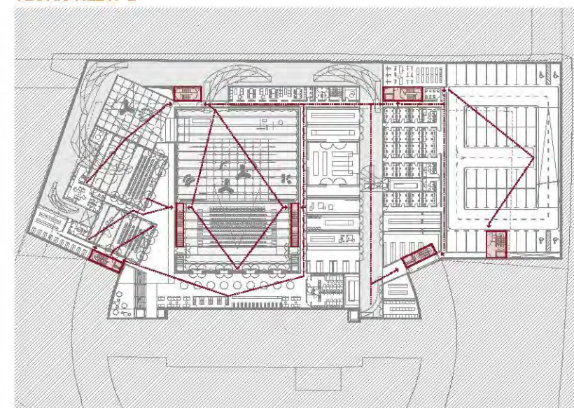
Shema požarne varnosti: TLORIS KLETI -2
