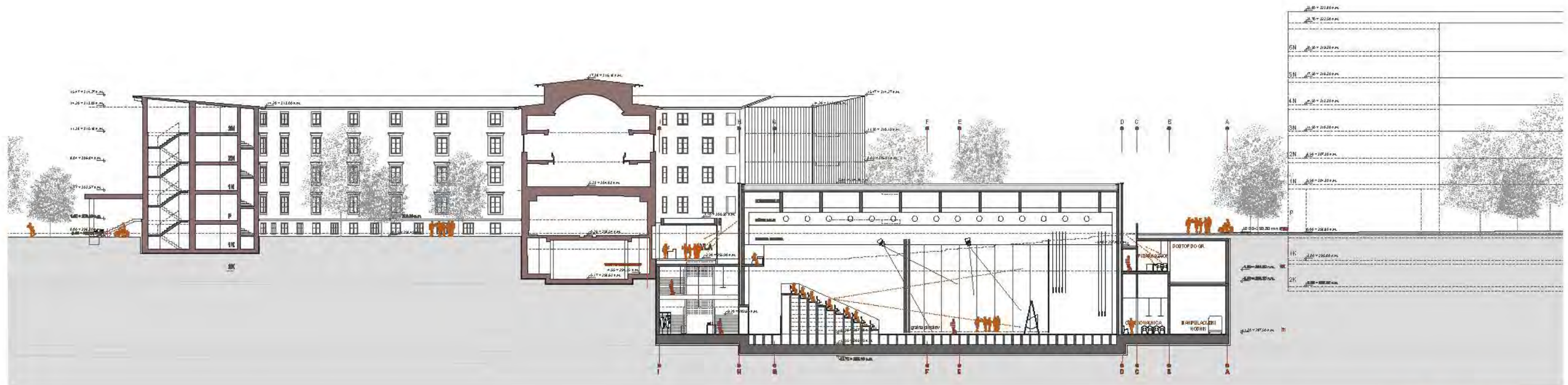
PREČNI PREREZ A-A M_1:500
