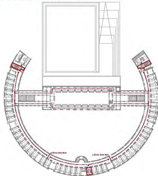
Shema požarne varnosti: TLORIS 2. IN 3. NADSTROPJA
