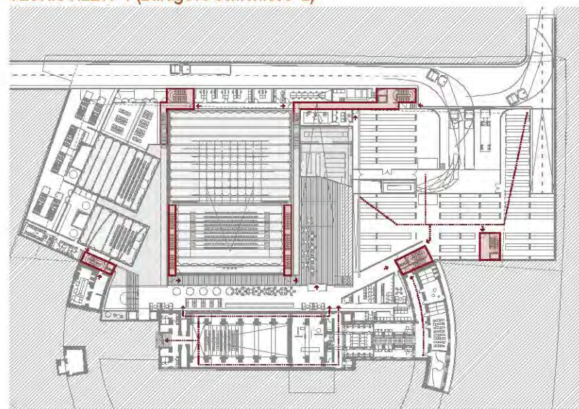
Shema požarne varnosti: TLORIS KLETI -1 (Baragovo semenišče -2)
