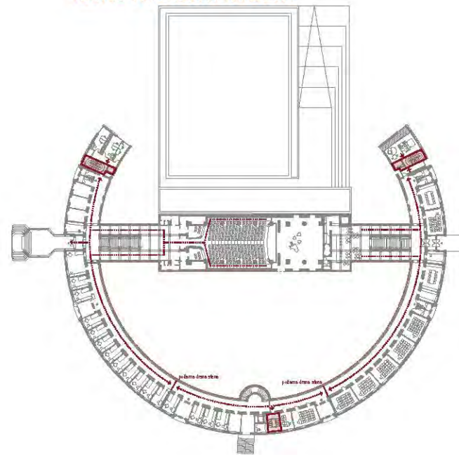
Shema požarne varnosti: TLORIS VIŠKEGA PRITLIČJA
