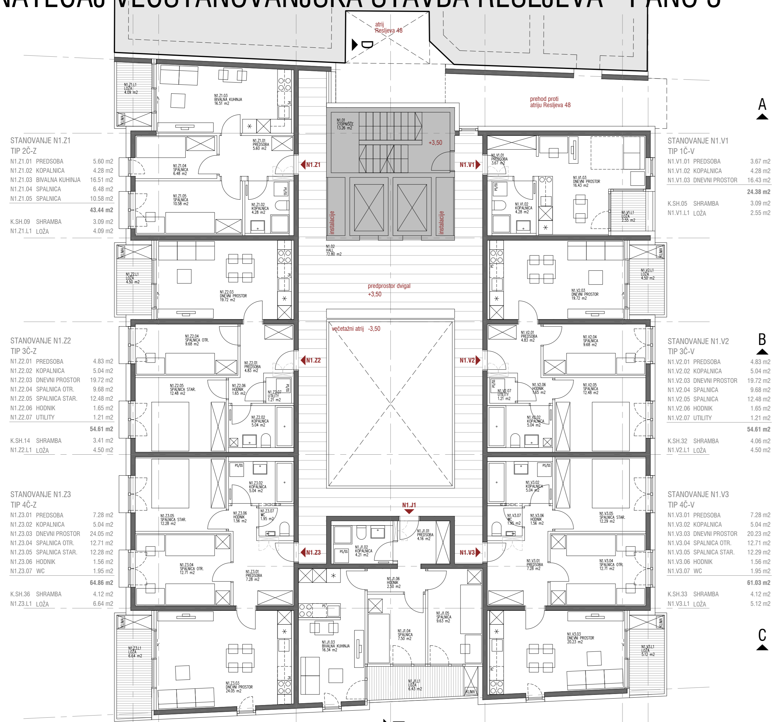
1. NADSTROPJE M 1:100
