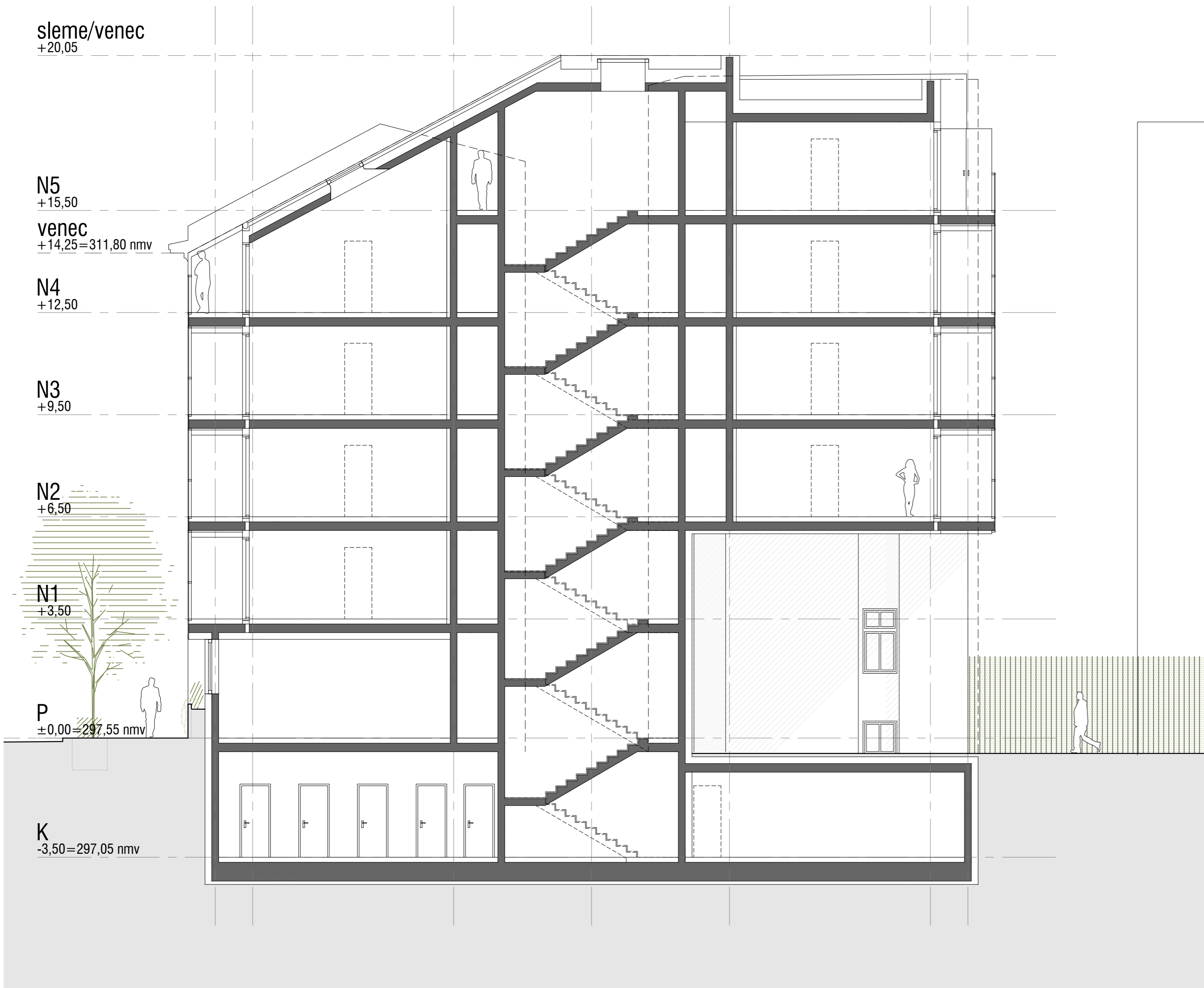
PREREZ A-A M 1:100
