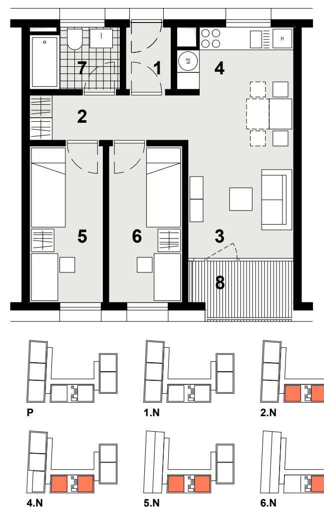
katalog stanovanj M_1:100
