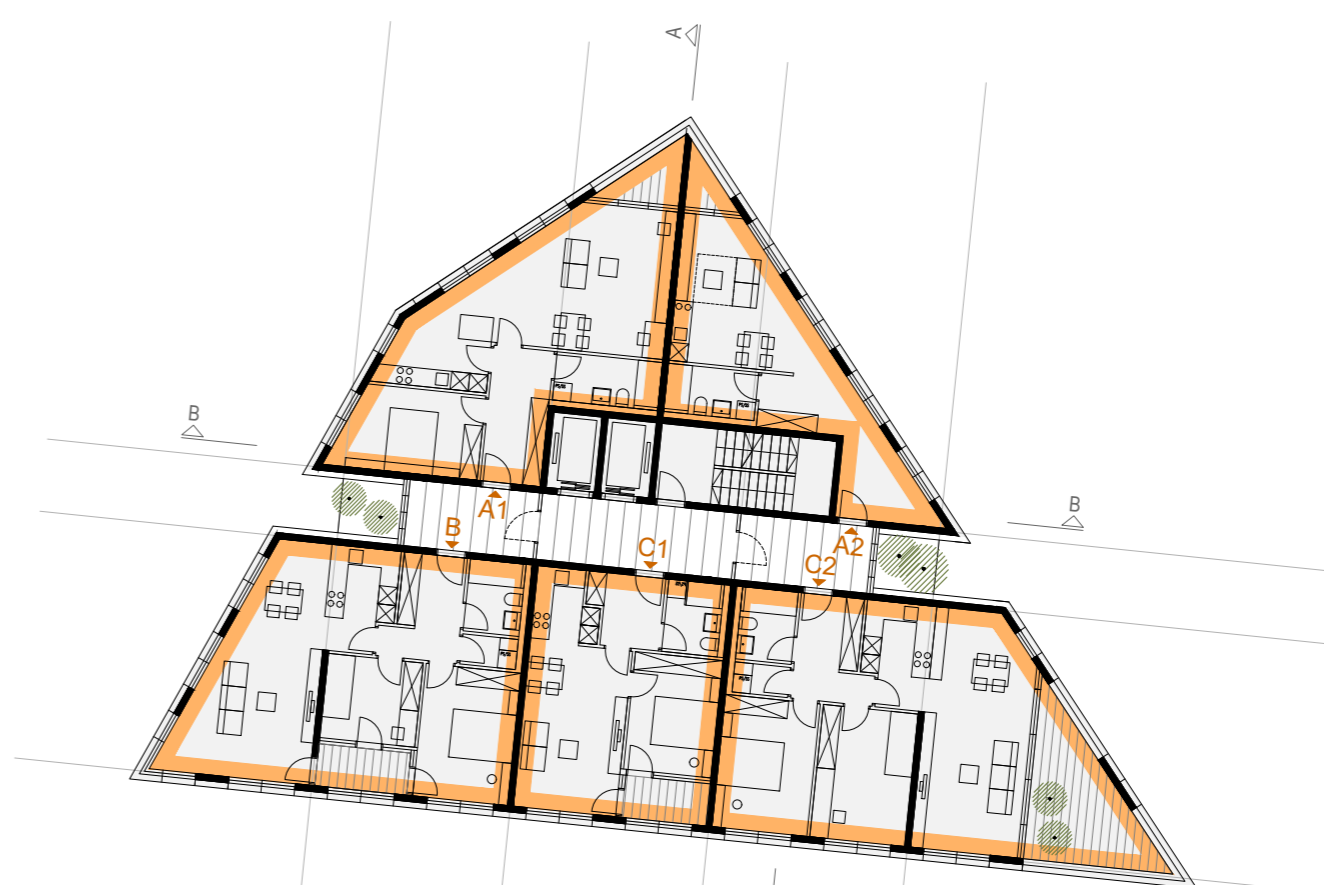
3.-10. NADSTROPJE M 1:250
