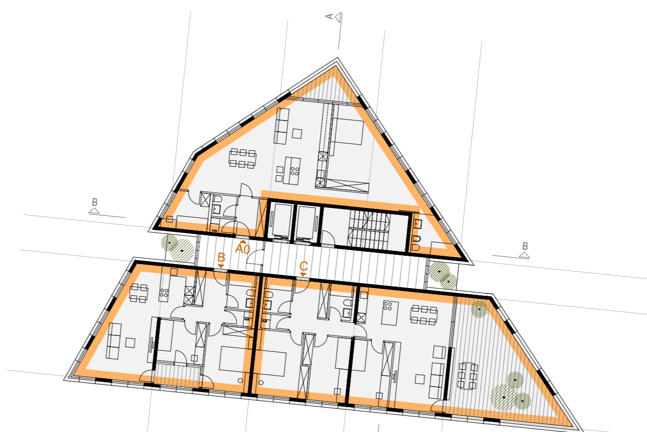
13.-14. NADSTROPJE M 1:250
