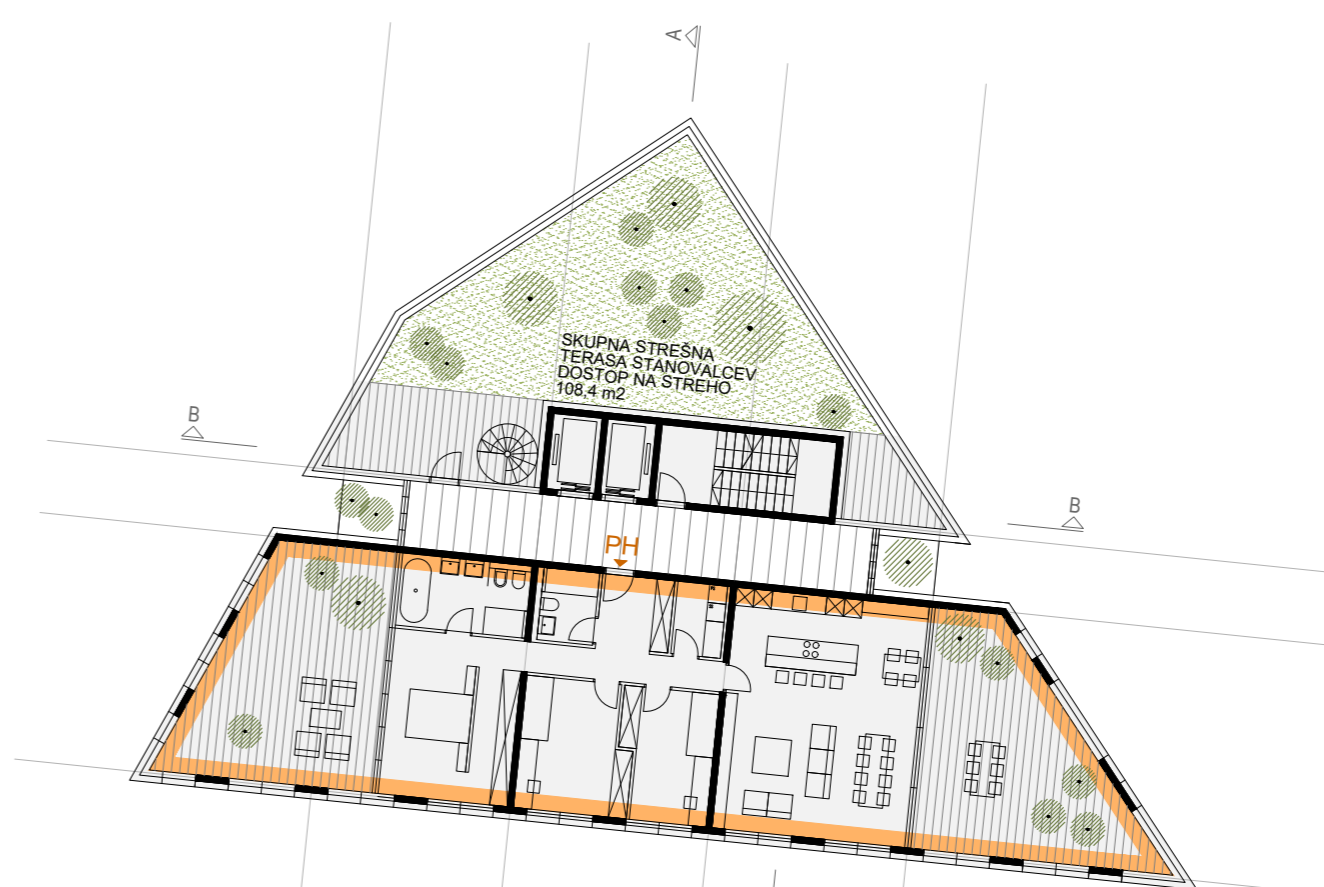
15. NADSTROPJE M 1:250
