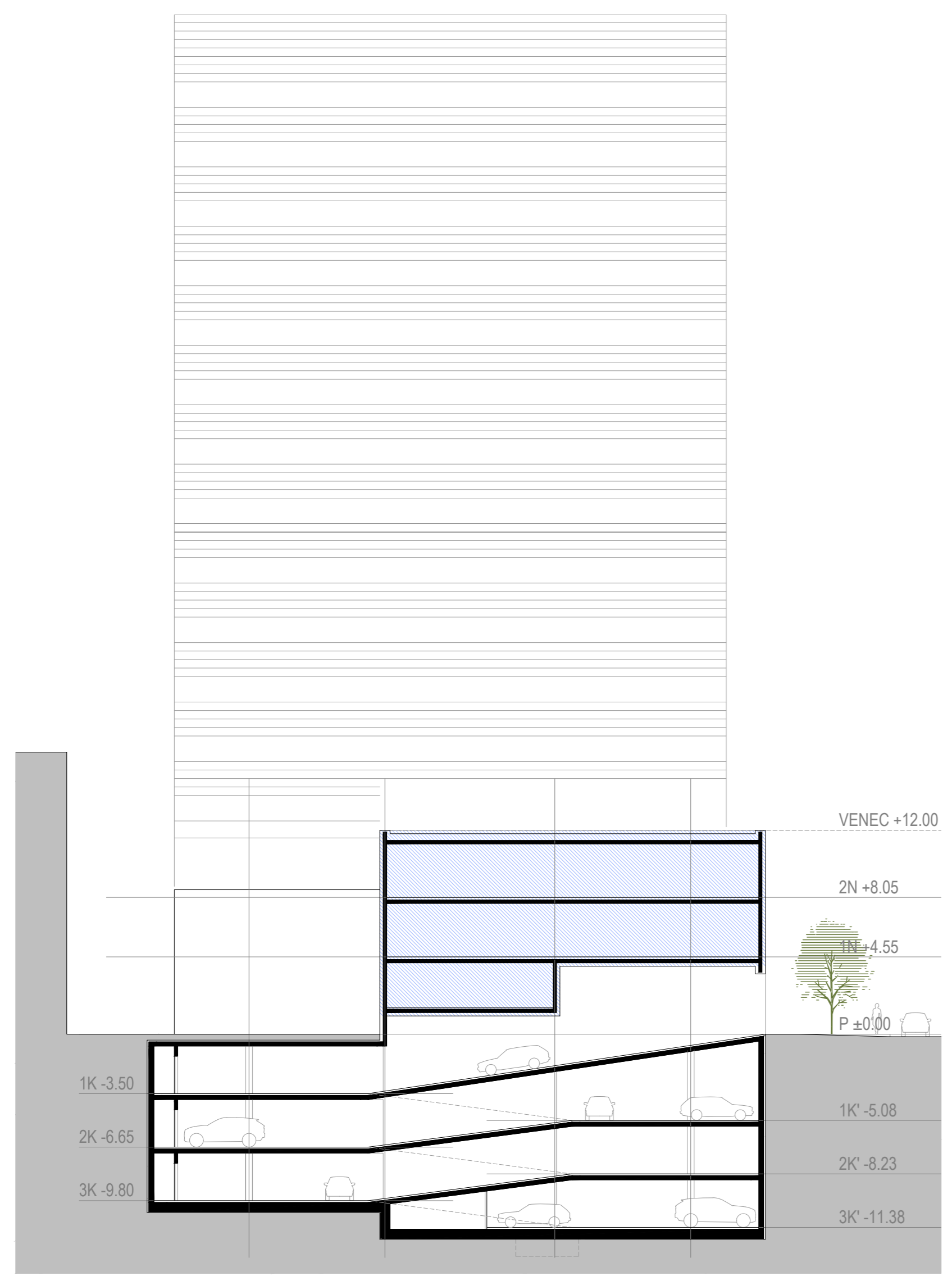
PREREZ C-C M 1:250
