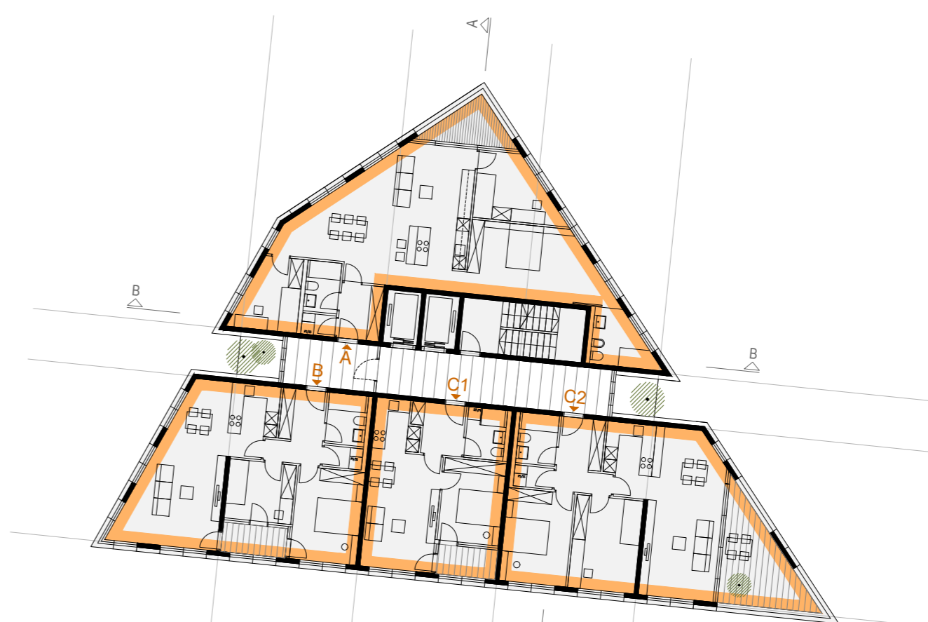
11.-12. NADSTROPJE M 1:250
