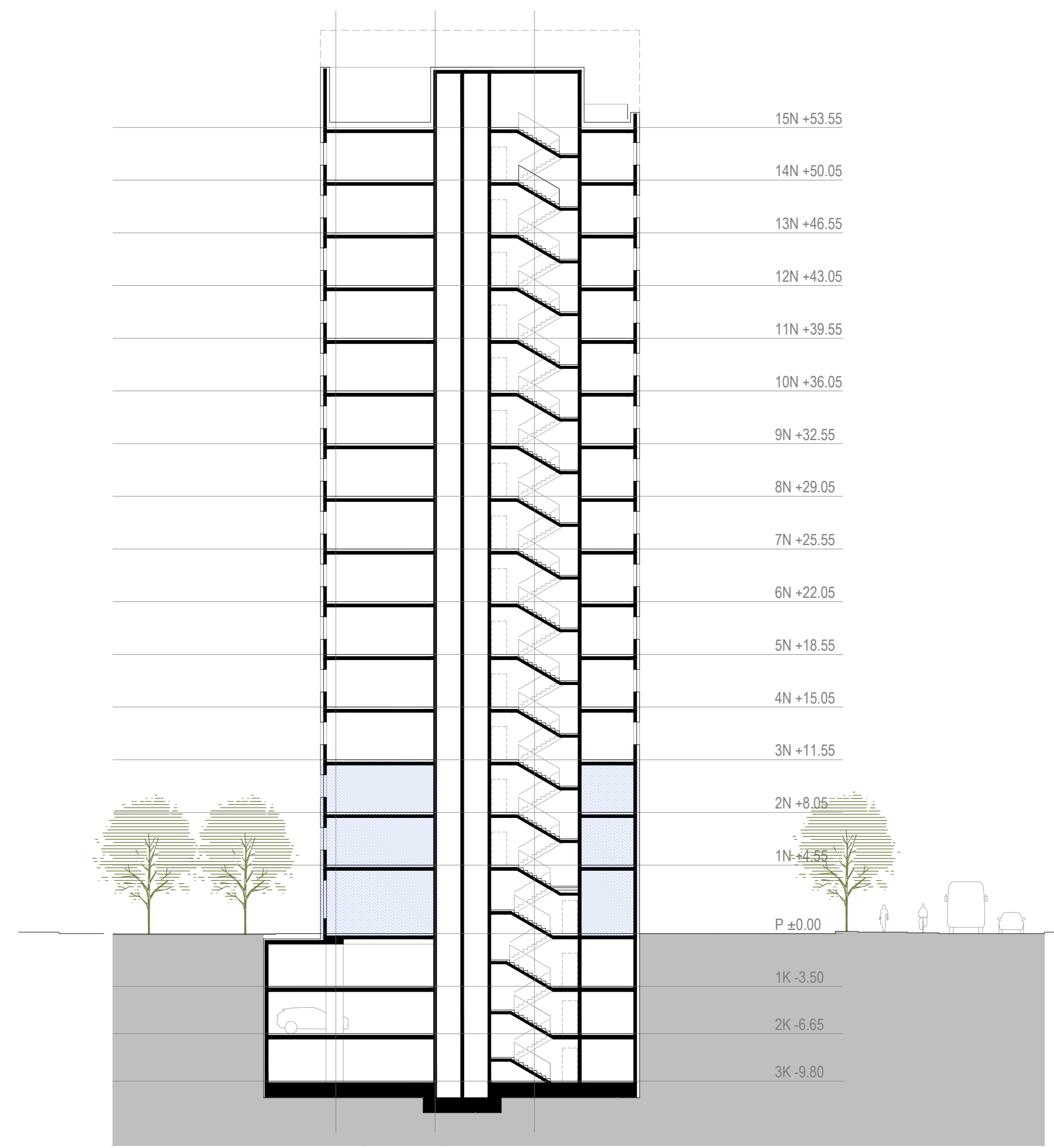
PREREZ B-B M 1:250
