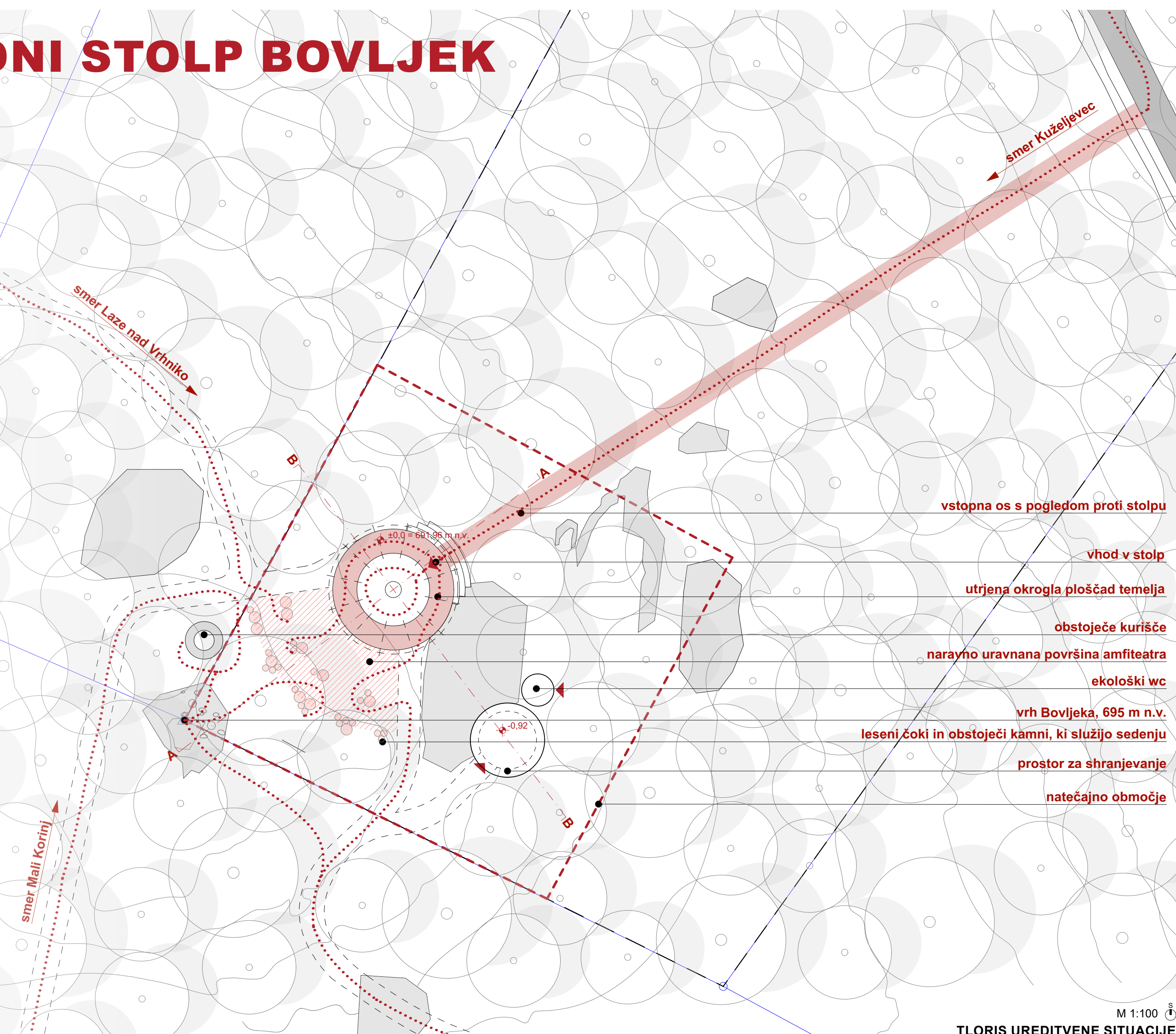
TLORIS UREDITVENE SITUACIJE
