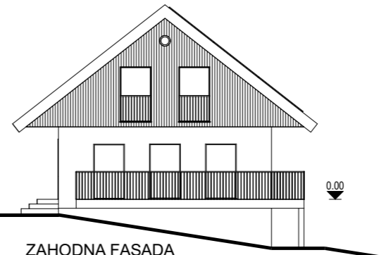
ZAHODNA FASADA
