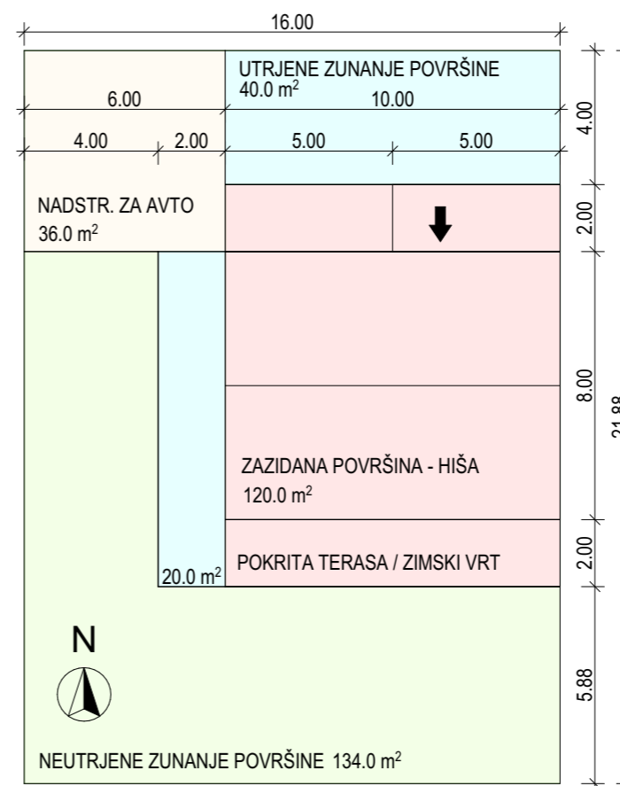
CELOTNA POVRŠINA GPS 350.0 m 2 M 1:200
