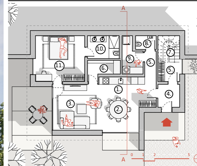
TLORIS 1. NADSTROPJA_M 1:200
