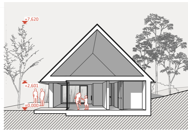
PREREZ A_M 1:200
