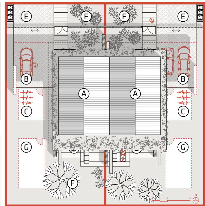
SITUACIJA_M 1:300
