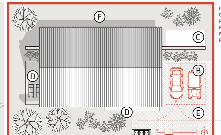
SITUACIJA_M 1:300
