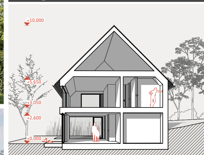
PREREZ A_M 1:200
