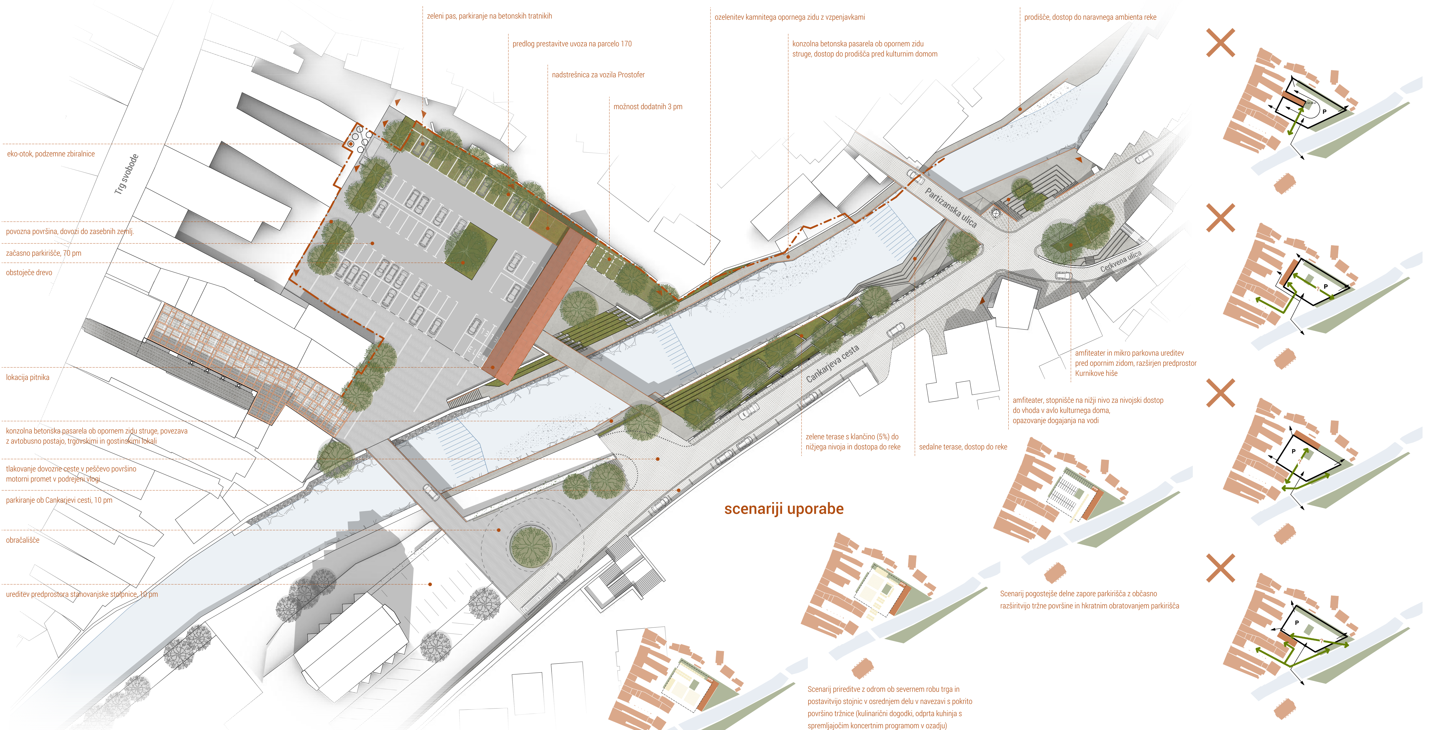
ureditvena situacija območja tržnice M 1:500
