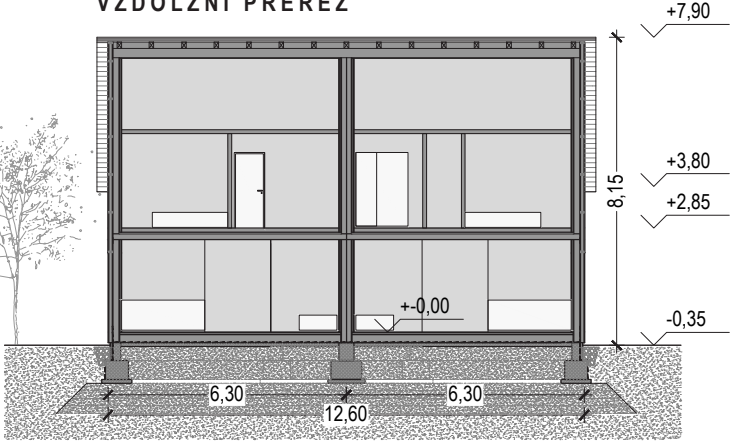
VZDOLŽNI PREREZ
