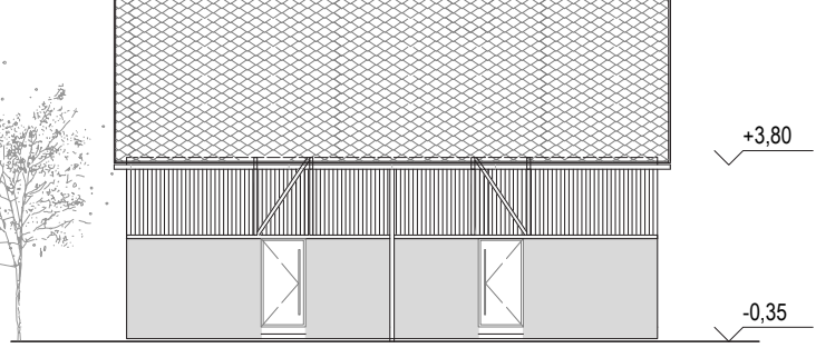
SEVERNA FASADA
