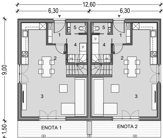
TLORIS PRITLIČJA, enota 1 in 2
