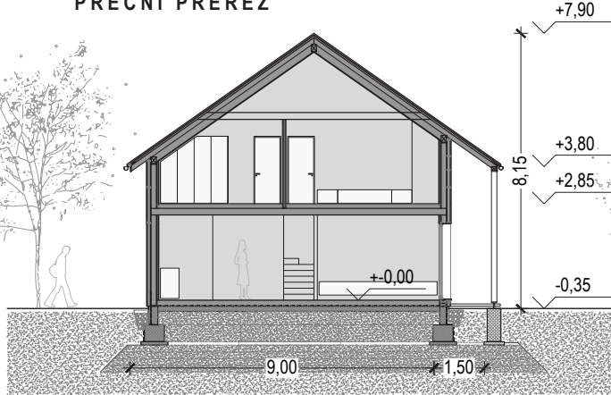
PREČNI PREREZ
