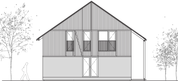
ZAHODNA FASADA
