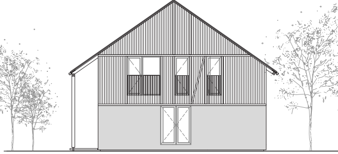
VZHODNA FASADA
