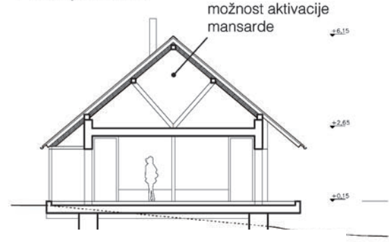
Prečni prerez AA
