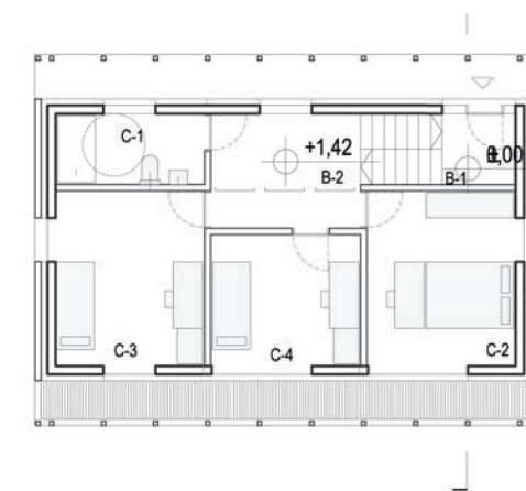
TLORIS NADSTROPJA M 1:200
