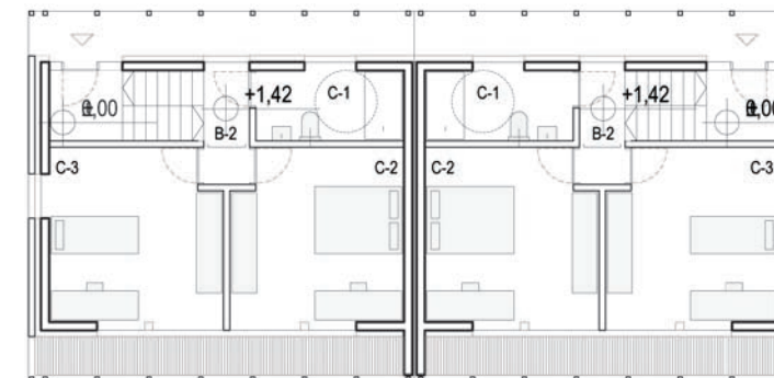
TLORIS NADSTROPJA M 1:200
