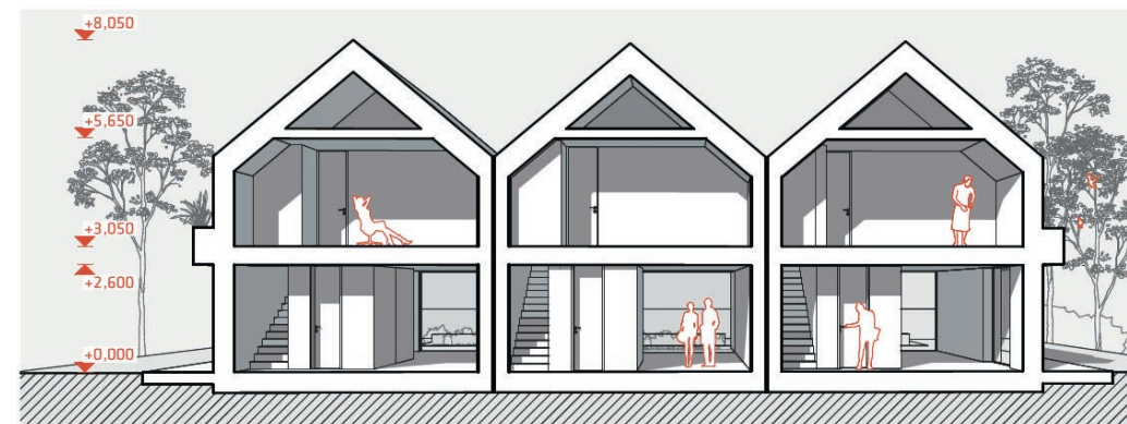
PREREZ A_M 1:200
