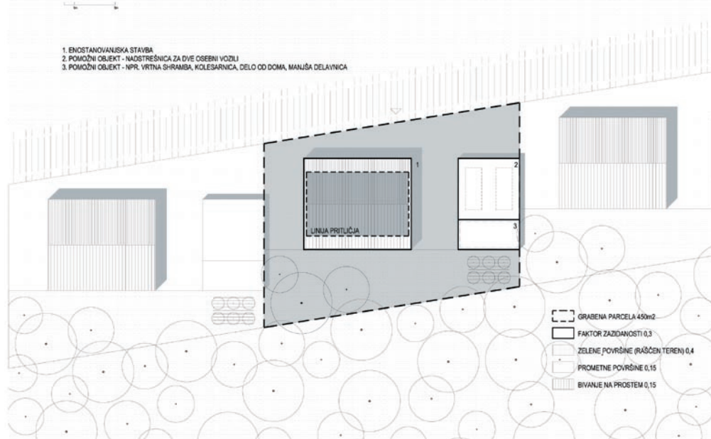
SHEMATSKI PRIKAZ ORGANIZACIJE PARCELE Z MOŽNO UMESTITVJO POMOŽNIH OBJEKTOV
