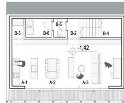
TLORIS PRITLIČJA M 1:200
