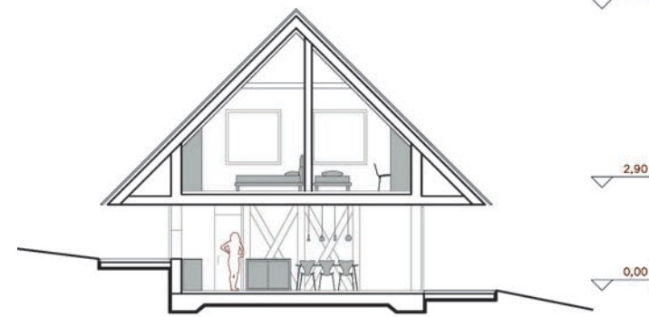
▼ PREREZ B-B 8,20
