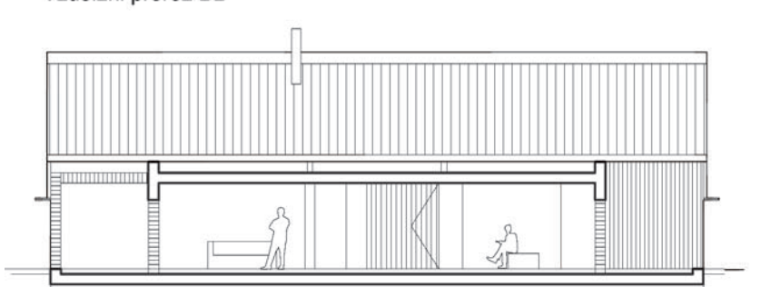
Vzdolžni prerez BB
