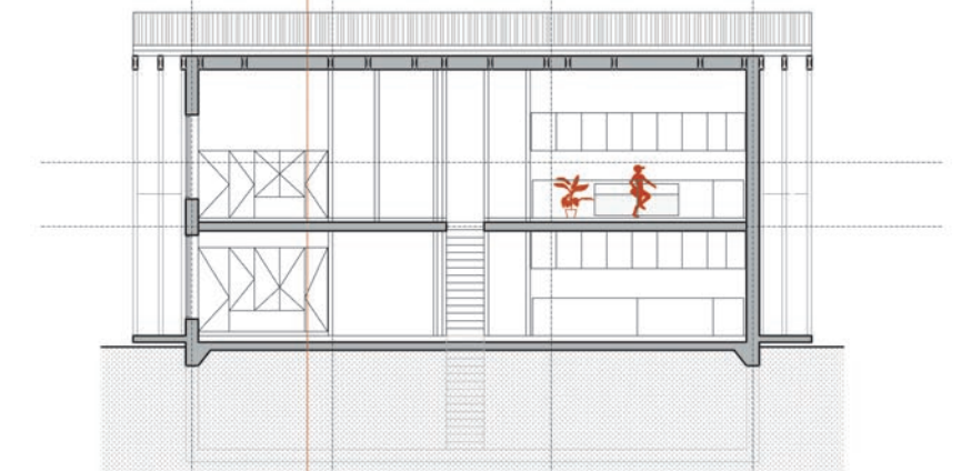
vzdolžni prerez M1:200
