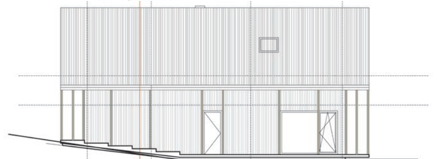
zahodna fasada M1:200
