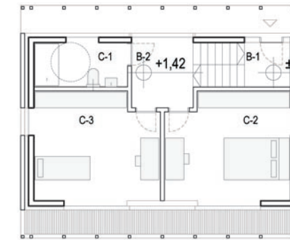
TLORIS NADSTROPJA M 1:200
