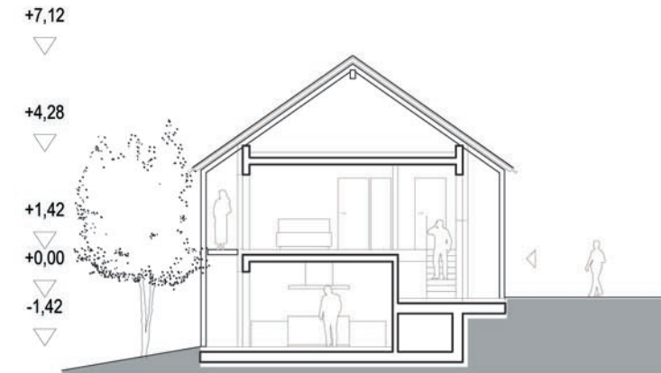
PREČNI PREREZ *M 1:200
