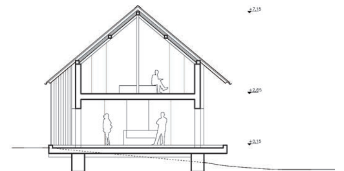
04. "ODEBELJENA" STENA PROSTORSKE RAZŠIRITVE
