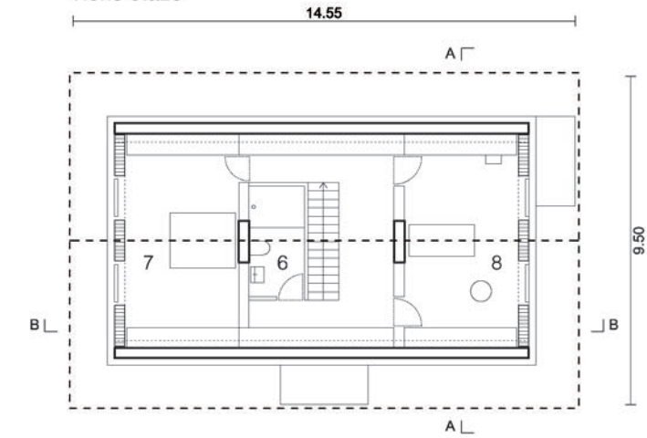
Tloris etaže
