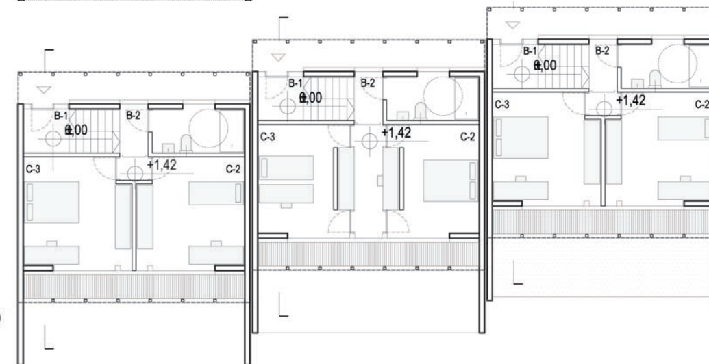
TLOORIS NADSTROPJA M 1:200
