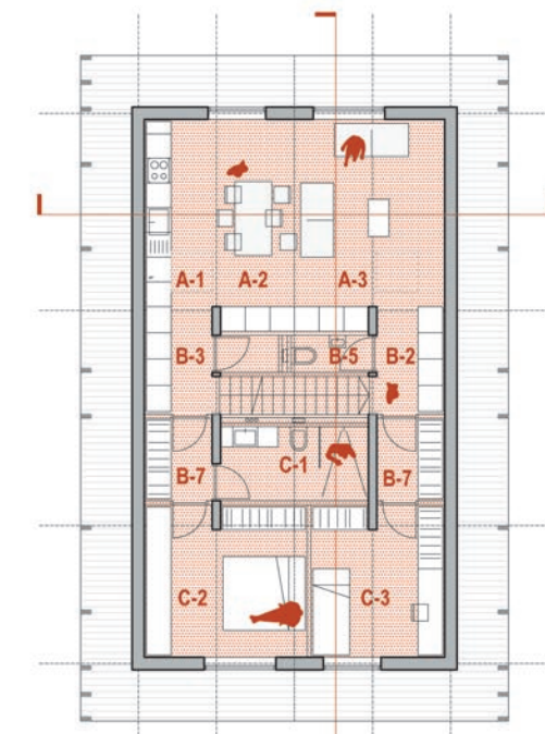
nadstropje M1:200
