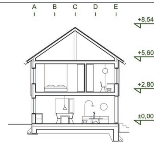
PREČNI PREREZ, m=1:200
