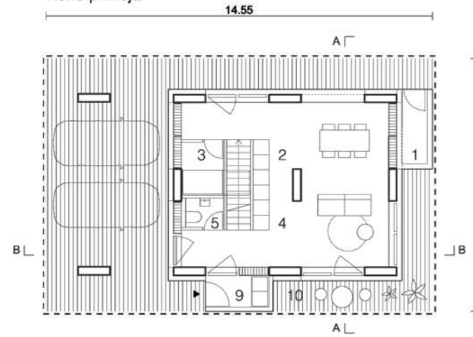
Tloris pritličja
