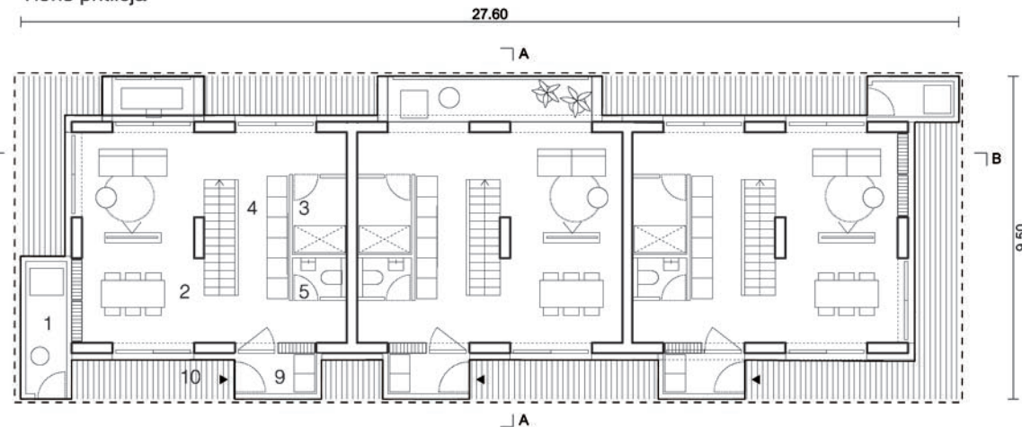
Tloris pritličja
