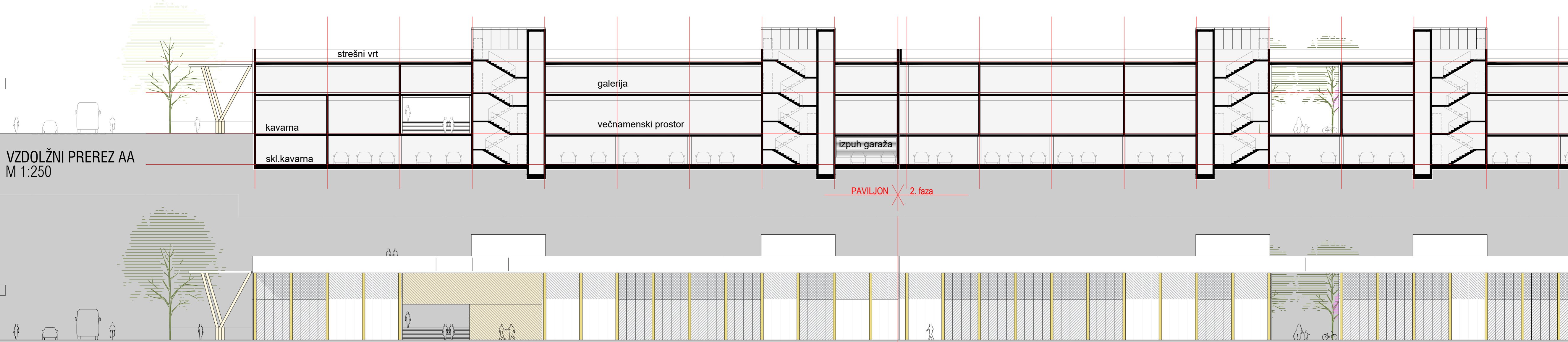
VZDOLŽNI PREREZ AA M 1:250
