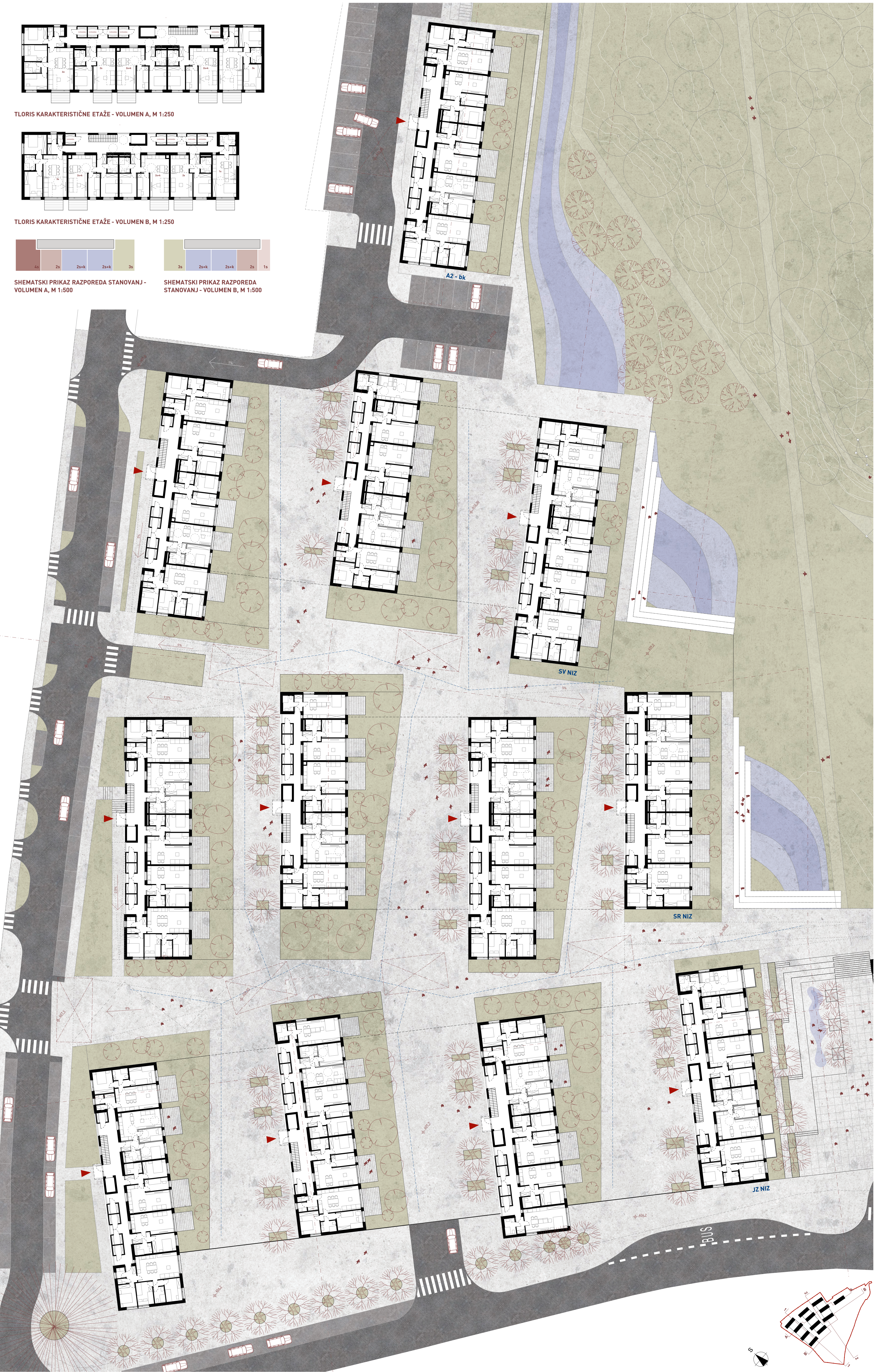
SITUACIJA S TLORISI PRITLIČIJ, M 1:250
