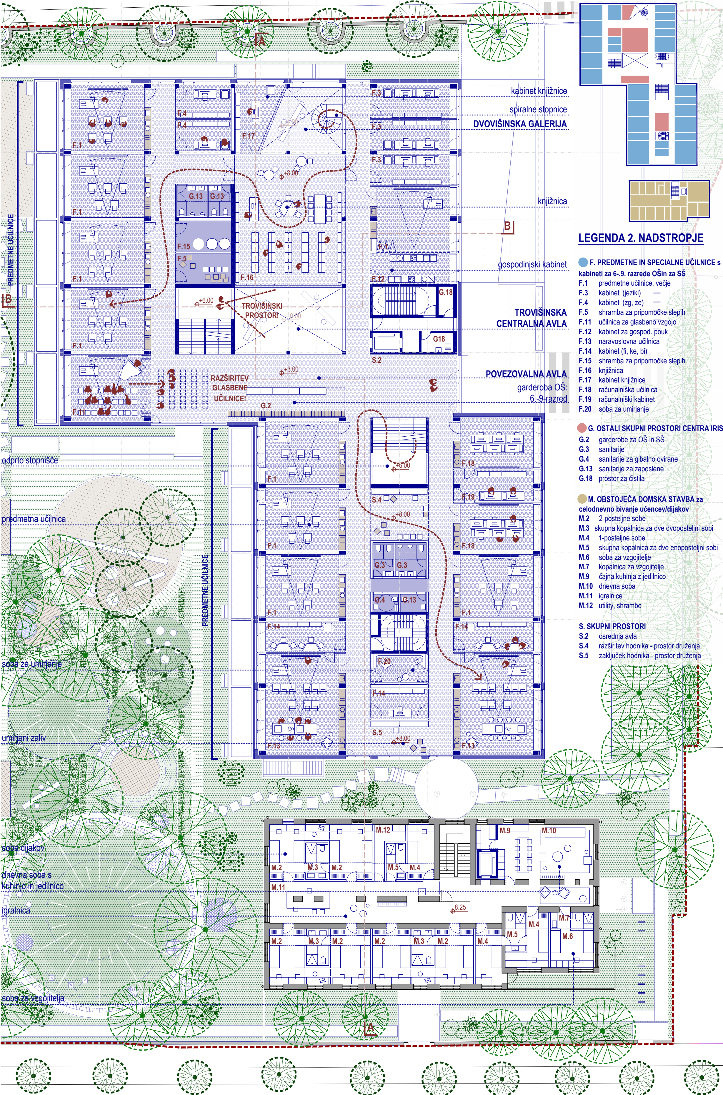
TLORIS 2. NADSTROPJA M 1:200
