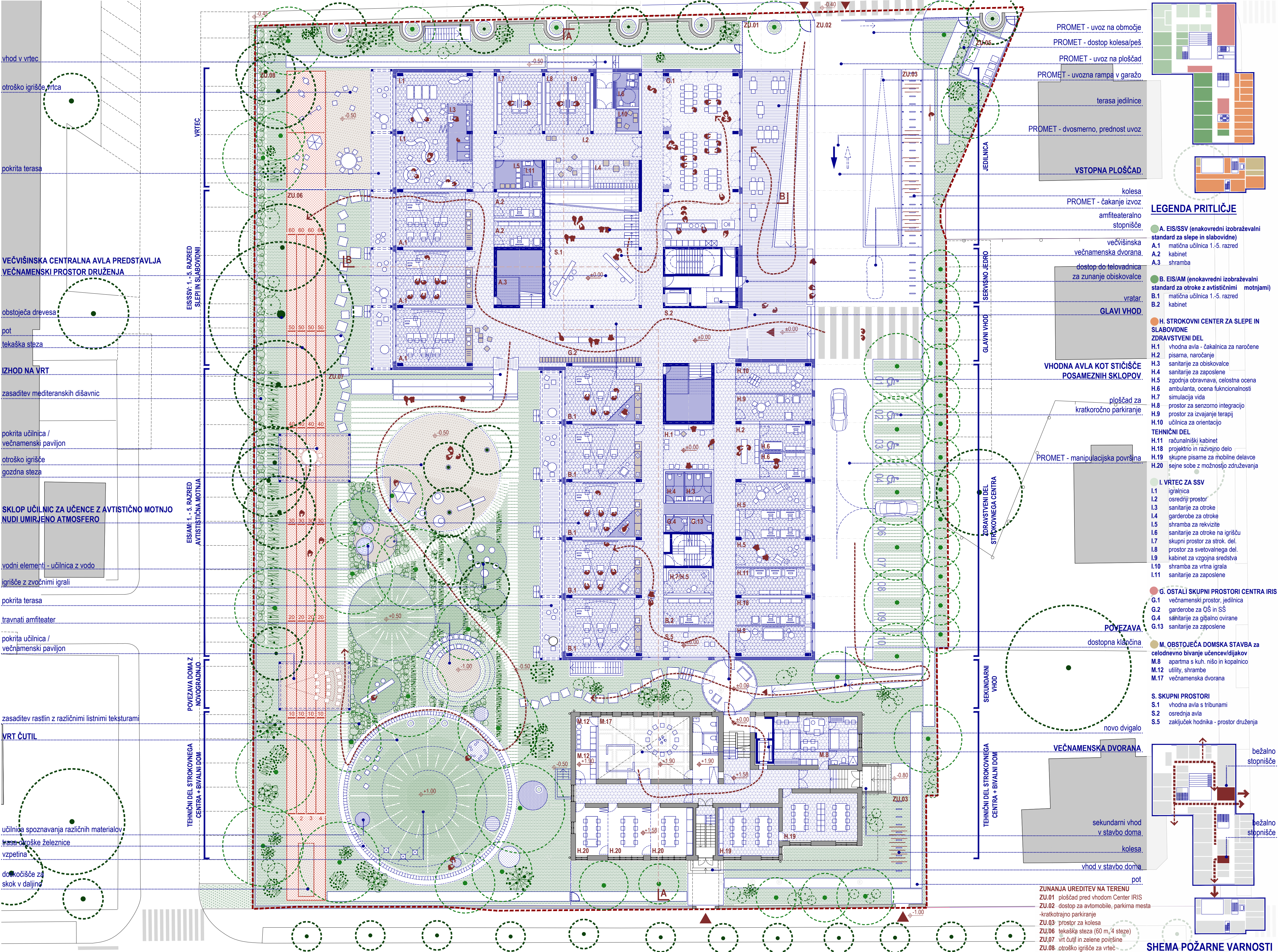
TLORIS PRITILČJA Z ZUNANJO UREDITVIJO IN PROMETNO UREDITVIJO M 1:200
