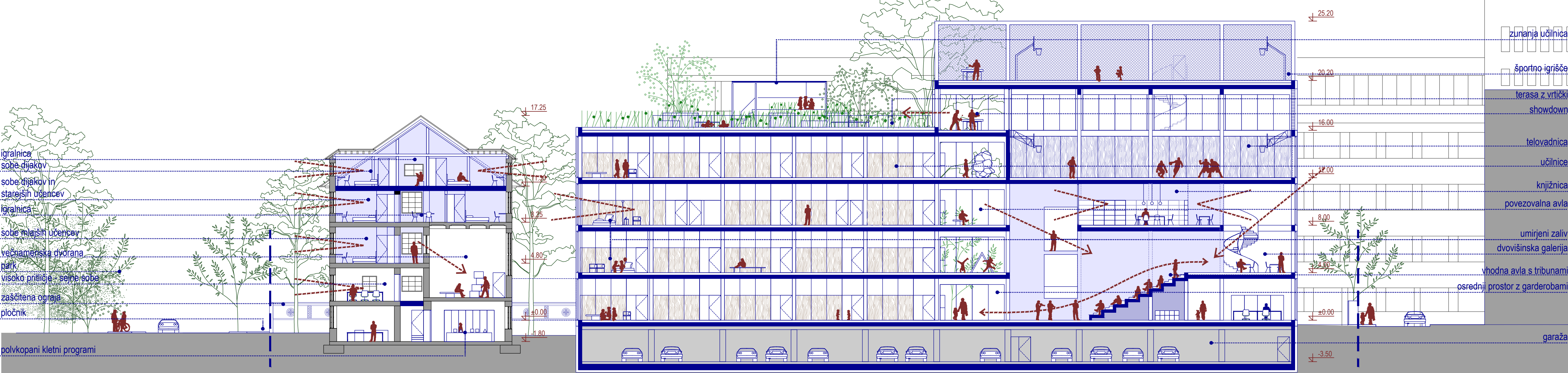
VZDOLŽNI PREREZ M 1:200
