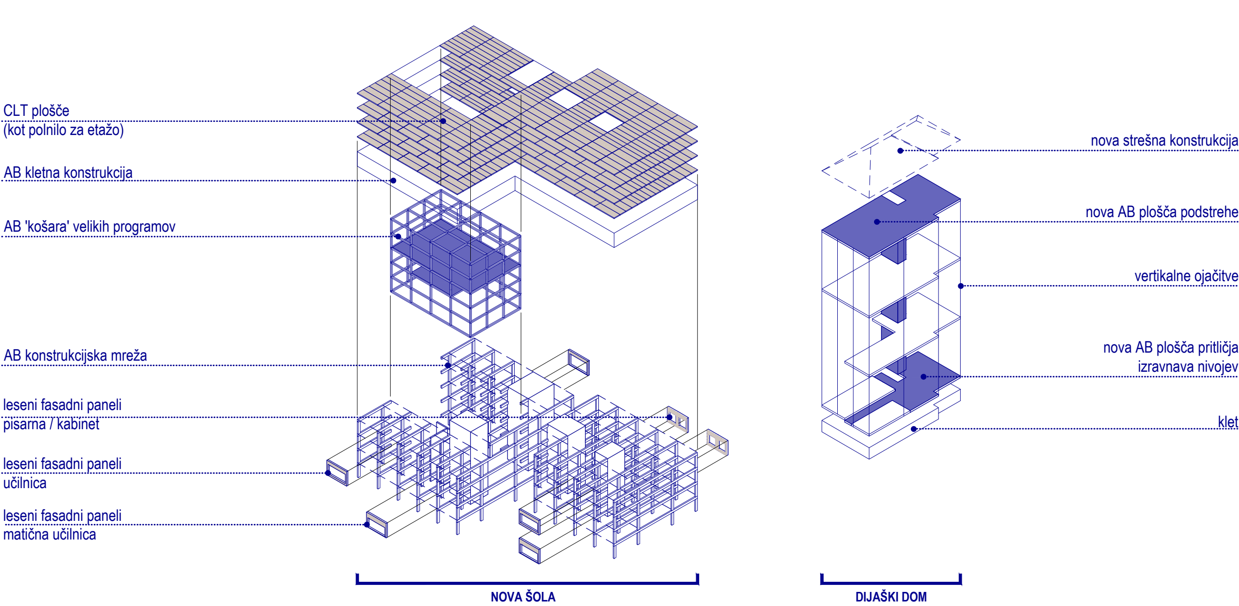
ŠOLA JE KONSTRUKCIJSKI HIBRID AB KONSTRUKCIJE, CLT LESENIH ETAŽNIH PLOŠČ, S BETONSKO 'KOŠARO' VELIKIH PROGRAMOV V 'SRCU'.
