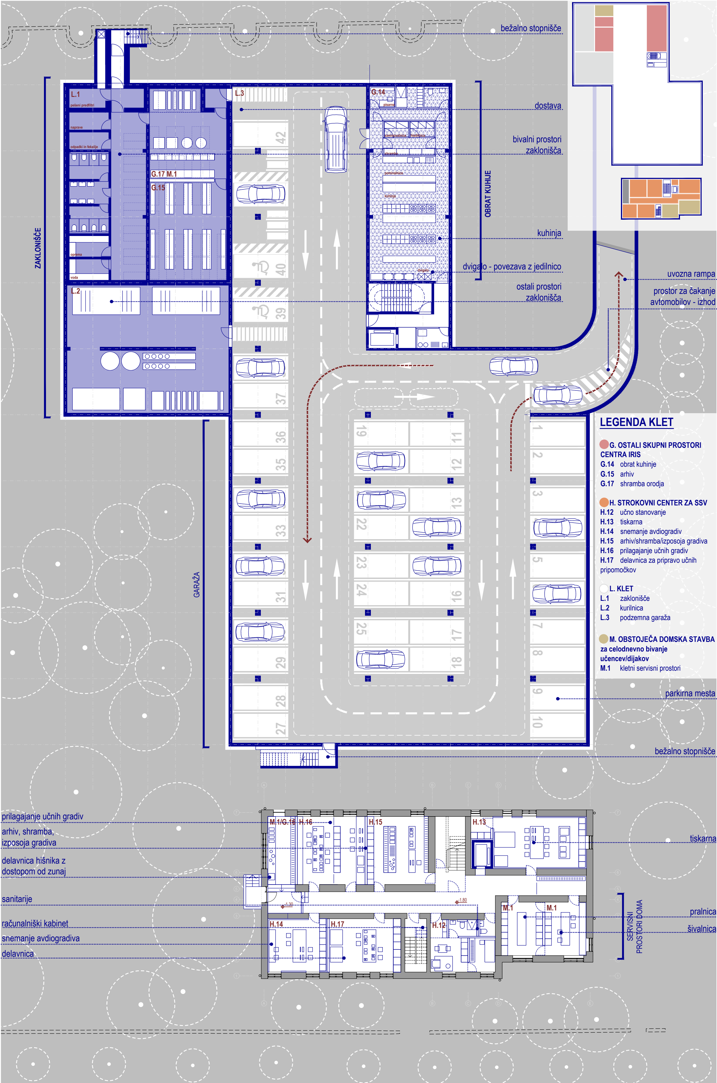
TLORIS KLETI M 1:200
