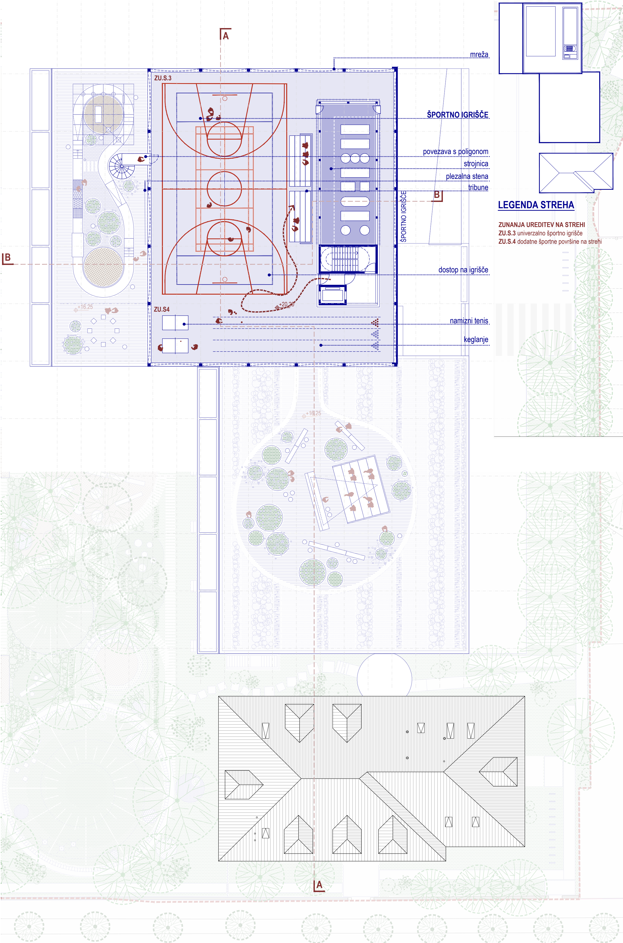
TLORIS STREHE M 1:200
