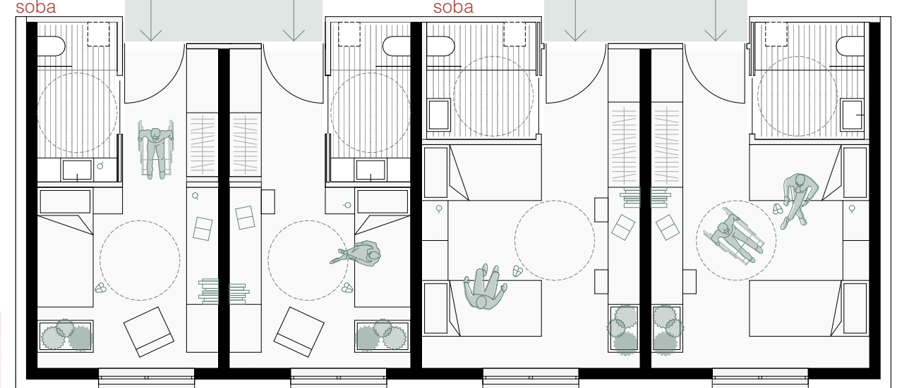
SEMA SOBE 1:100
