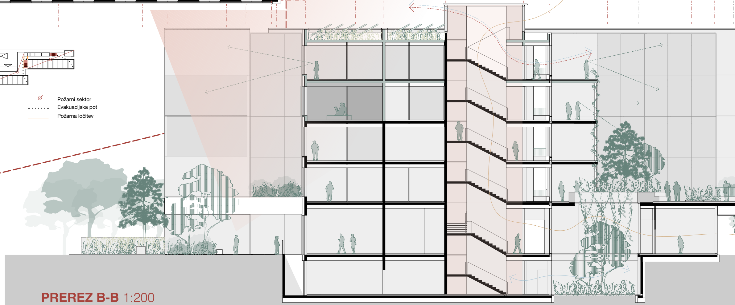
PREREZ B-B 1:200
