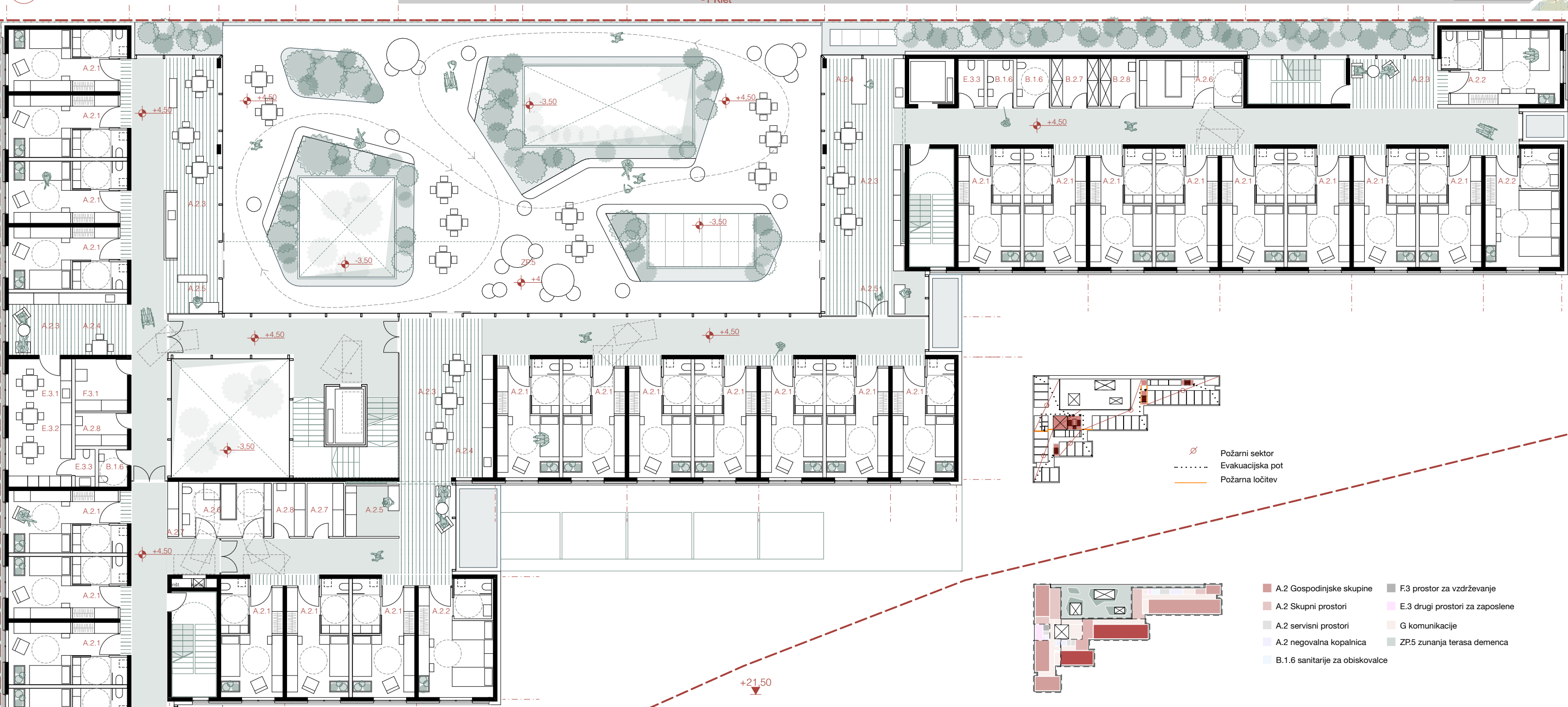
TLORIS 1. NADSTROPJA 1:200
