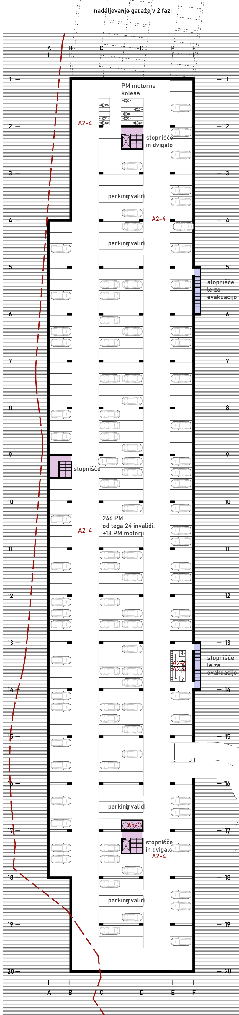
TLORIS KLETI -3.9m M 1:500
