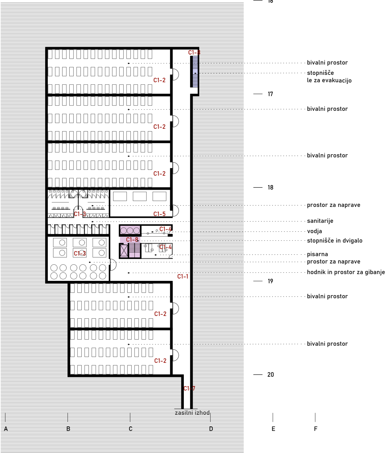
TLORIS ZAKLONIŠČA -8.5m M 1:500
