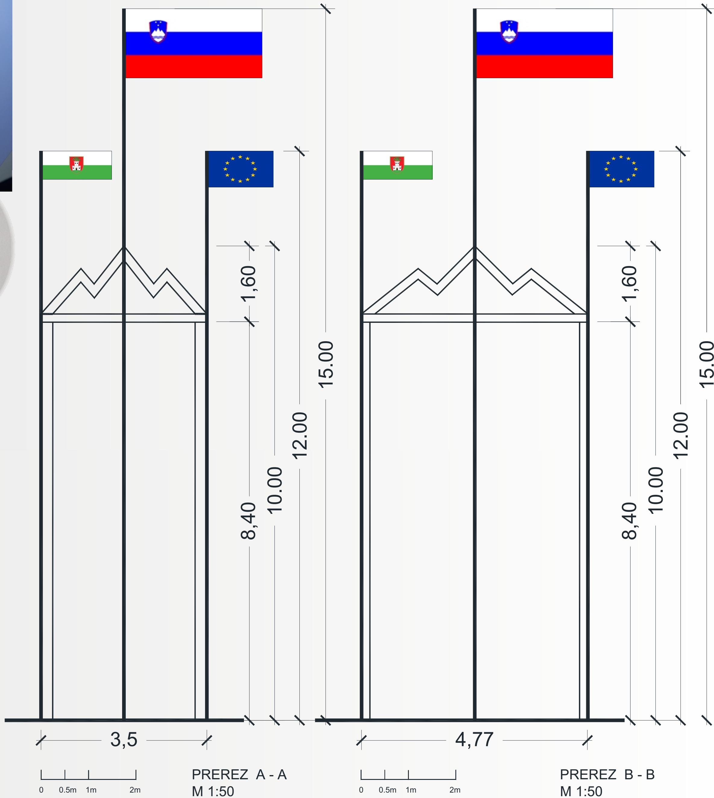
NAČRTI : TLORIS, PREREZ A - A, PREREZ B - B
