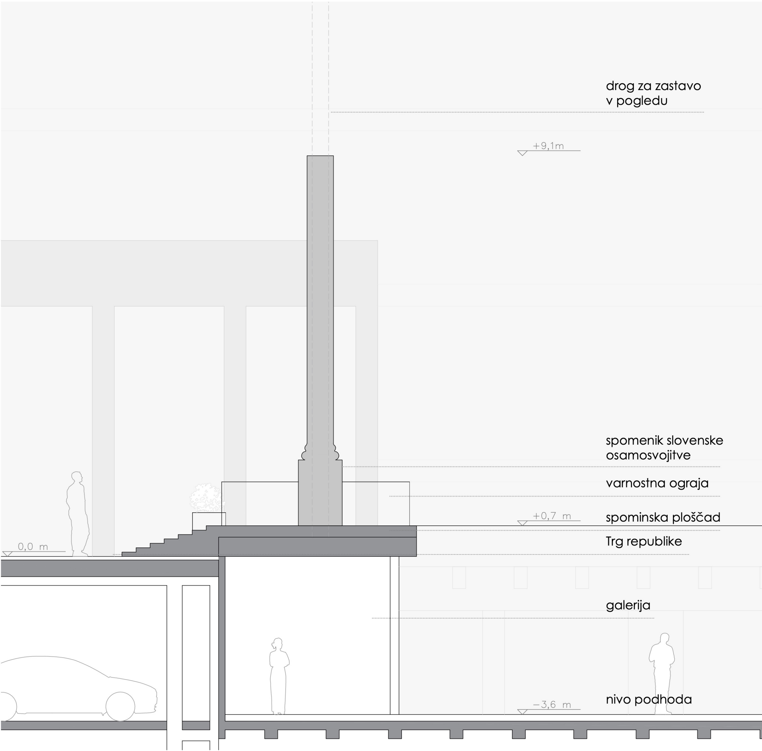
Prerez V-Z v merilu M50.
