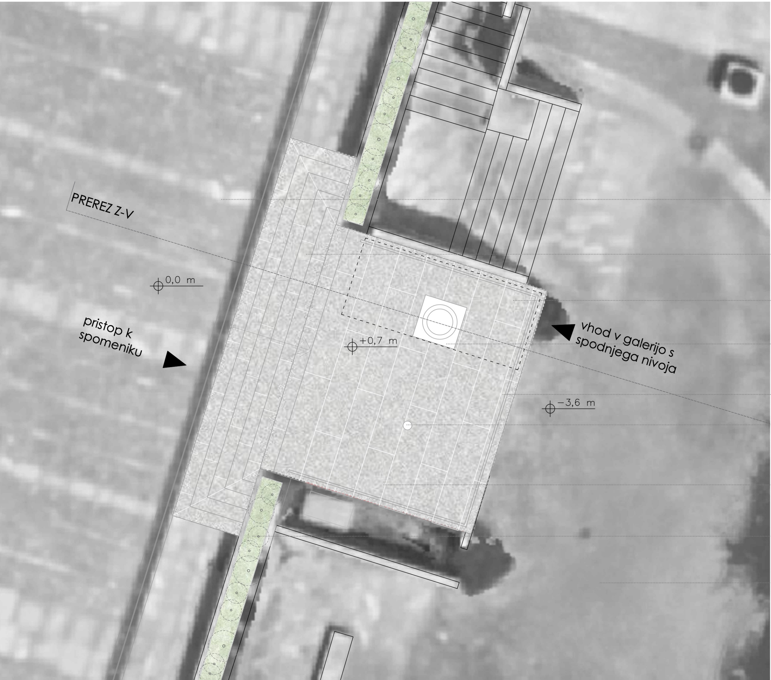
Tloris območja spomenika v merilu 1:50.
