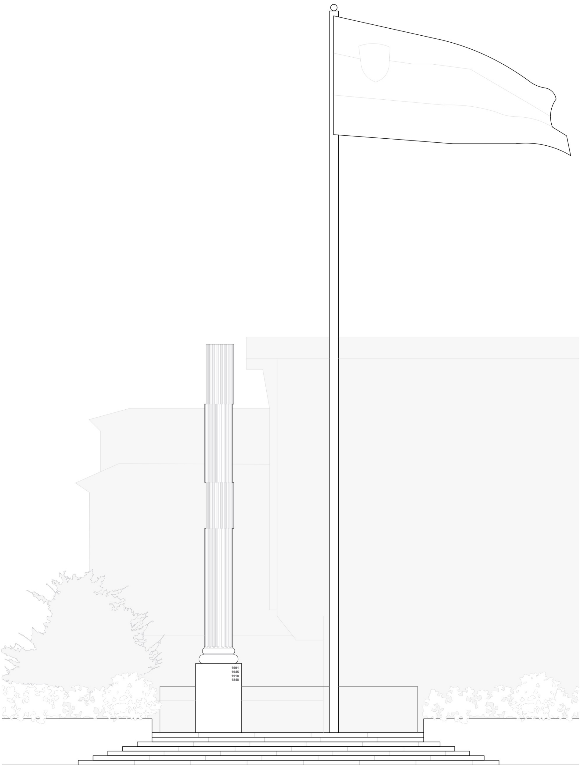
Pogled na spomenik z zahoda, v merilu 1:50.
