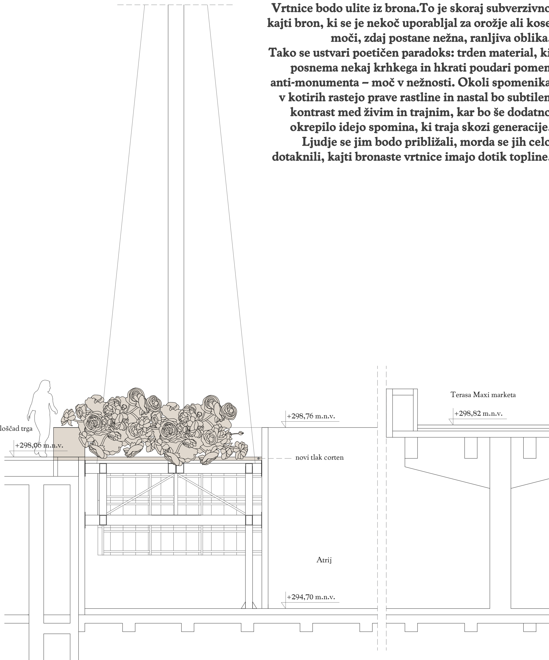
PREREZ M 1:50
