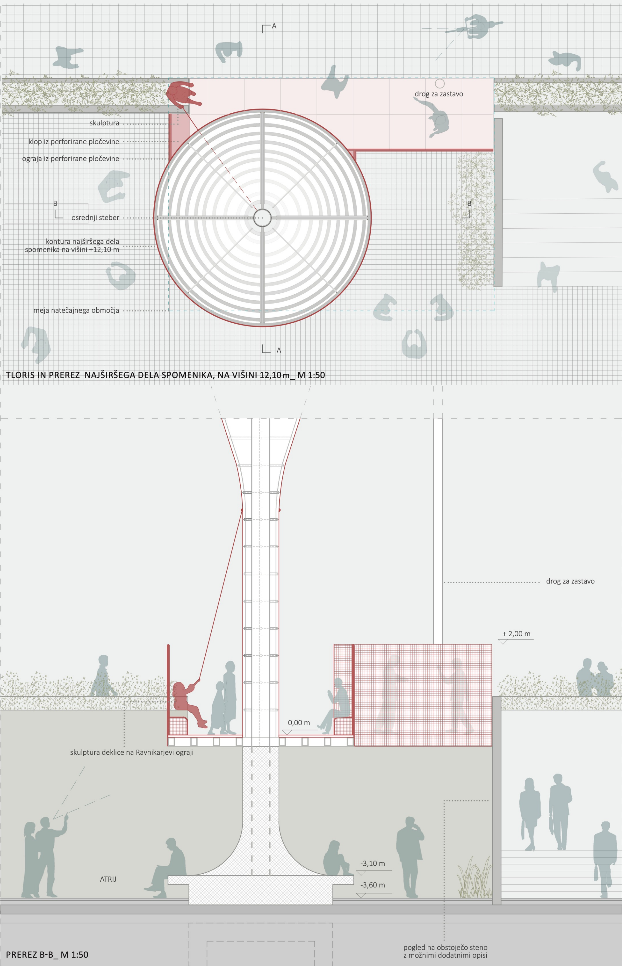
PREREZ B-B_M 1:50
