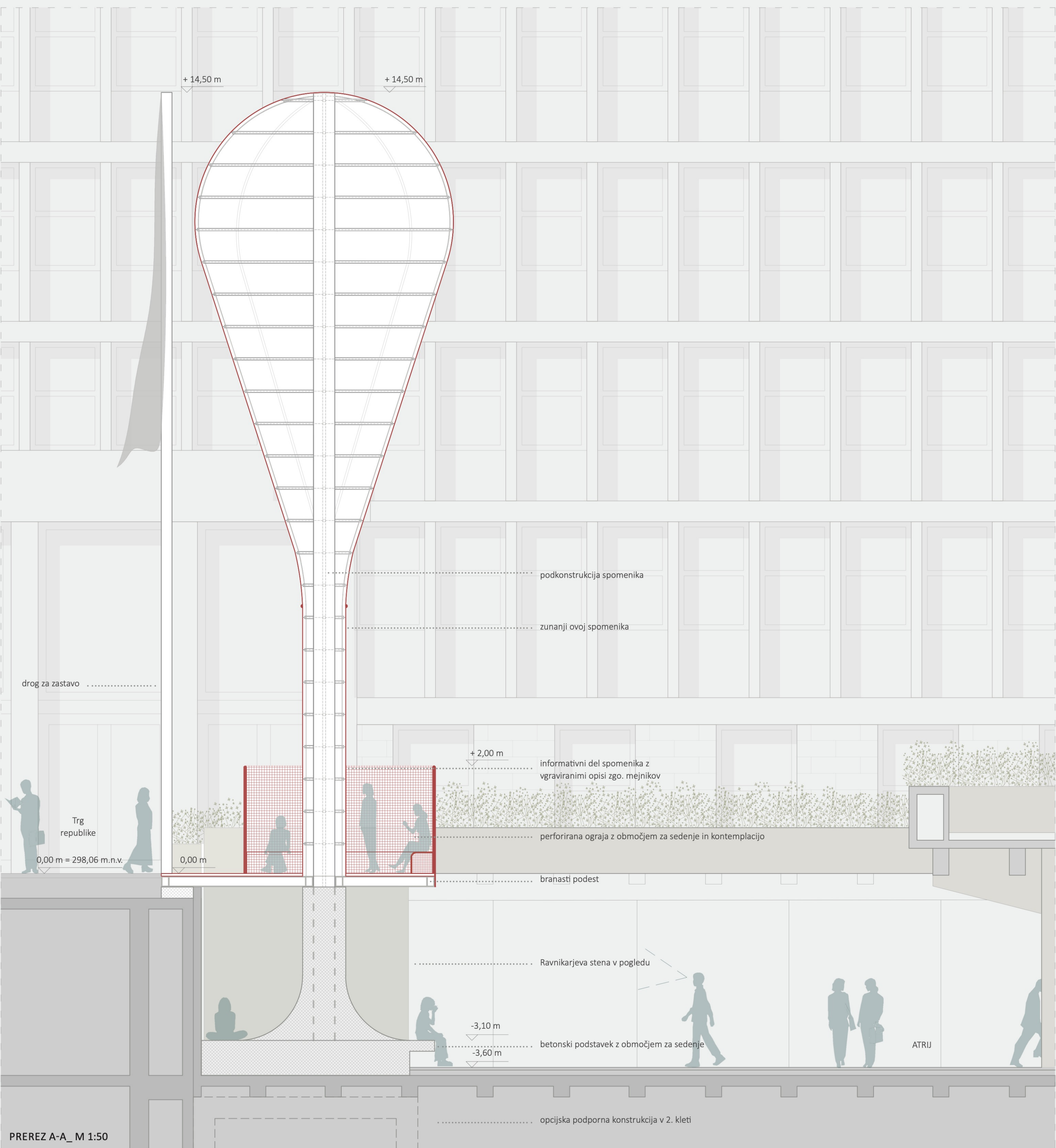
PREREZ A-A_M 1:50
