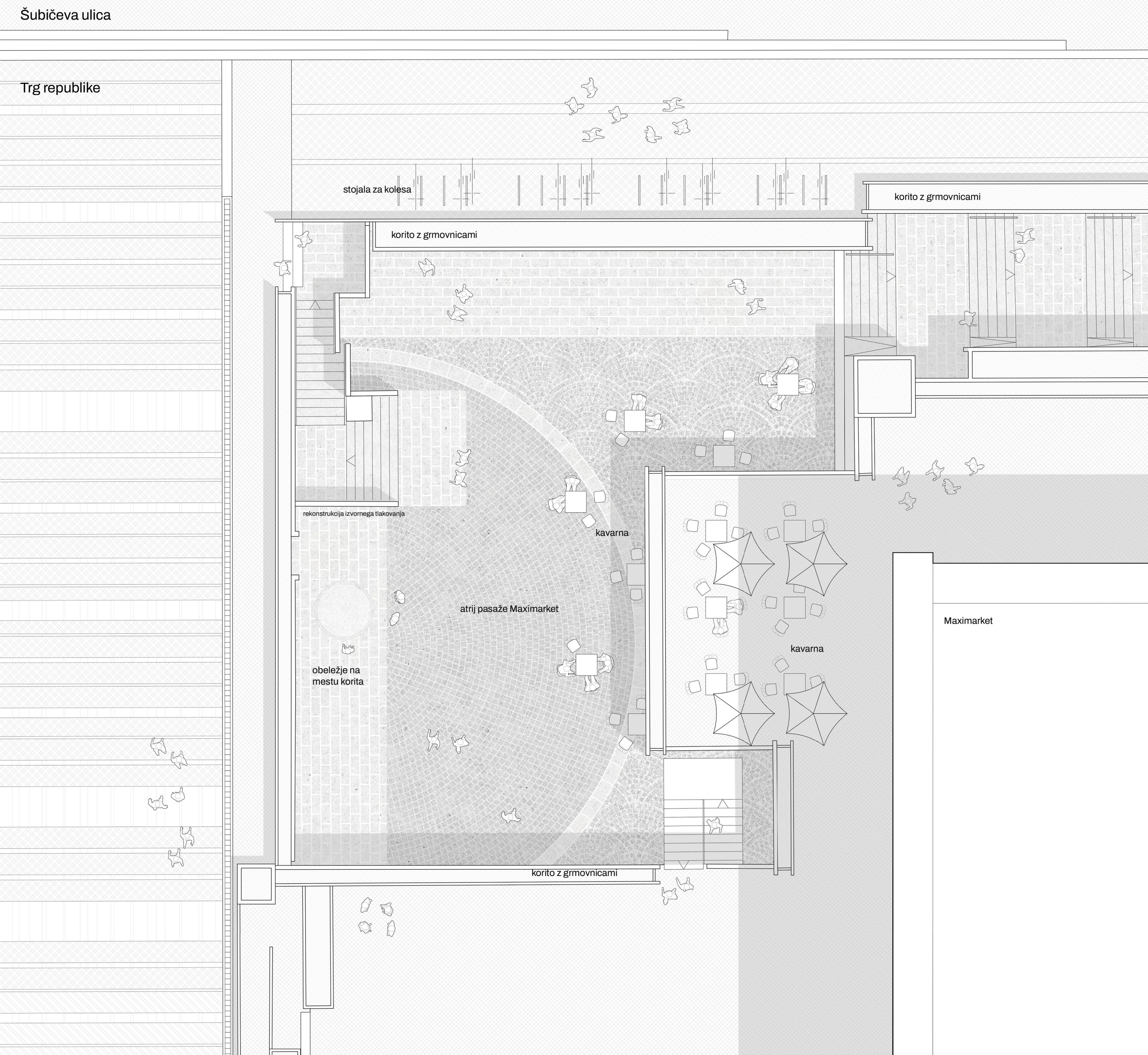
TLORIS ATRIJA PASAŽE MAXIMARKET, M 1:100
