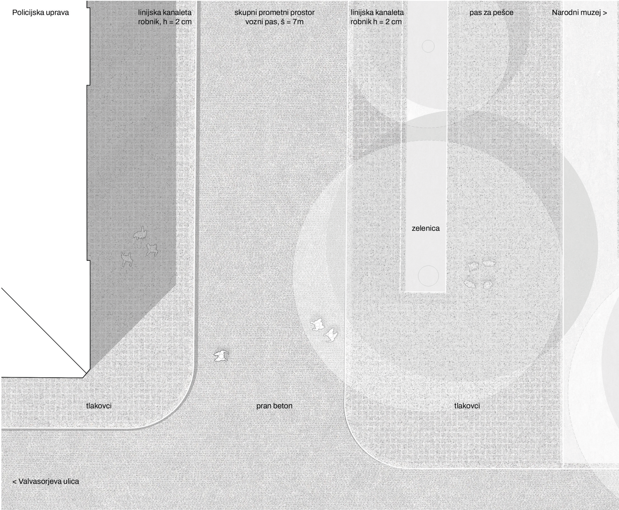
TLAKOVANJE ŠUBIČEVE ULICE, ZAHODNI ROB, M 1:100
