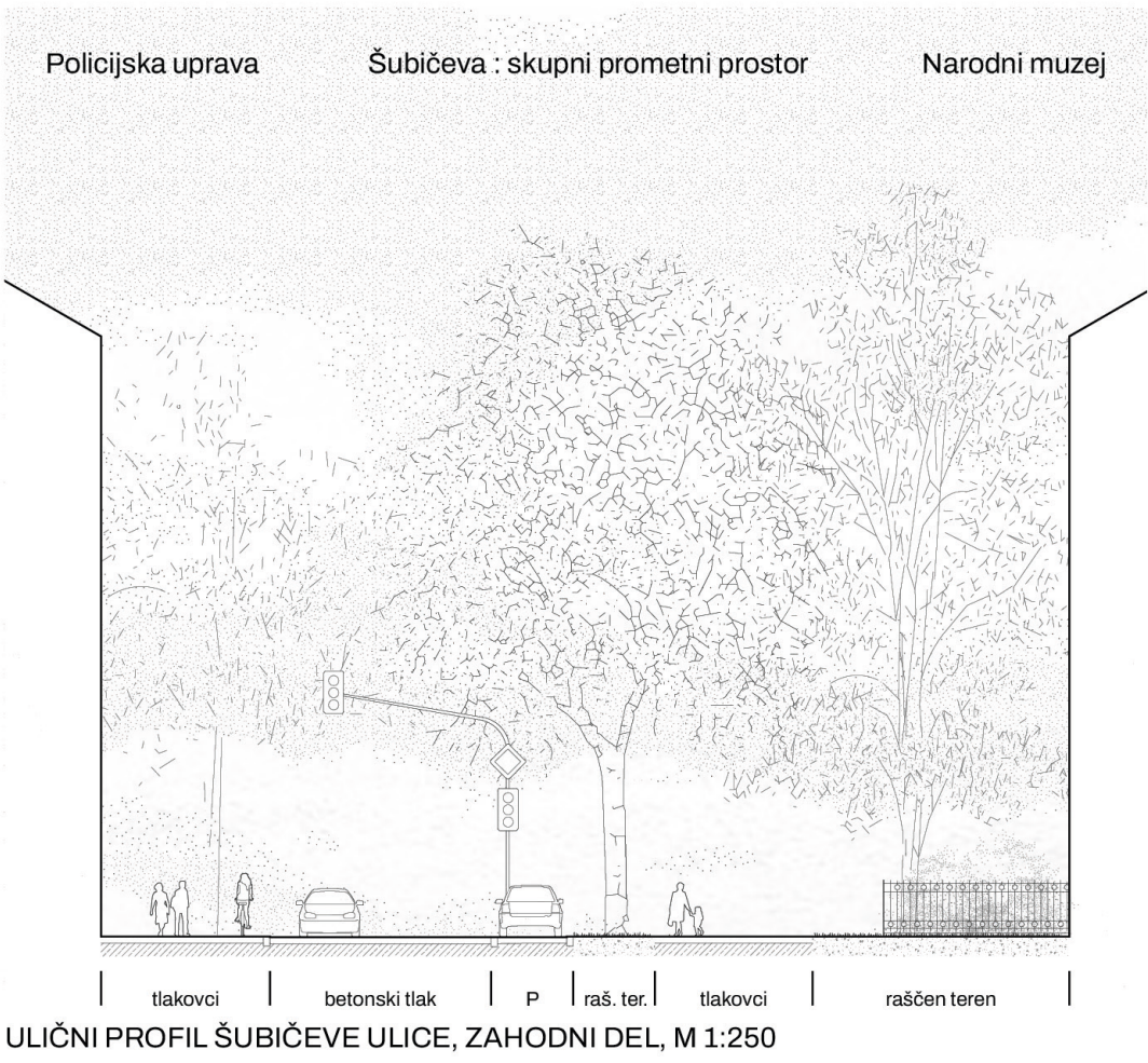
ULIČNI PROFIL ŠUBIČEVE ULICE, ZAHODNI DEL, M 1:250
