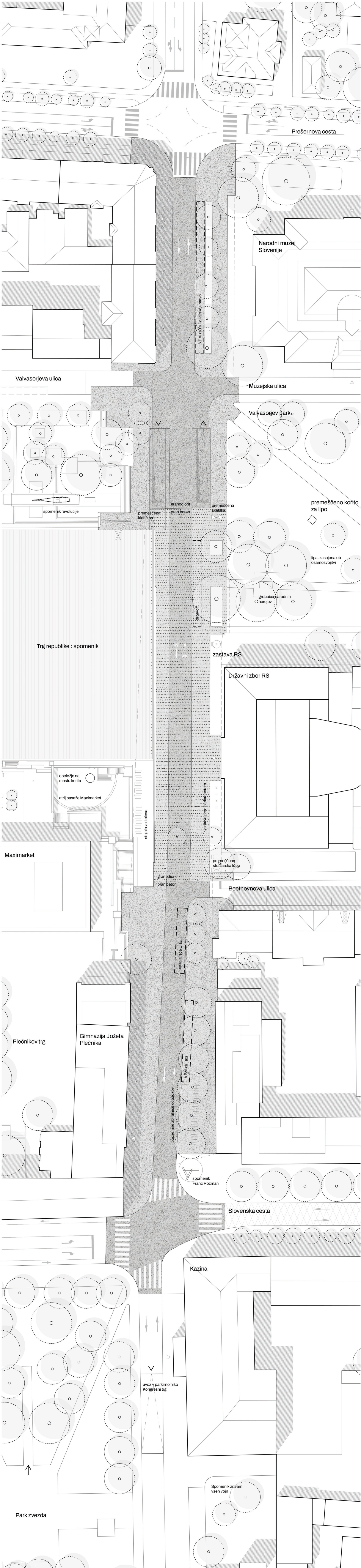
UREDITEV ŠUBIČEVE ULICE, SITUACIJA M 1:500
