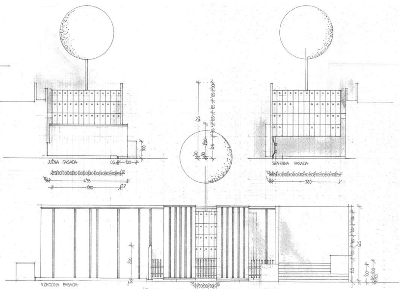
KORITO ZA LIPO, NAČRT DATIRAN 20. 6. 1991 (I)
