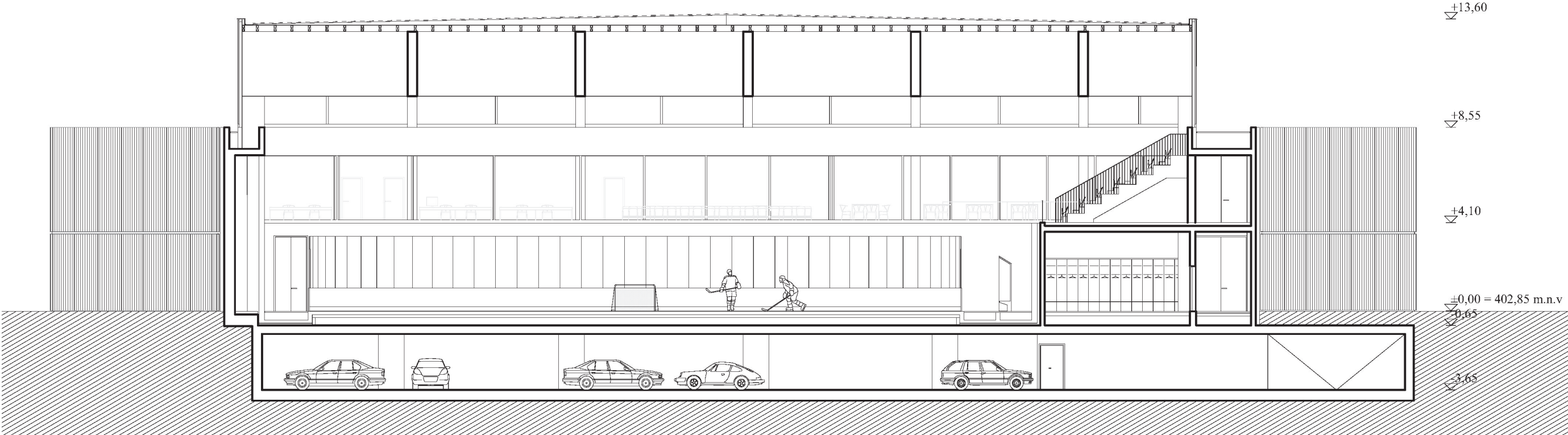
Prečni prerez
