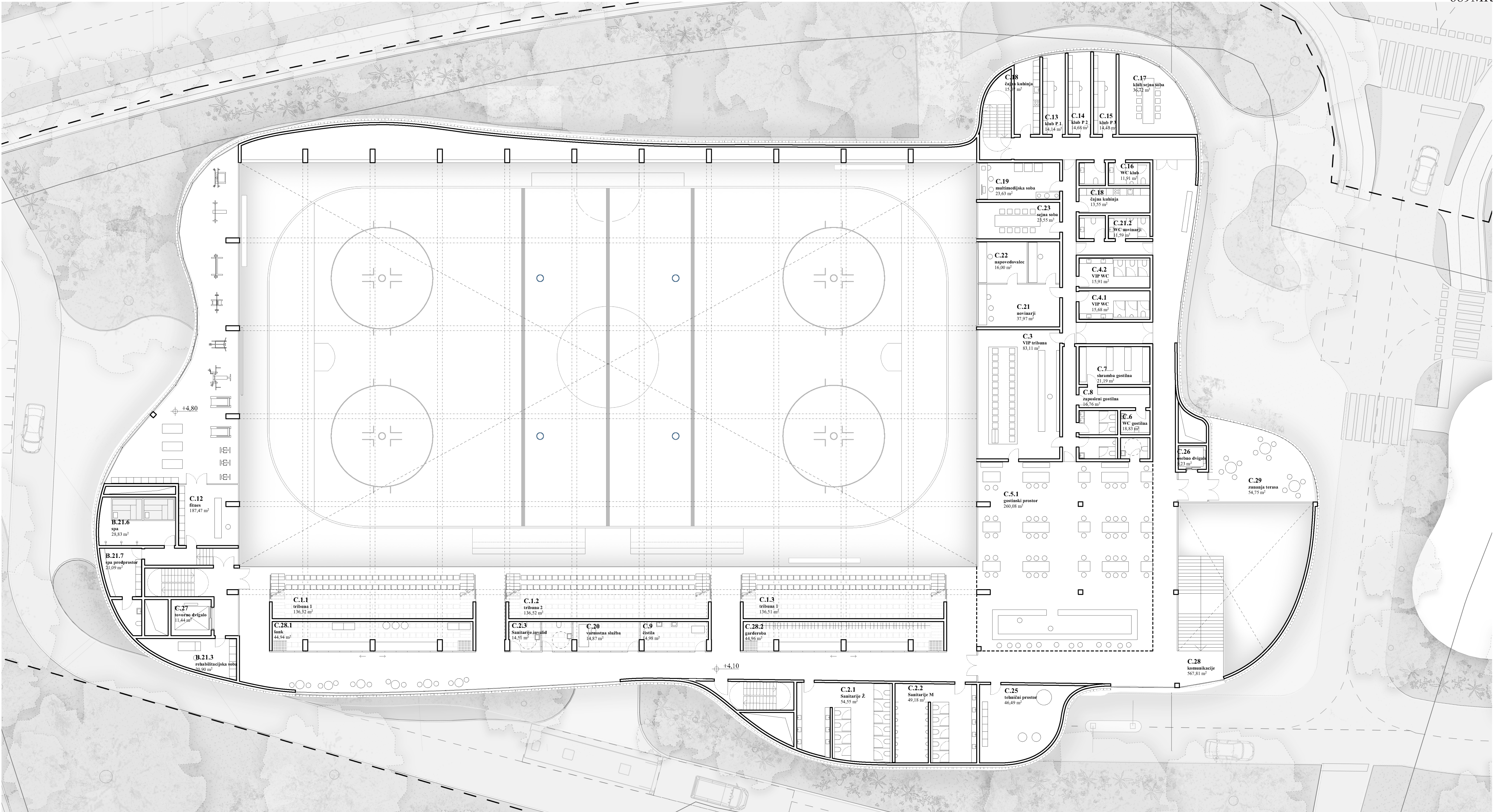
Tloris 1. nadstropja
