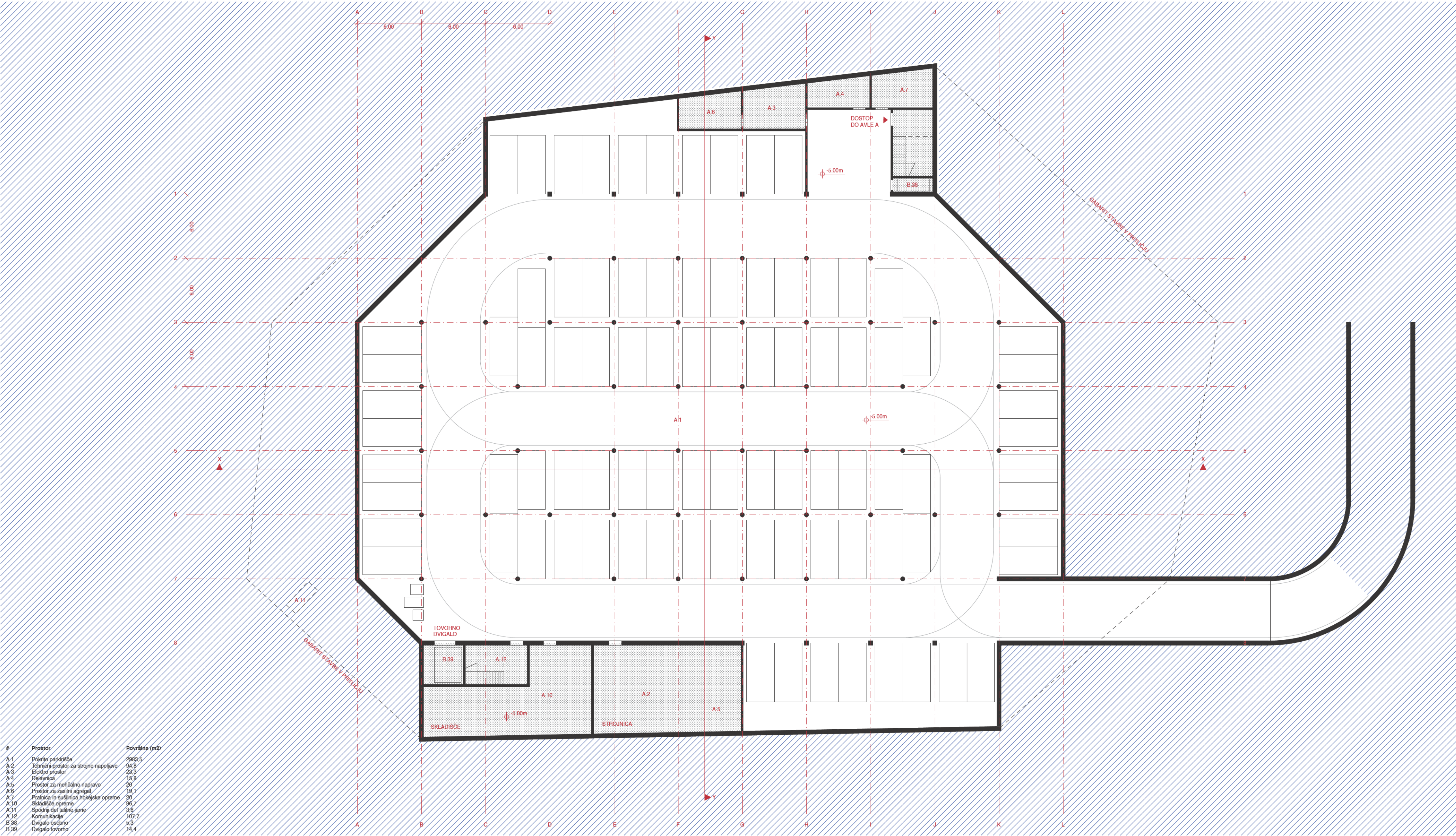
Tloris kleti M 1:200
