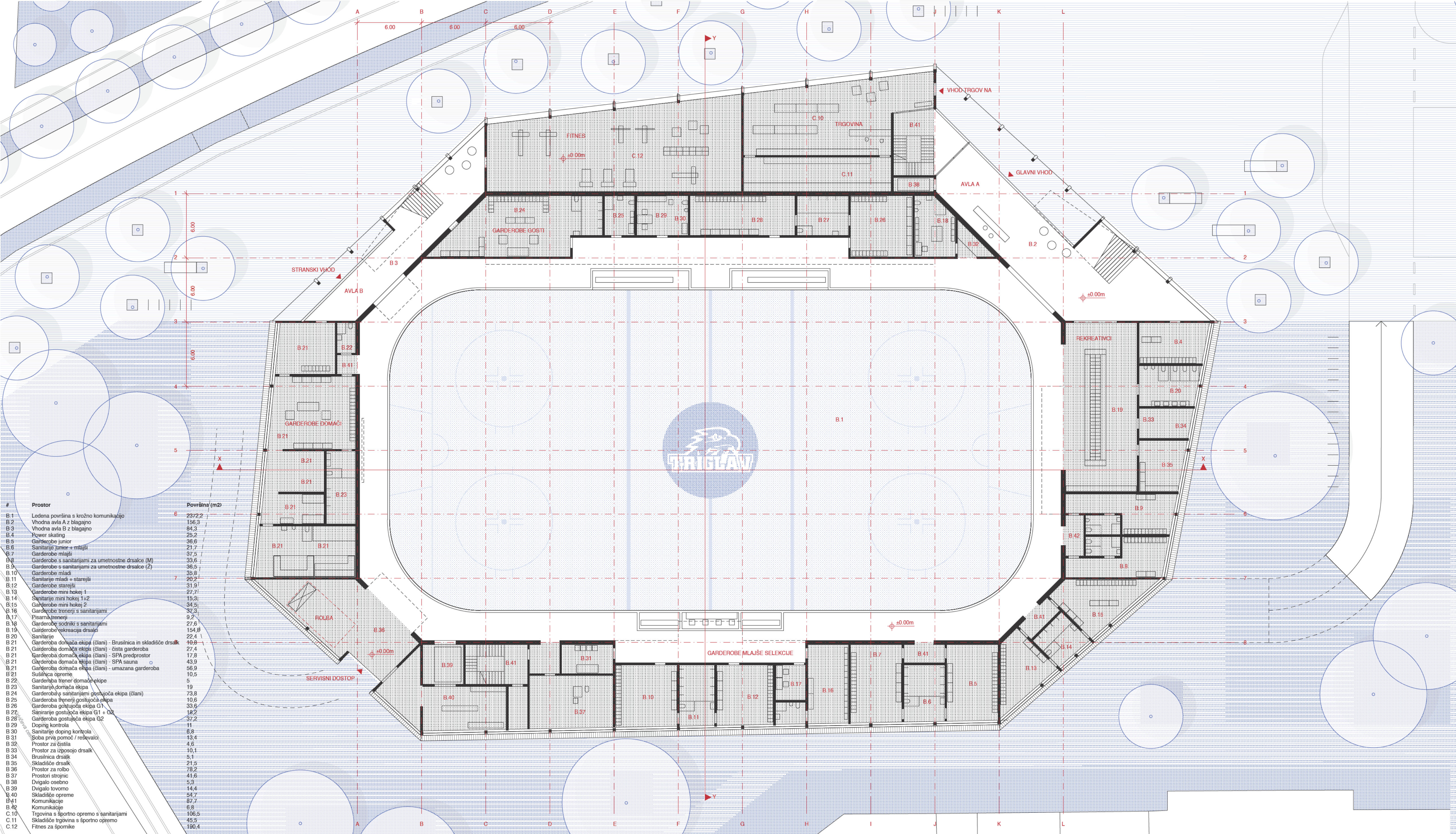
Tloris pritličja M 1:200
