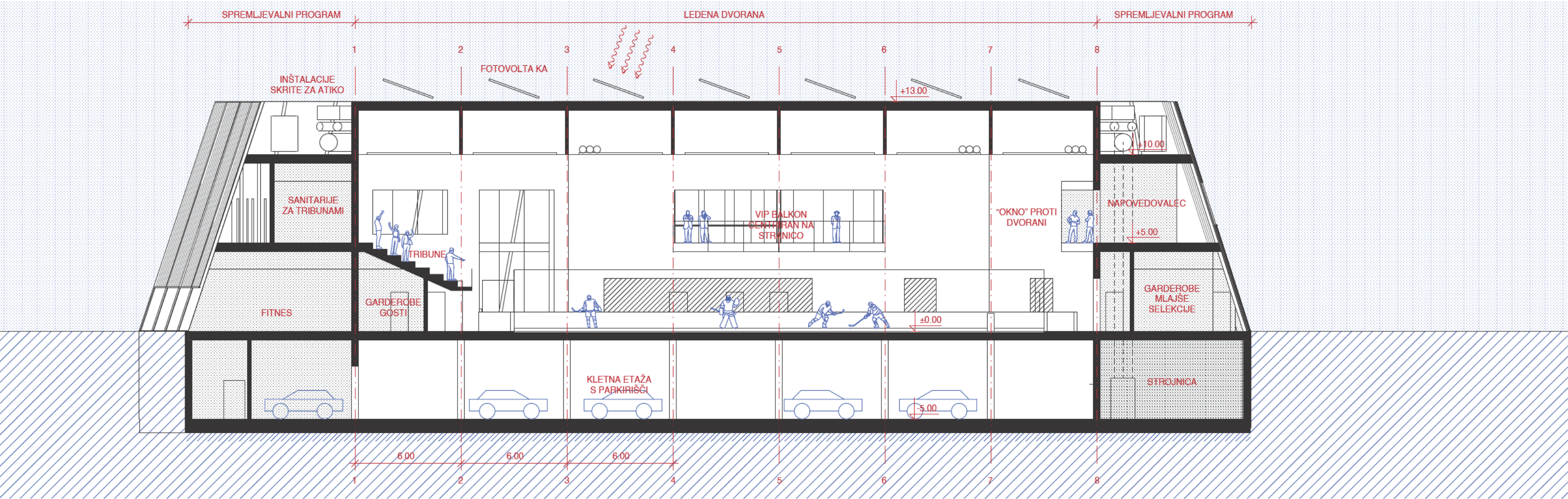
Prerez Y-Y M 1:200
