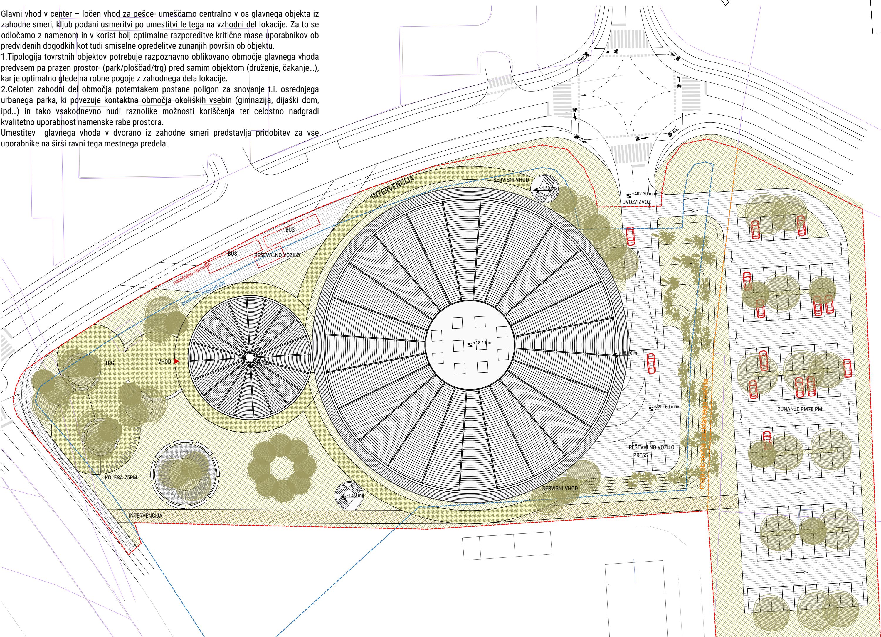
UREDITVENA SITUACIJA NATEČAJNEGA OBMOČJA (S PRIKAZOM TLORISA STREHE) TER ZUNANJO IN PROMETNO UREDITVIJO, M 1:500
