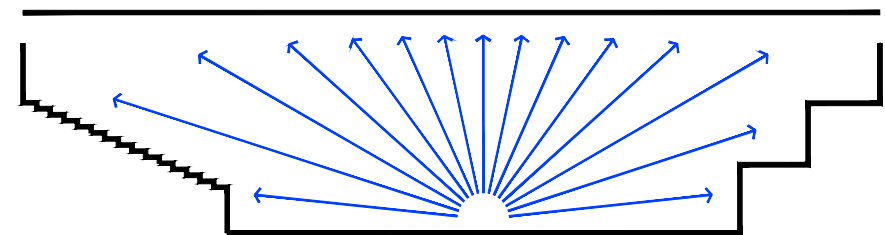
SCHEMA PREREZA DVORANE - AMBIENT AUDITORIJA
