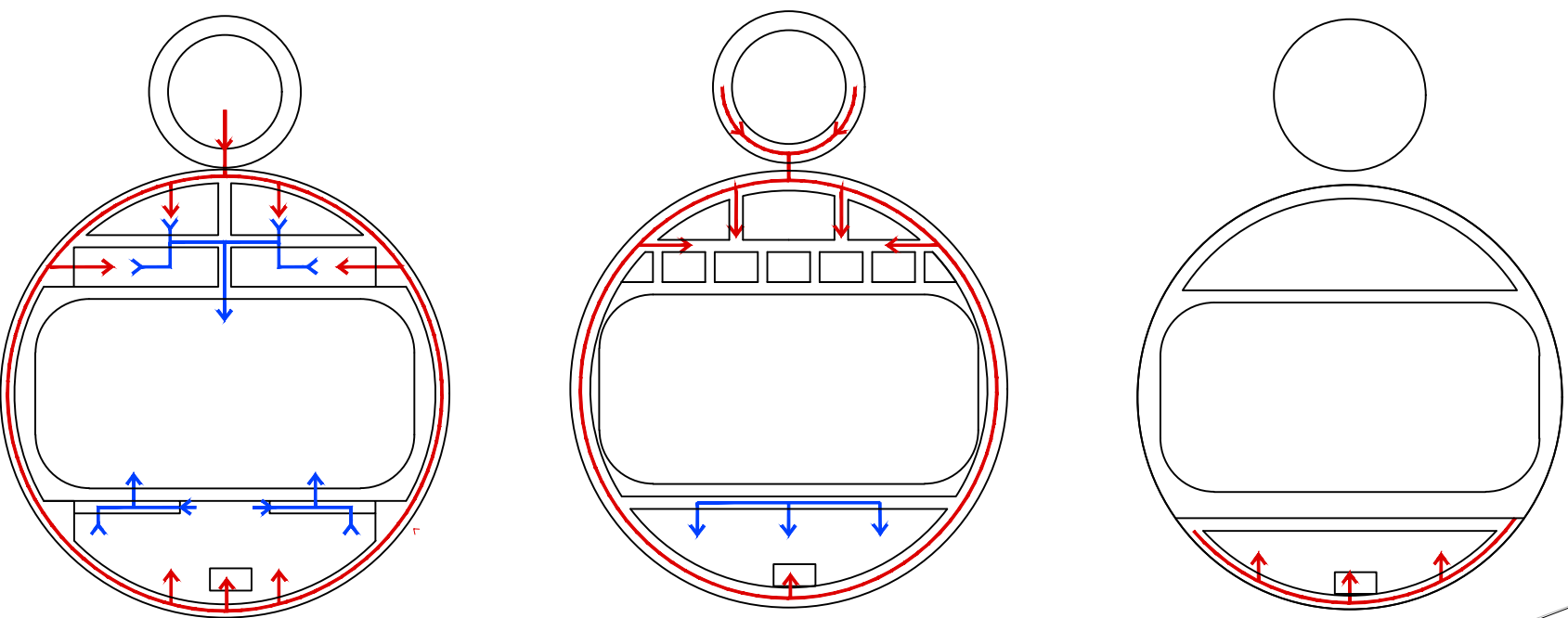
SHEMA ČISTE /UMAZANE POTI
