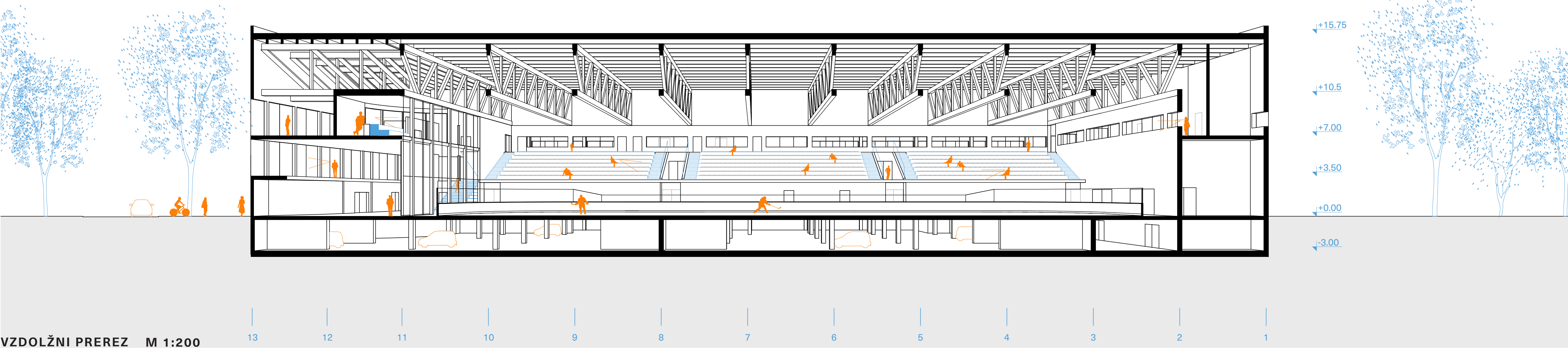
VZDOLŽNI PREREZ M 1:200
