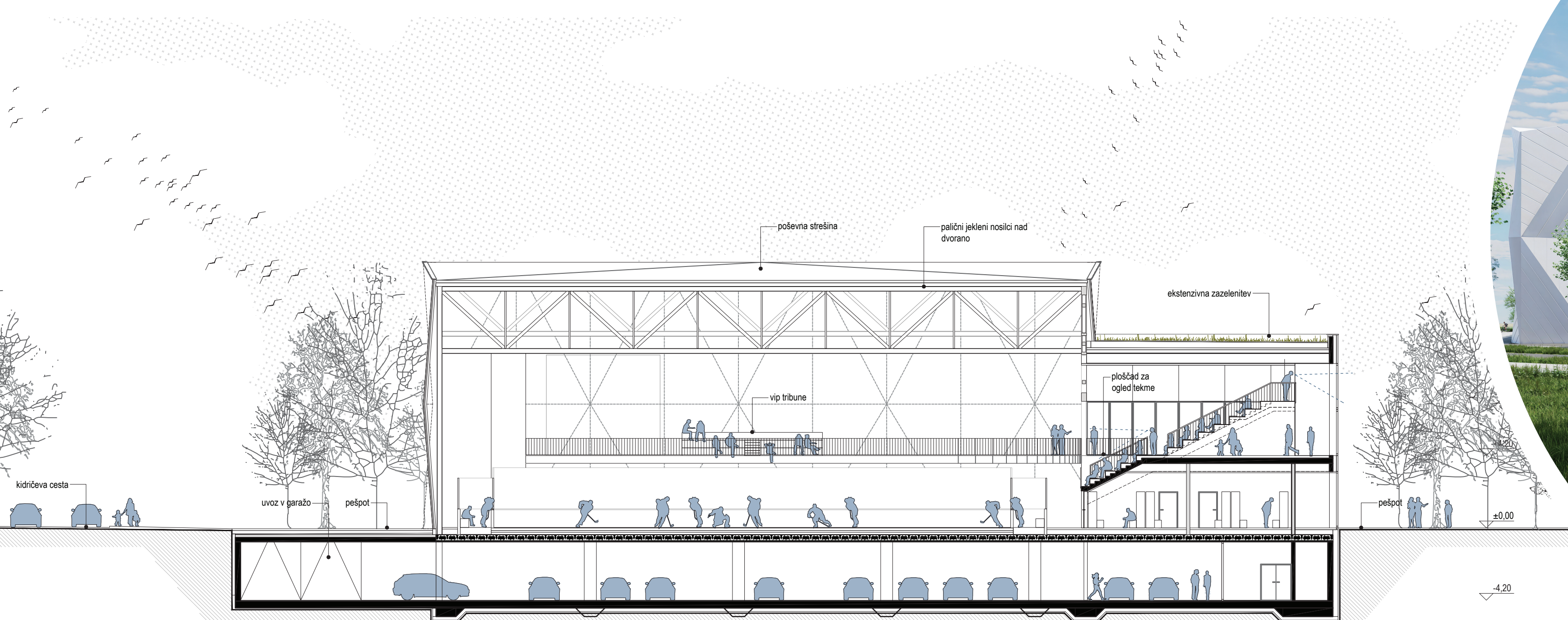
VZDOLŽNI PREREZ OBJEKTA IN TERENA M 1:200
