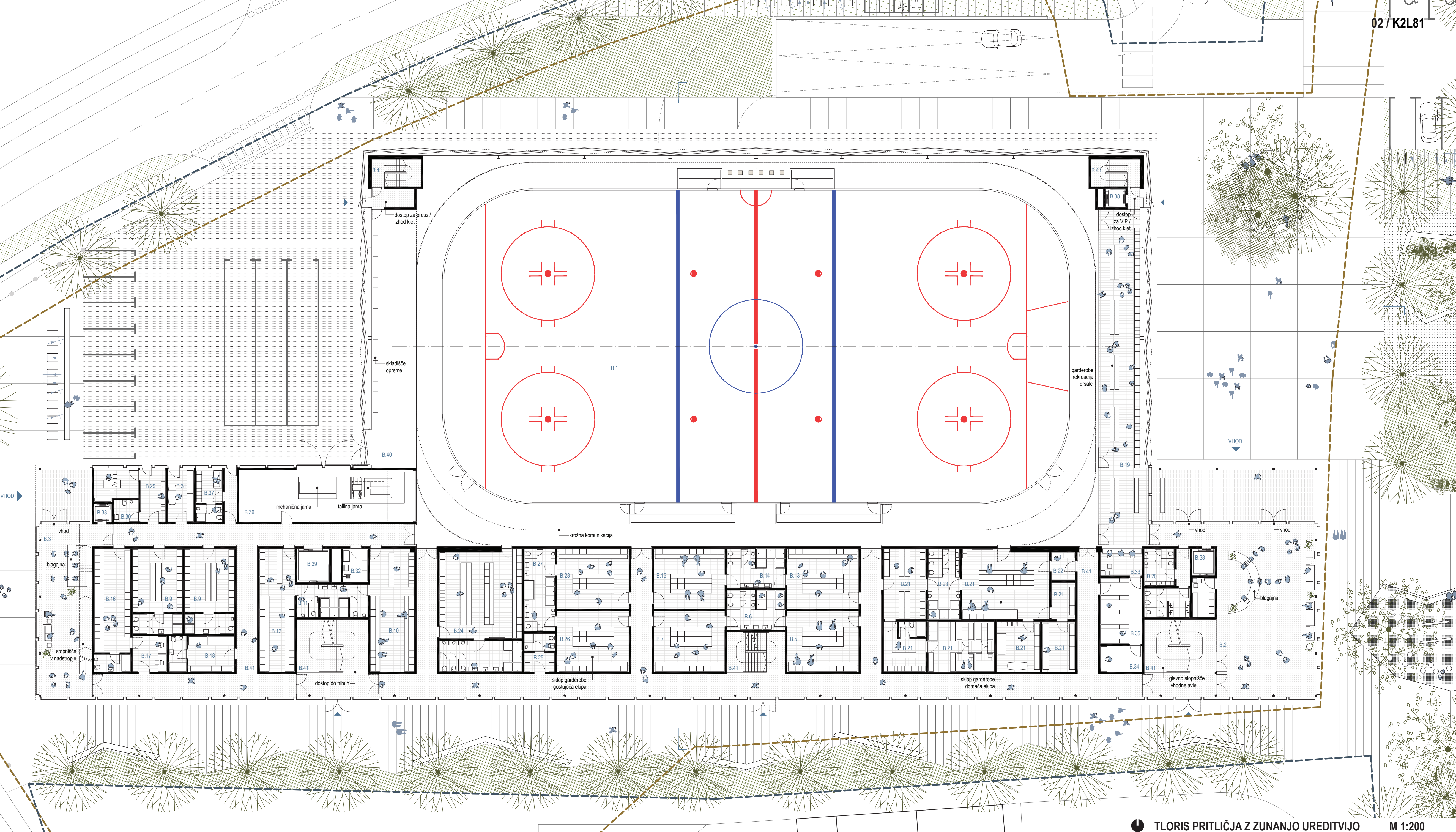
TLORIS PRITLIČJA Z ZUNANJO UREDITVIJO
