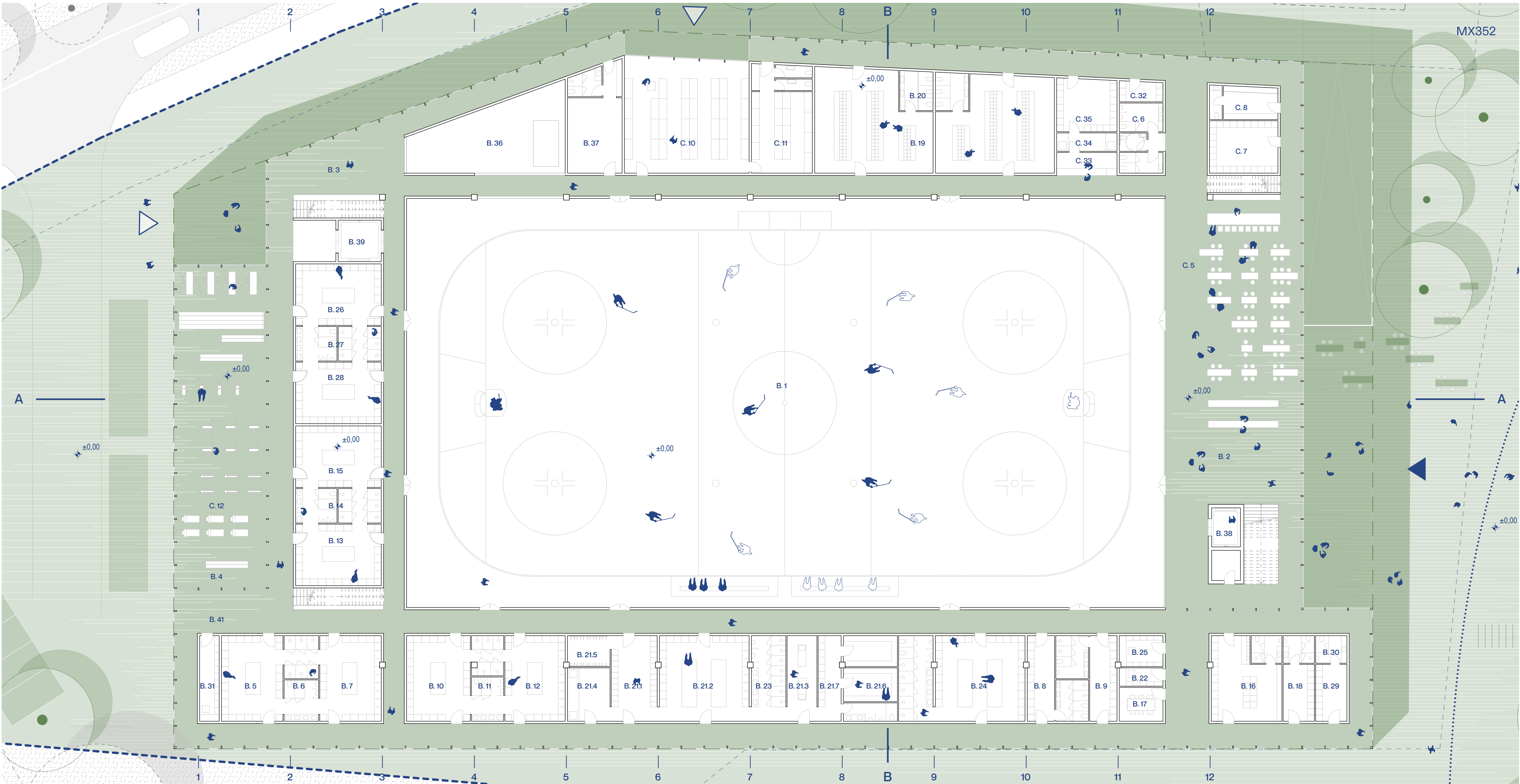
tloris pritličja M 1:200
