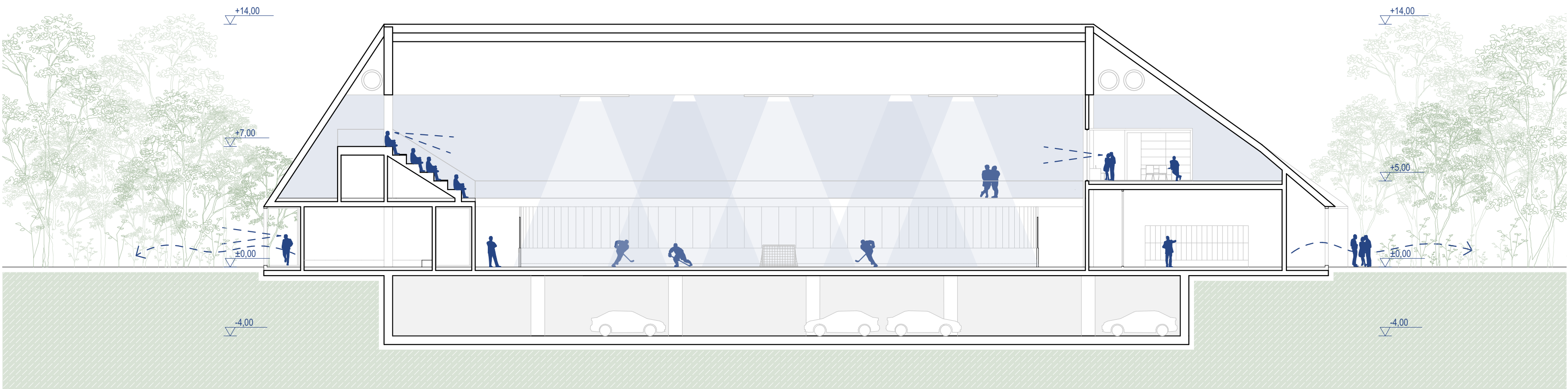
prečni prerez M 1:200
