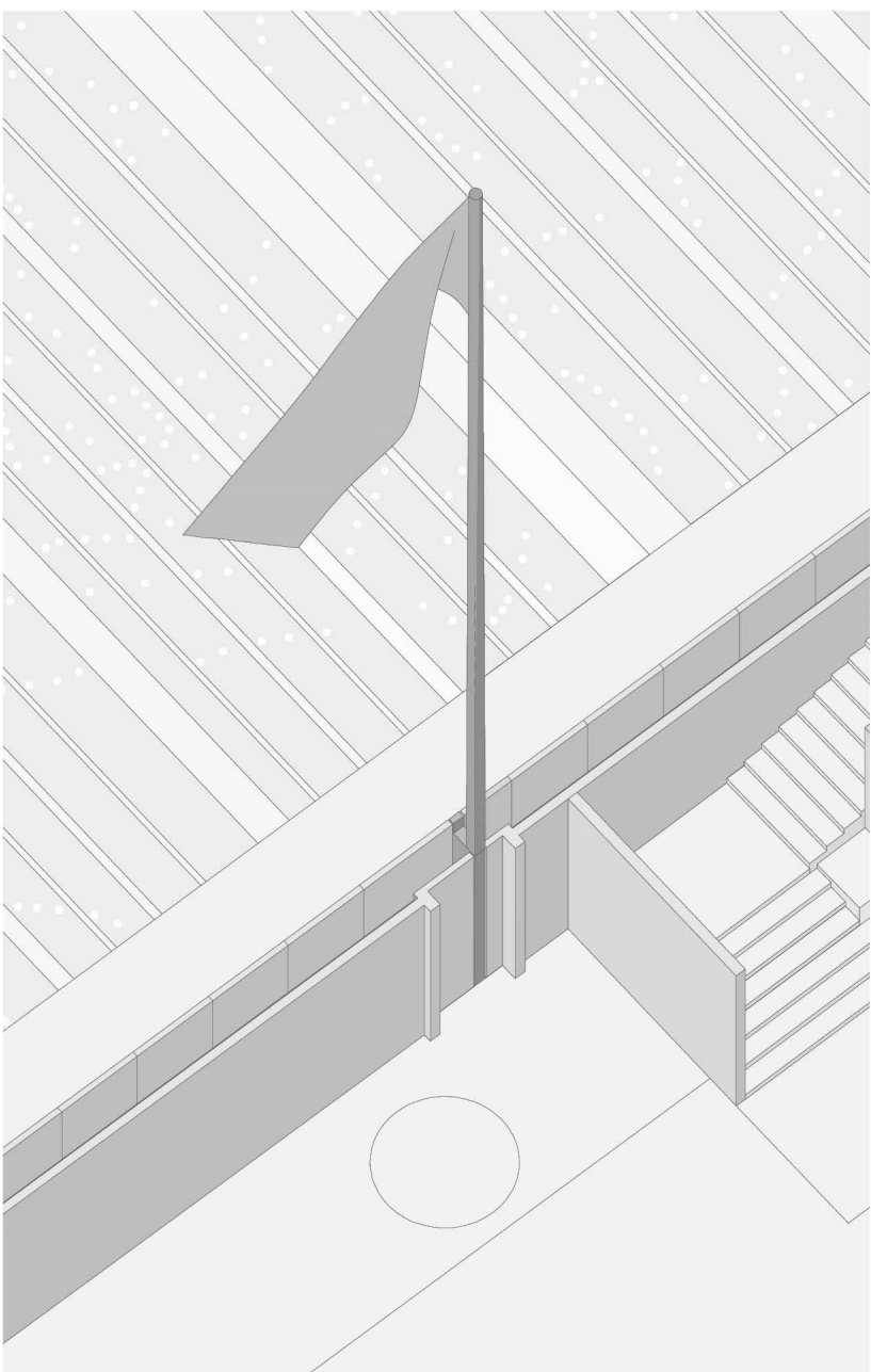
ZASTAVNI DROG JE UMEŠČEN V ZAREZO V ŠIRINI OBSTOJEČEGA BETONSKEGA KORITA
