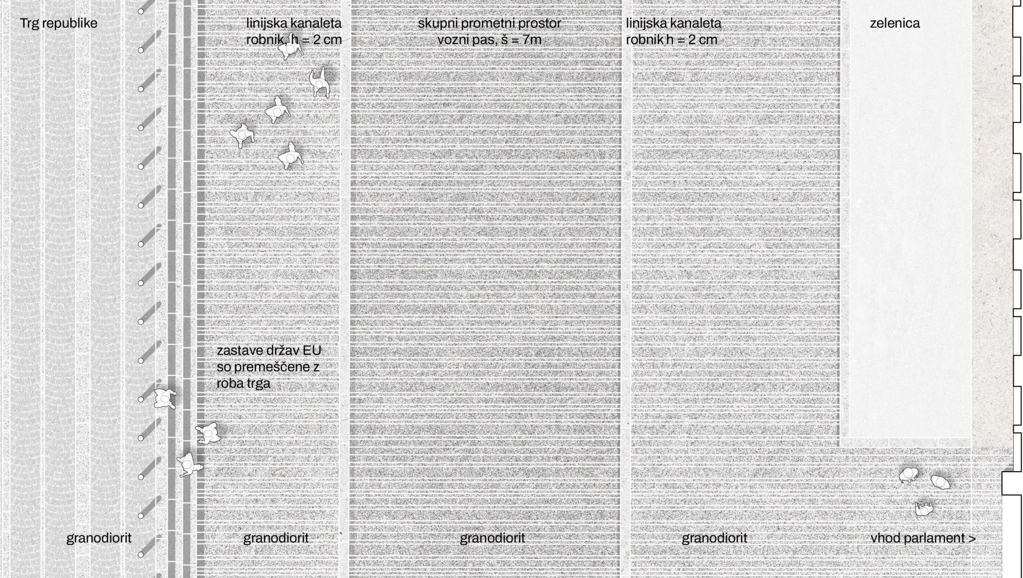
TLAKOVANJA ŠUBIČEVE ULICE, PRED PARLAMENTOM, M 1:100
