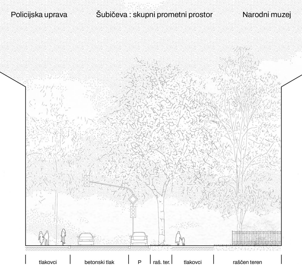
ULIČNI PROFIL ŠUBIČEVE ULICE, ZAHODNI DEL, M 1:250
